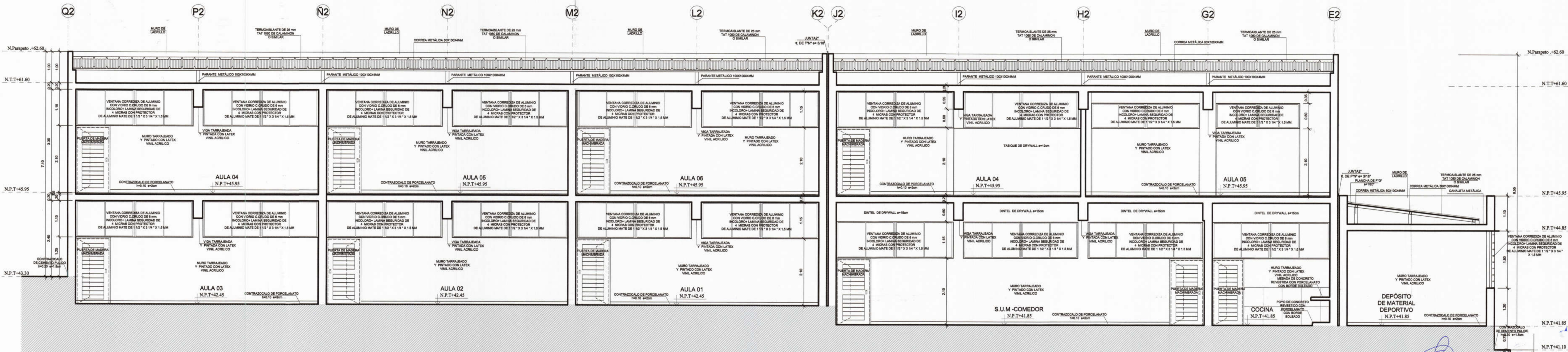
CORTE B-B 1/50
