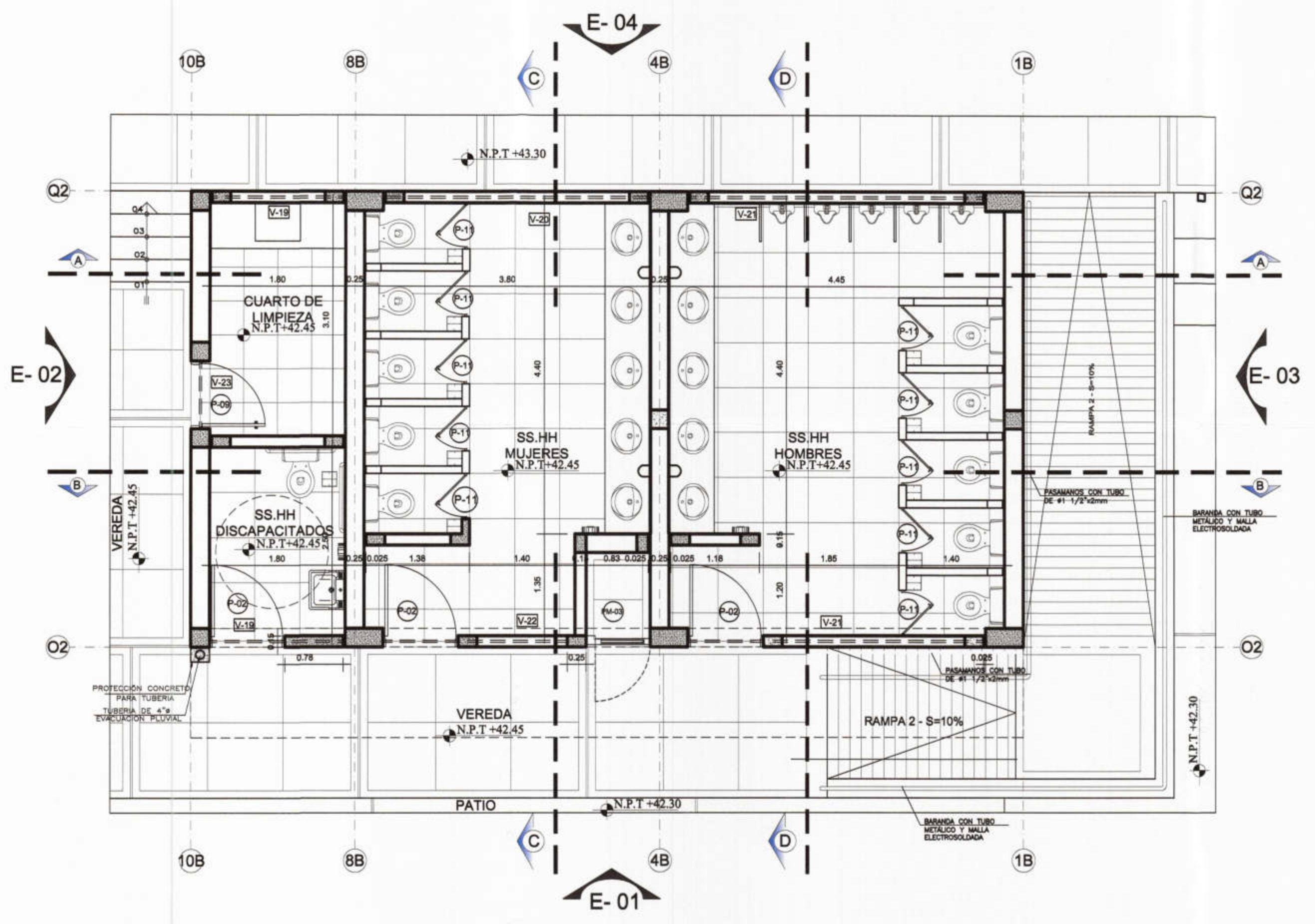
PRIMERA PLANTA 1/50
