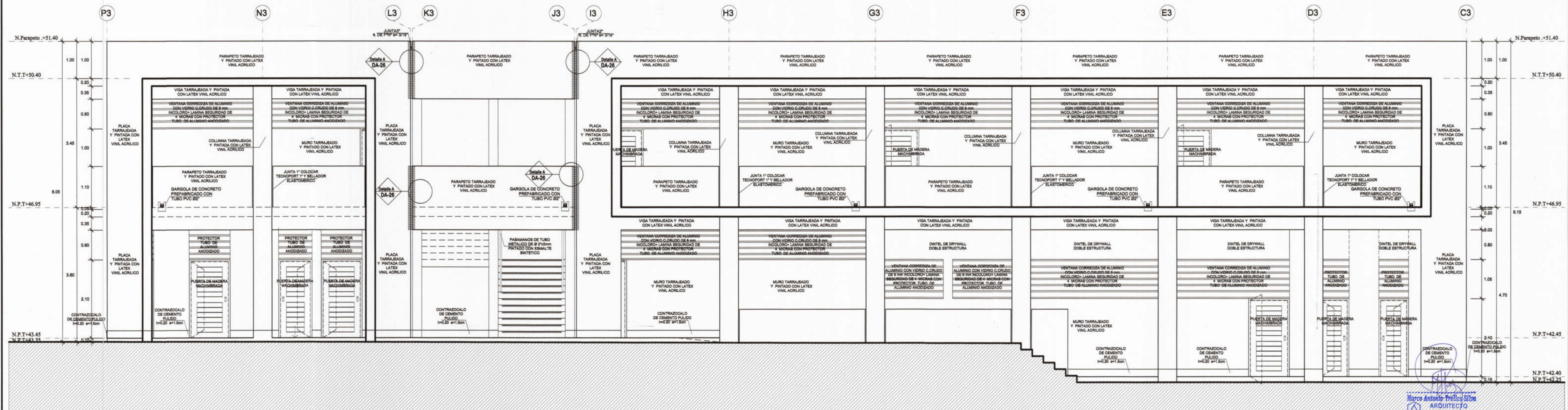
ELEVACION 02 1/50
