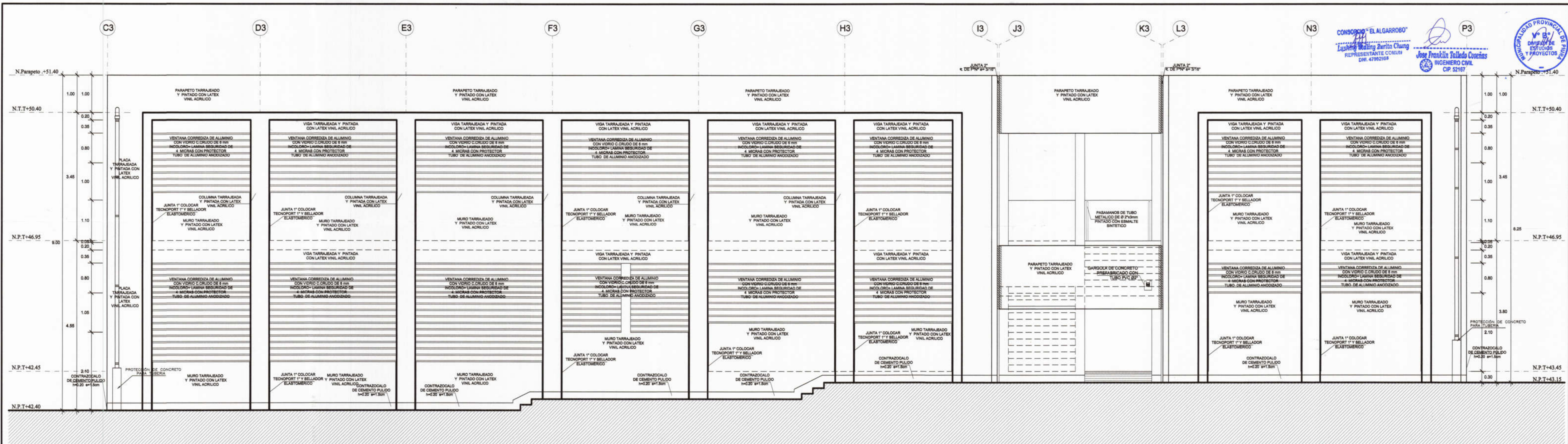
ELEVACION 01 1/50
