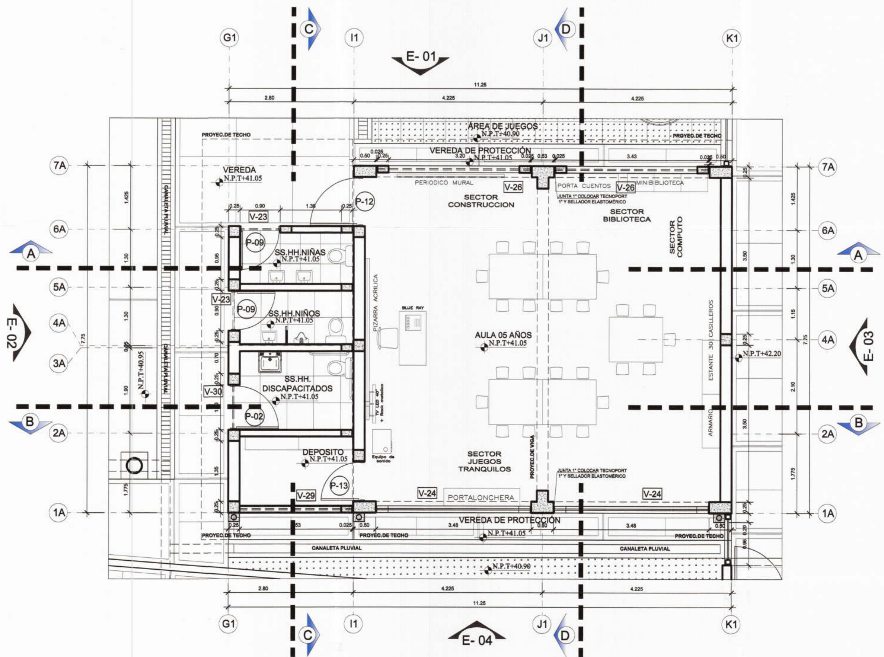
PRIMERA PLANTA 1/50
