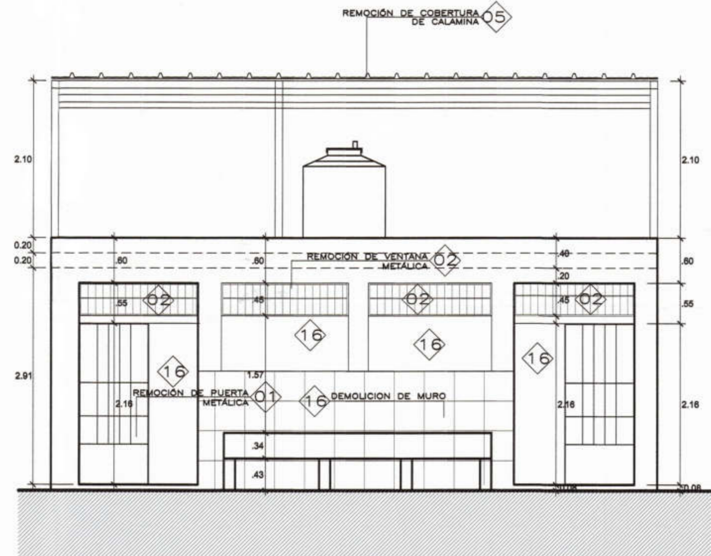
ELEVACION 01 1/50
