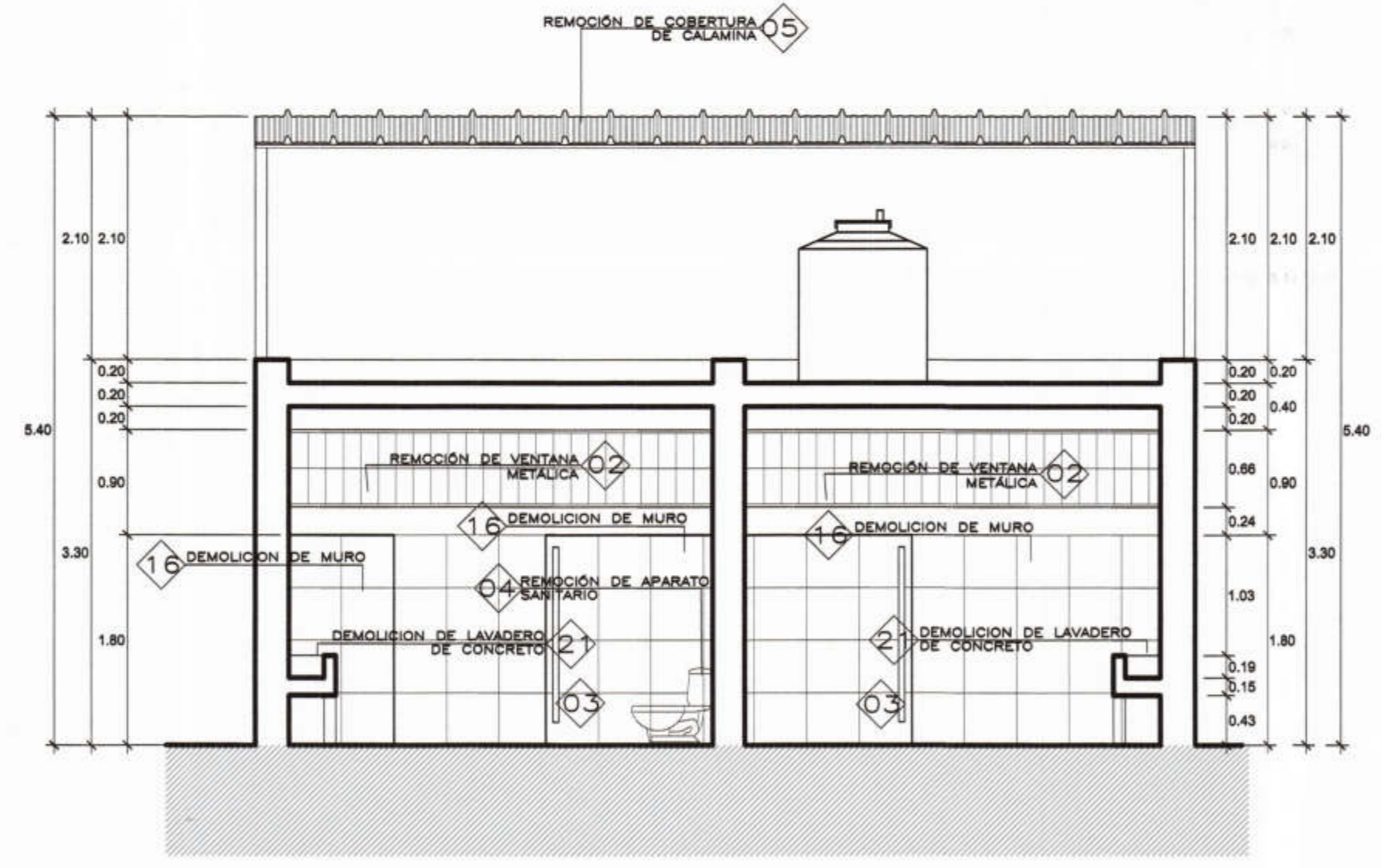
CORTE B-B 1/50
