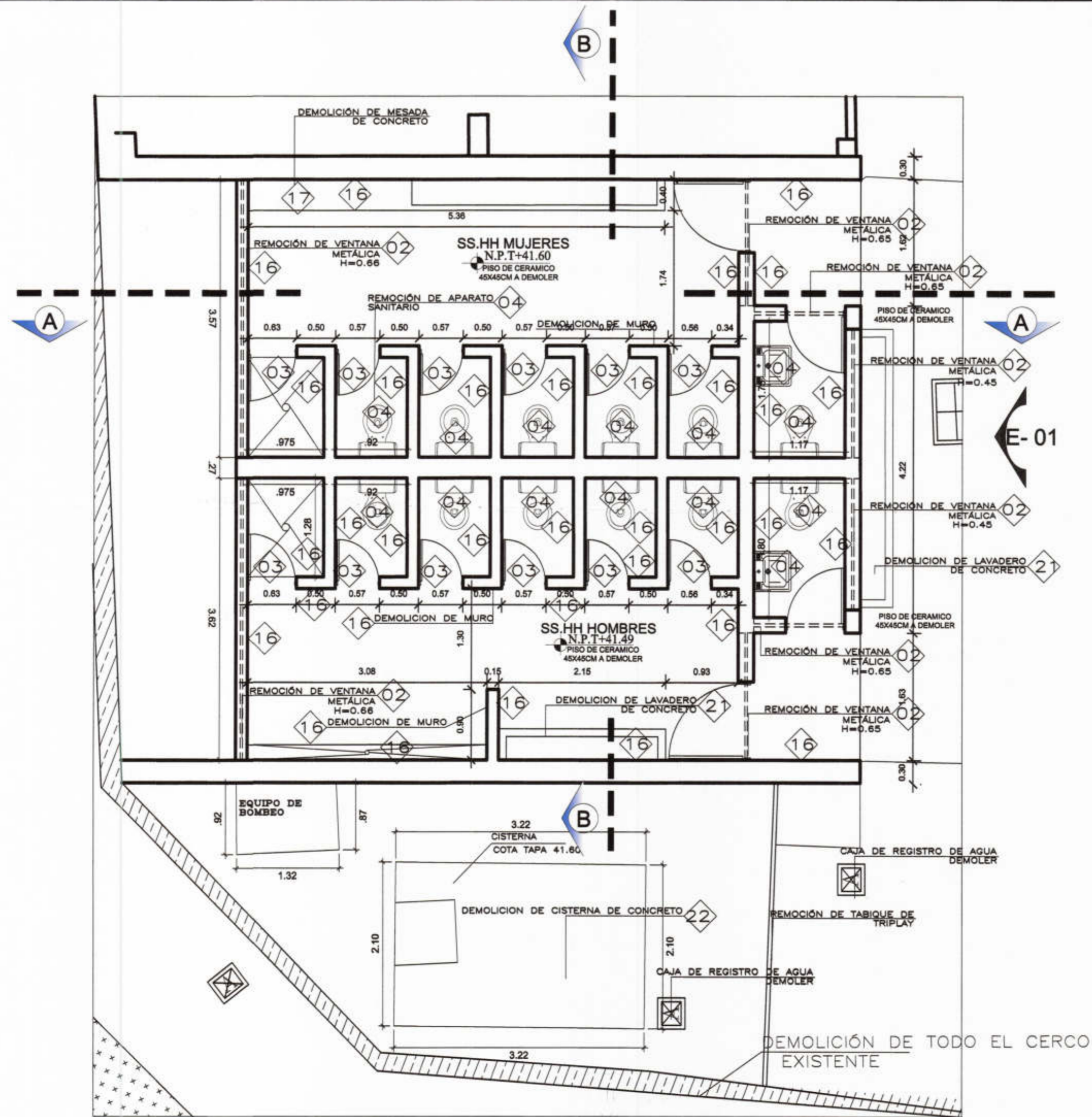
PRIMERA PLANTA-BLOQUE 01 A DEMOLER 1/50
