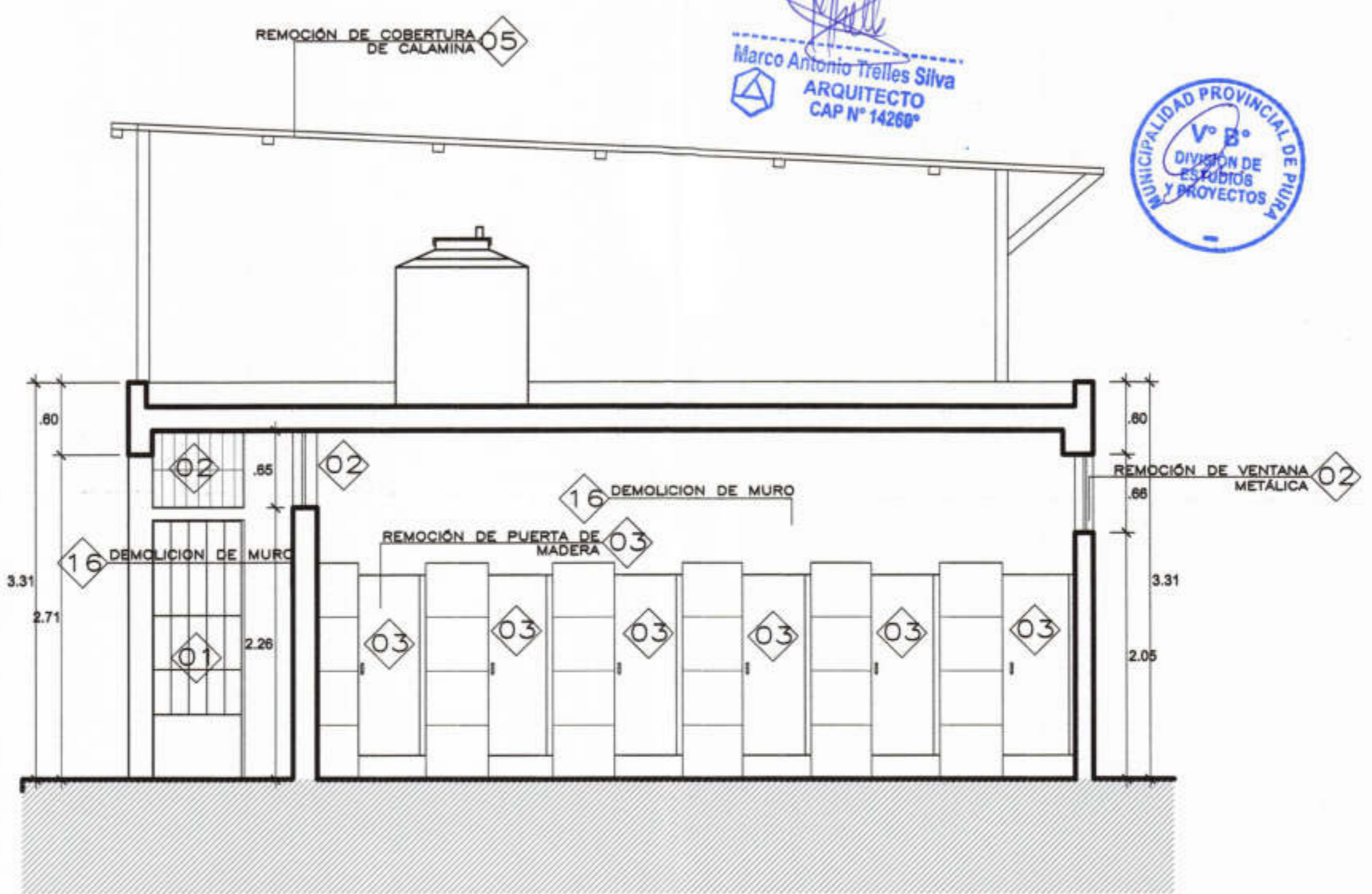
CORTE A-A 1/50
