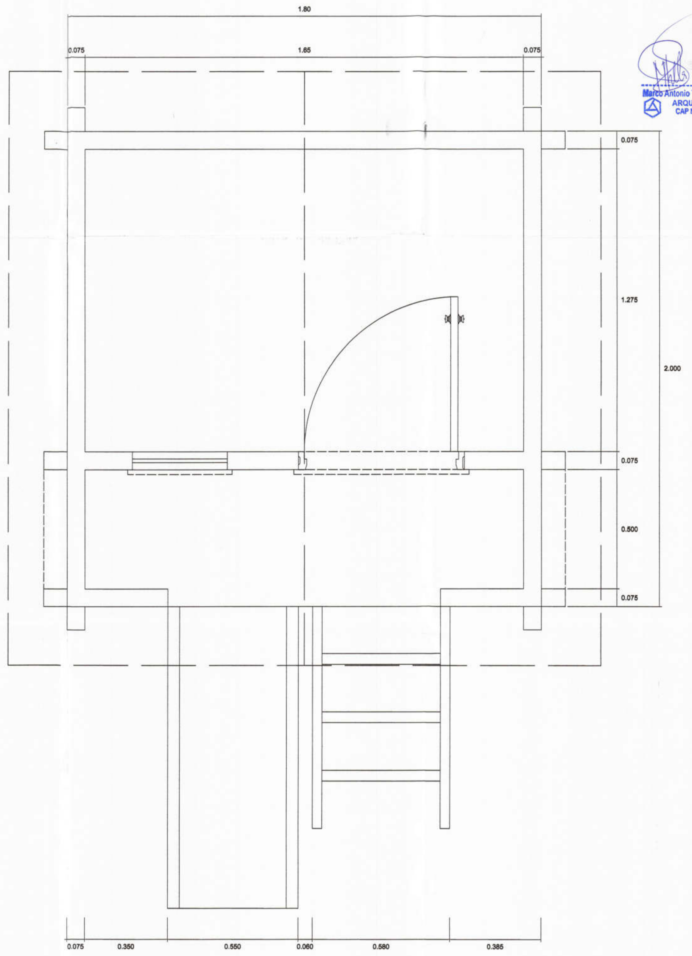
CASITA DE MADERA ESC: 1/10 CANTIDAD 02
