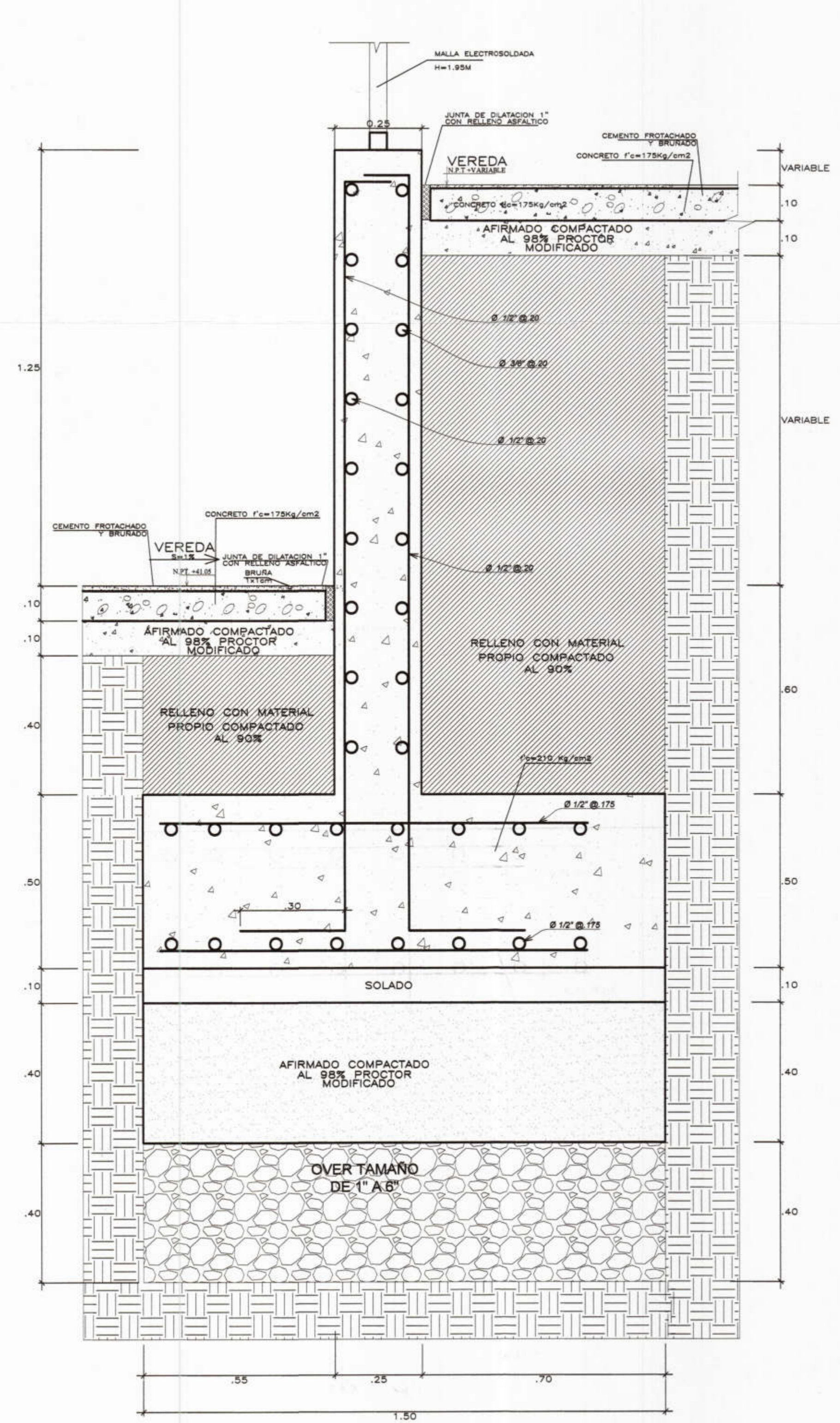
17 DETALLE VEREDA-MURO DE CONTENCIÓN-VEREDA Esc.: 1/10
