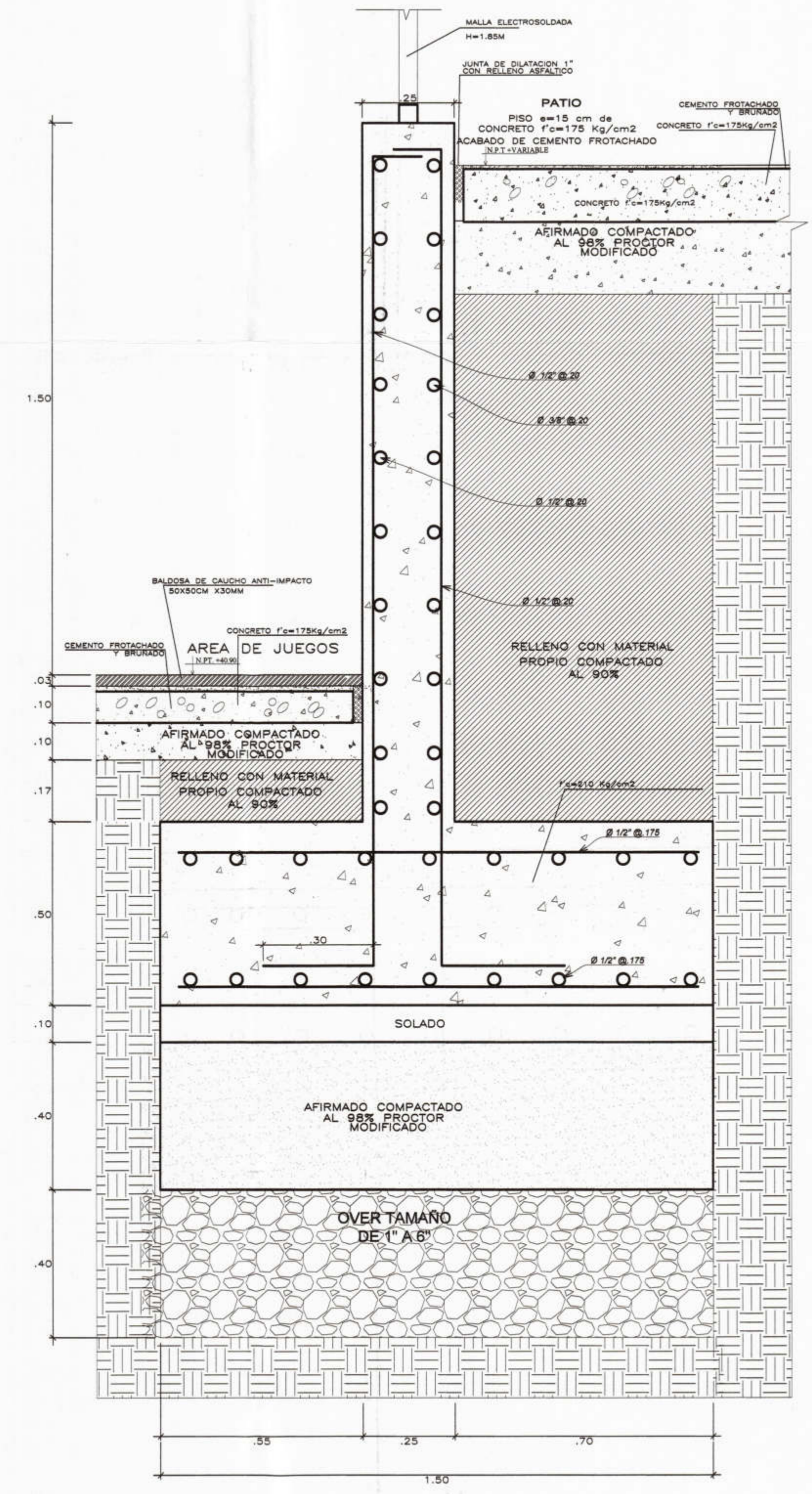
18 ÁREA DE JUEGOS-MURO DE CONTENCIÓN-PATIO Esc.: 1/10
