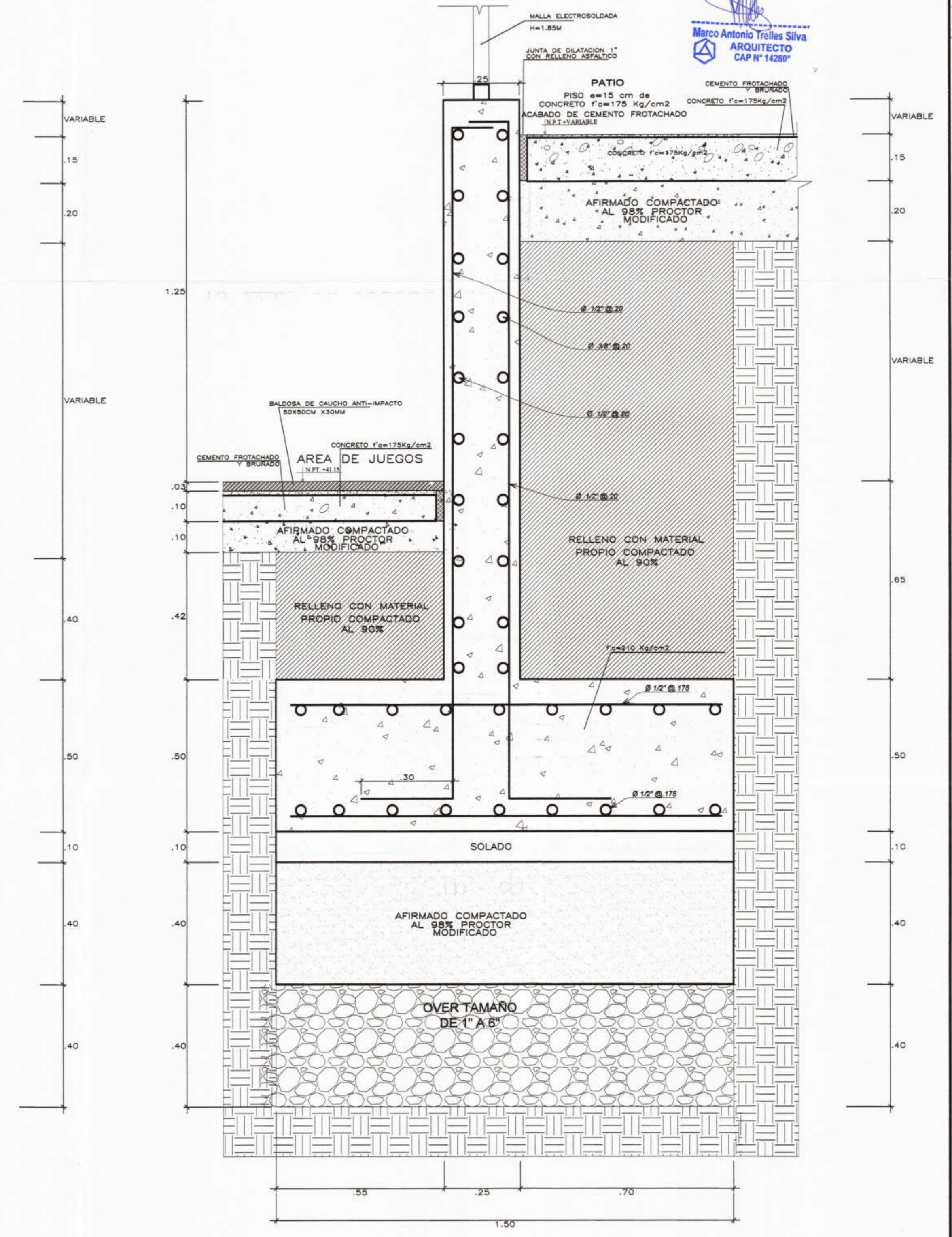
19 ÁREA DE JUEGOS-MURO DE CONTENCIÓN-PATIO Esc.: 1/10
