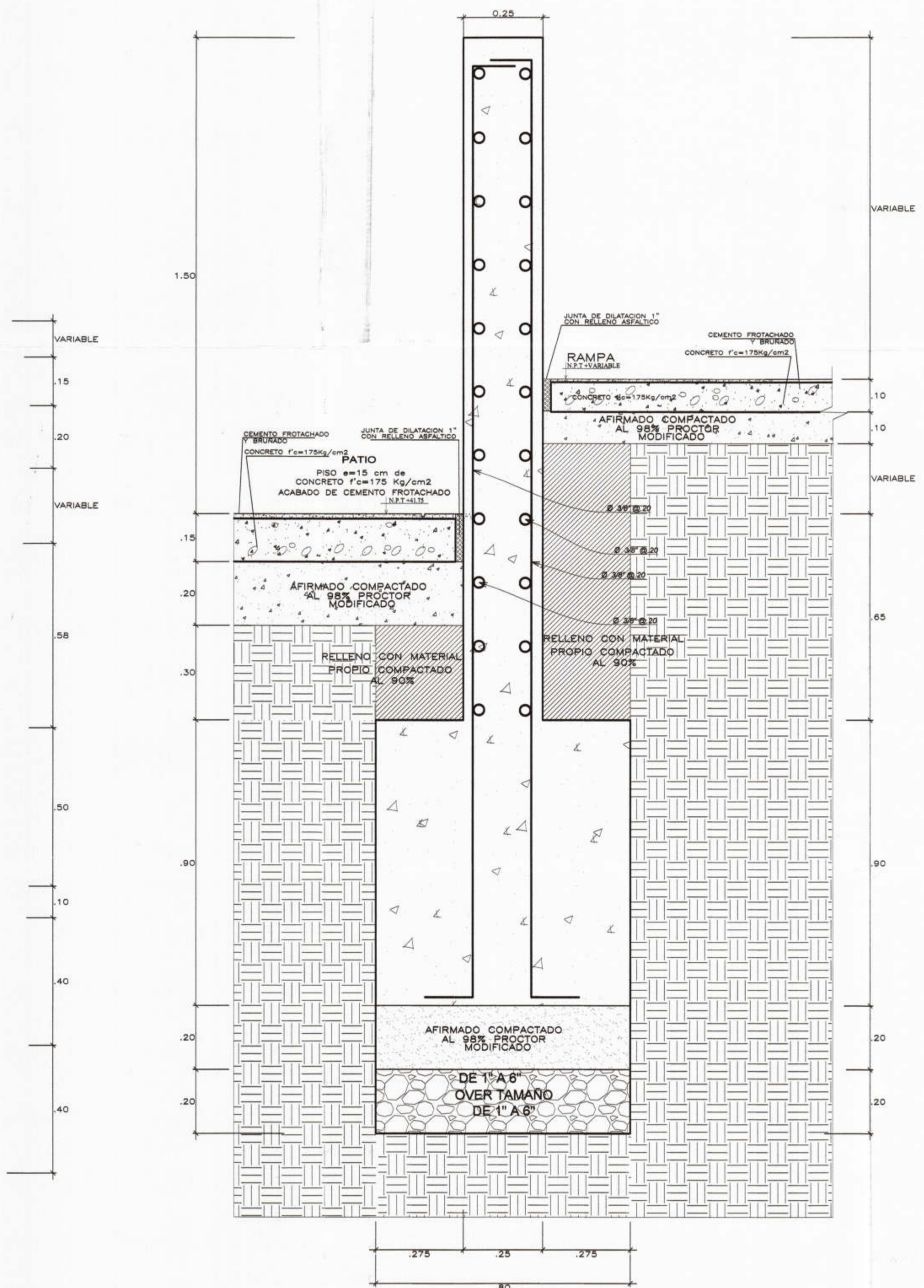
21 DETALLE PATIO-MURO DE CONTENCIÓN-RAMPA ESC.: 1/10
