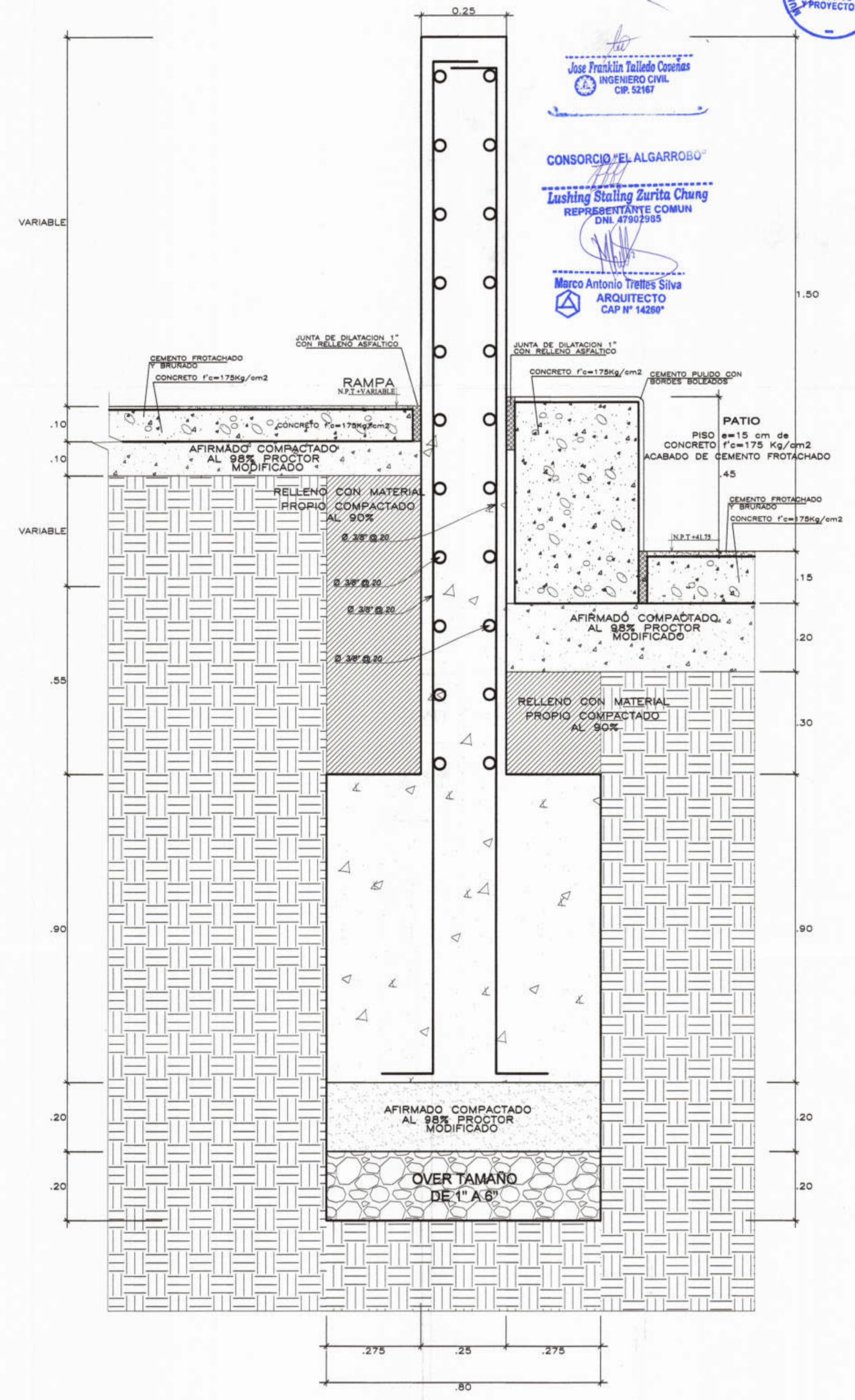
22 DETALLE RAMPA-MURO DE CONTENCIÓN-BANCA DE CONCRETO ESC.: 1/10
