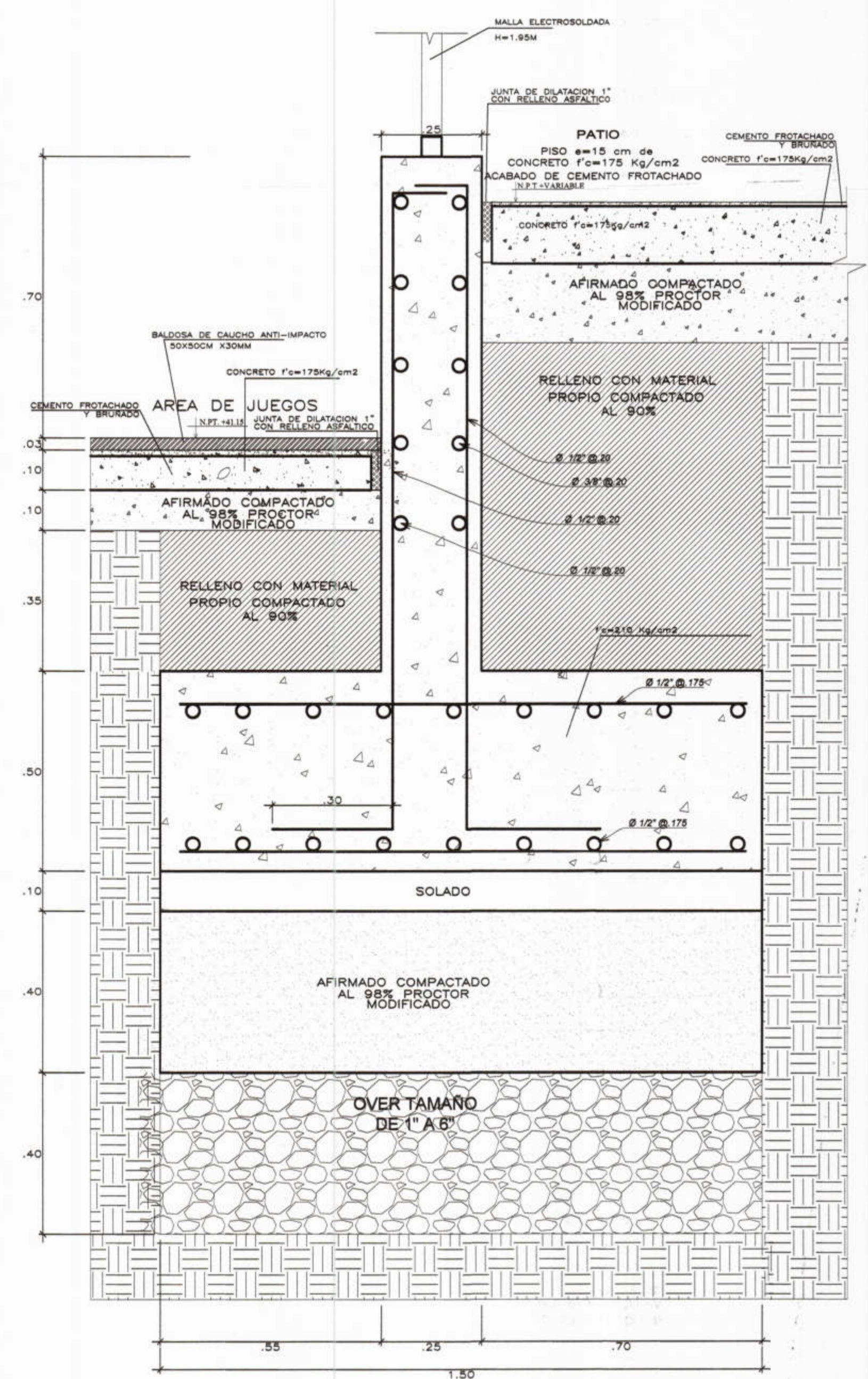
20 AREA DE JUEGOS-MURO DE CONTENCIÓN-PATIO ESC.: 1/10
