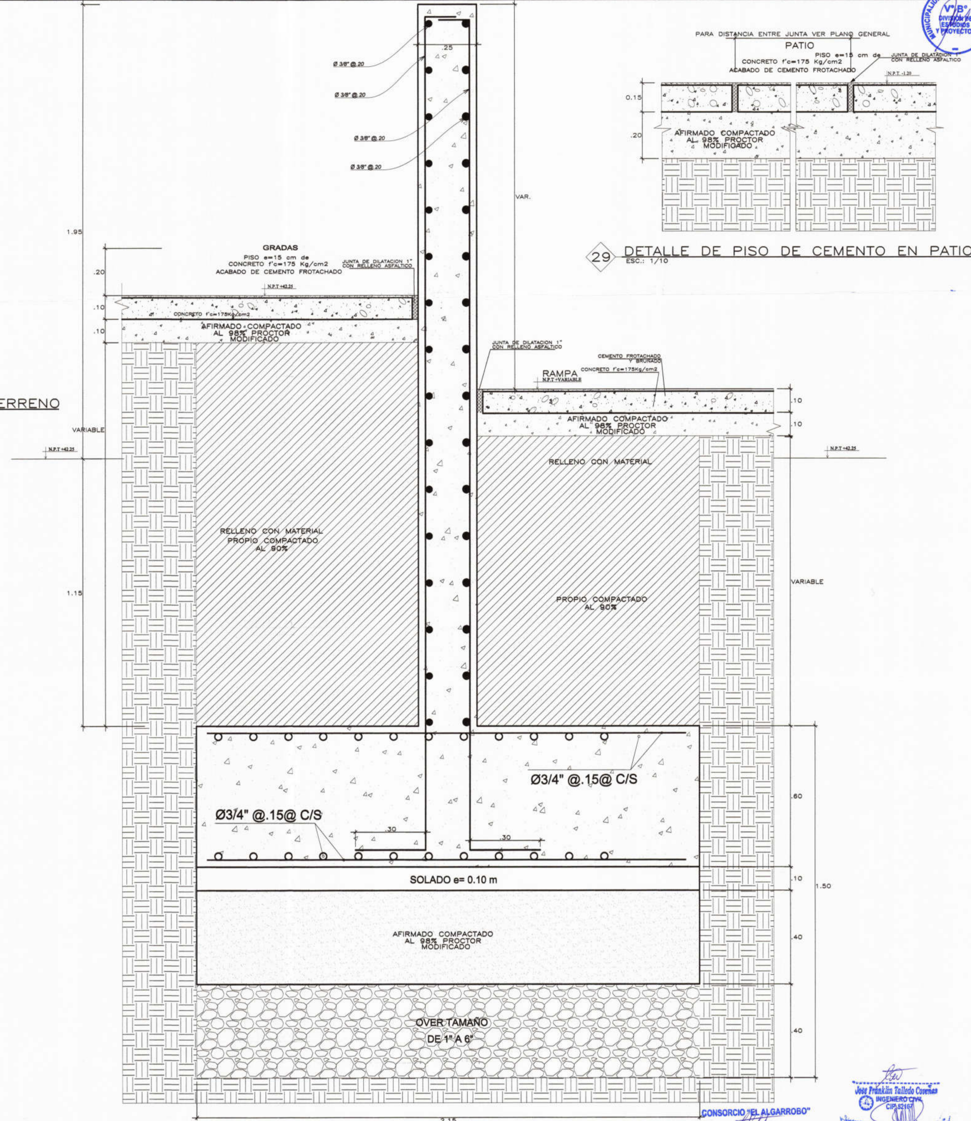
27 DETALLE PATIO-MURO DE CONTENCIÓN-RAMPA ESC.: 1/10
