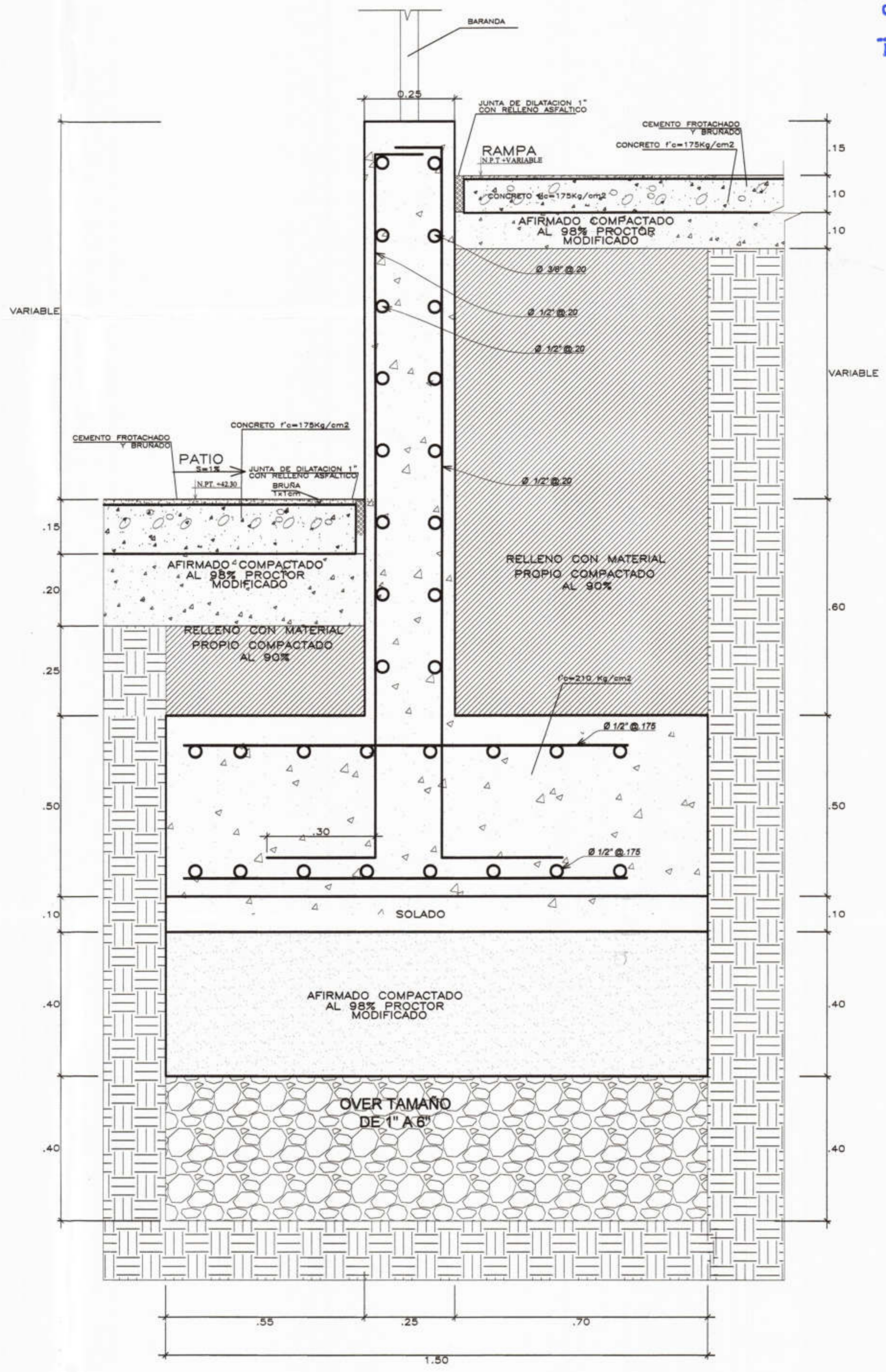
37 DETALLE PATIO-MURO DE CONTENCIÓN-RAMPA ESC.: 1/10
