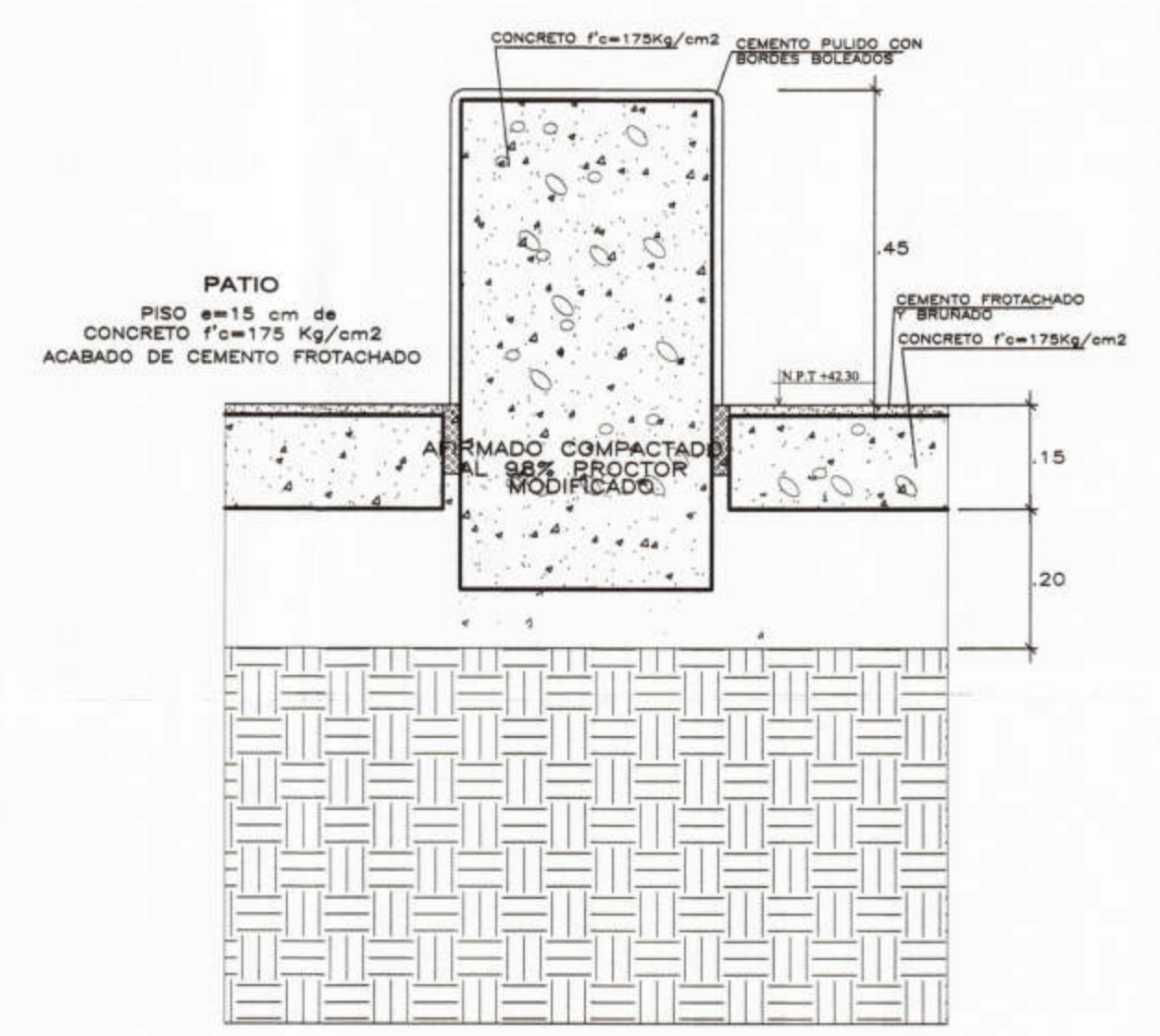
38 DETALLE POYO DE CONCRETO ESC.: 1/10
