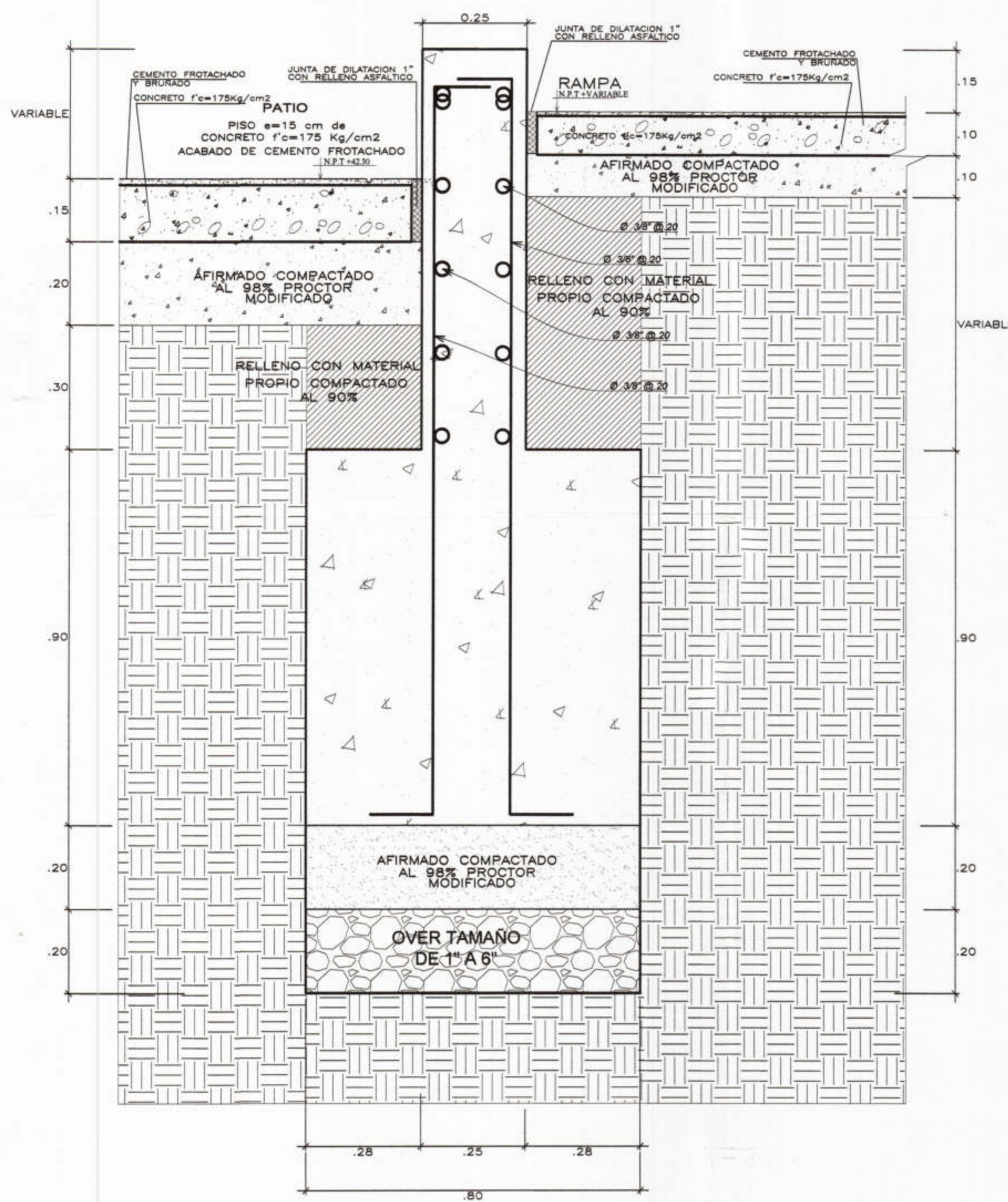
36 DETALLE PATIO-MURO DE CONTENCIÓN-RAMPA ESC.: 1/10
