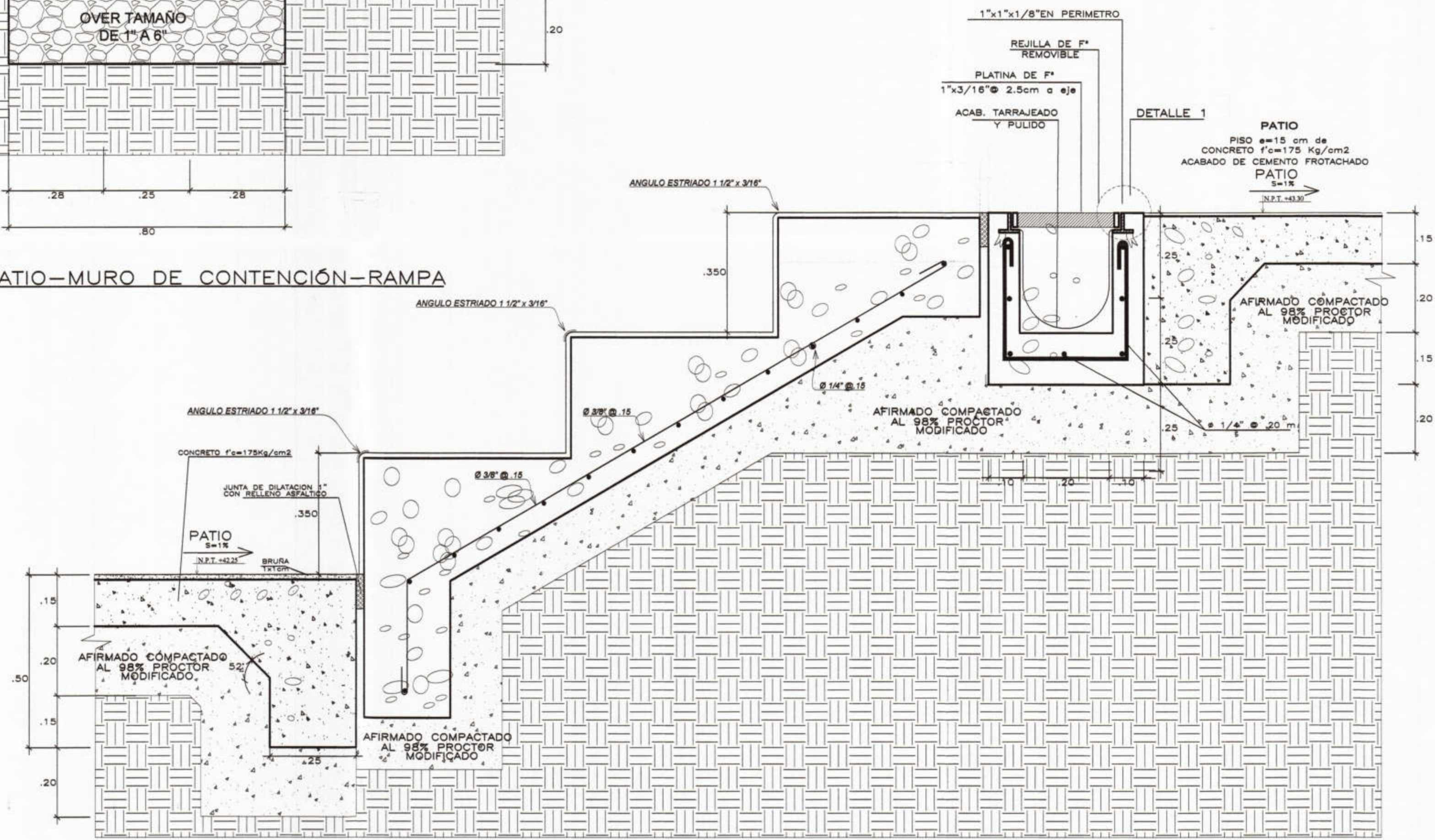
35 DETALLE DE PATIO-GRADAS-PATIO ESC.: 1/10
