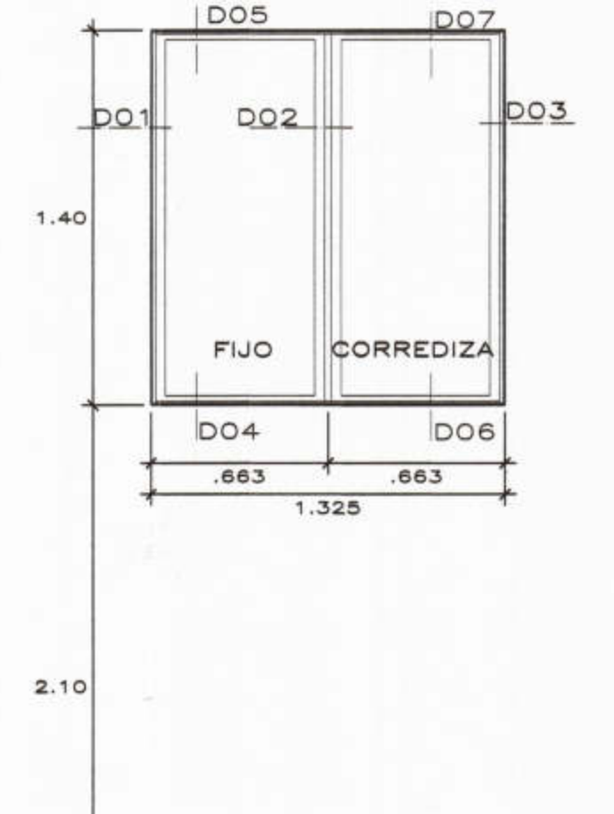
V-04 esc: 1/25 11 unidades VENTANA DE ALUMINIO SERIE 25 (MIYASATO O SIMILAR.) VIDRIO C. CRUDO DE 6 mm INCOLORO + LAMINA SEGURIDAD DE 4 MICRAS
