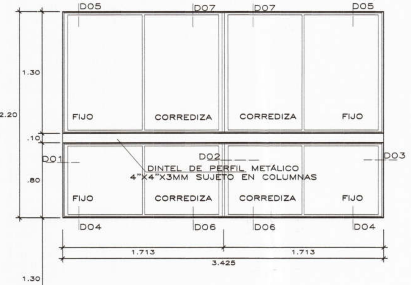
V-02 esc: 1/25 08 unidades VENTANA DE ALUMINIO SERIE 25 (MIYASATO O SIMILAR.) VIDRIO C. CRUDO DE 6 mm INCOLORO + LAMINA SEGURIDAD DE 4 MICRAS
