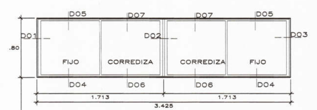
V-08 esc: 1/25 01 unidades VENTANA DE ALUMINIO SERIE 25 (MIYASATO O SIMILAR.) VIDRIO C. CRUDO DE 6 mm INCOLORO + LAMINA SEGURIDAD DE 4 MICRAS
