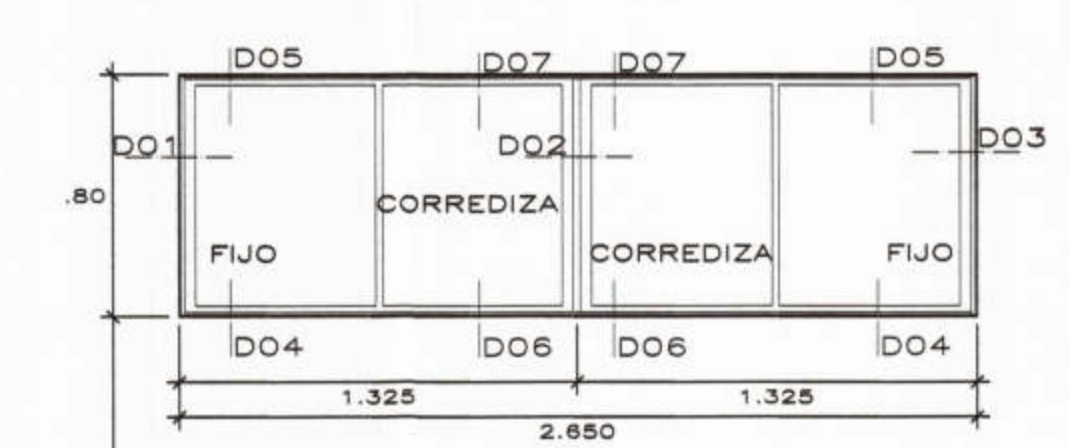
V-07 esc: 1/25 01 unidades VENTANA DE ALUMINIO SERIE 25 (MIYASATO O SIMILAR.) VIDRIO C. CRUDO DE 6 mm INCOLORO + LAMINA SEGURIDAD DE 4 MICRAS
