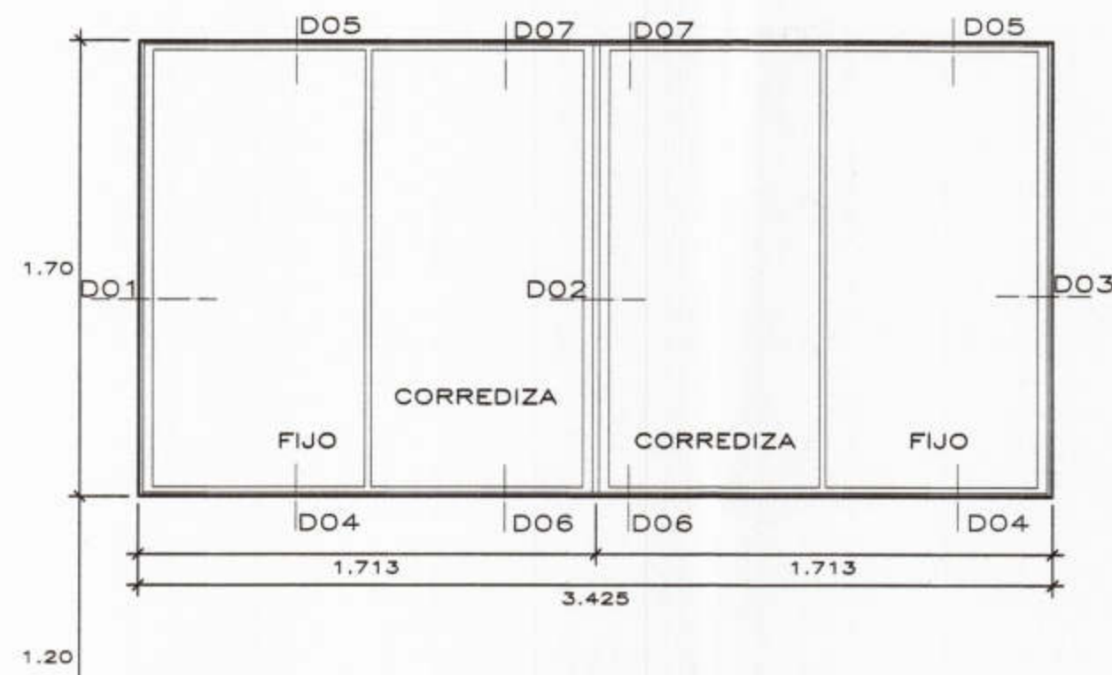
V-01 esc: 1/25 14 unidades VENTANA DE ALUMINIO SERIE 25 (MIYASATO O SIMILAR.) VIDRIO C. CRUDO DE 6 mm INCOLORO + LAMINA SEGURIDAD DE 4 MICRAS
