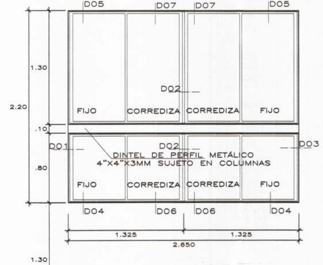
V-01 esc: 1/25 14 unidades VENTANA DE ALUMINIO SERIE 25 (MIYASATO O SIMILAR.) VIDRIO C. CRUDO DE 6 mm INCOLORO + LAMINA SEGURIDAD DE 4 MICRAS
