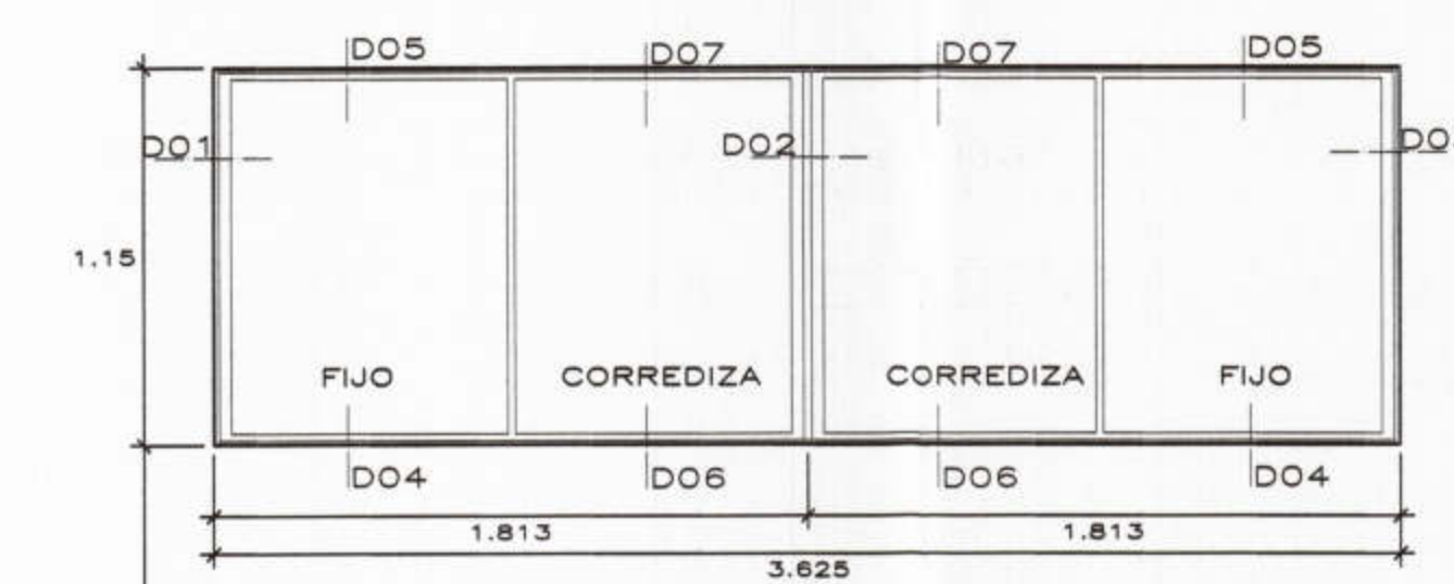
V-05 esc: 1/25 01 unidades VENTANA DE ALUMINIO SERIE 25 (MIYASATO O SIMILAR.) VIDRIO C. CRUDO DE 6 mm INCOLORO + LAMINA SEGURIDAD DE 4 MICRAS
