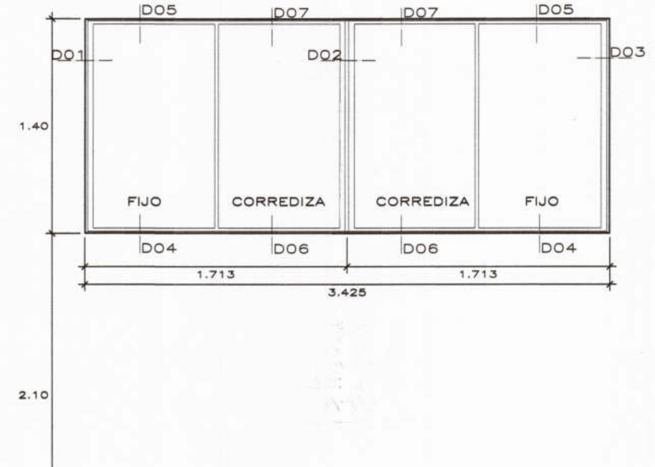
V-03 esc: 1/25 10 unidades VENTANA DE ALUMINIO SERIE 25 (MIYASATO O SIMILAR.) VIDRIO C. CRUDO DE 6 mm INCOLORO + LAMINA SEGURIDAD DE 4 MICRAS
