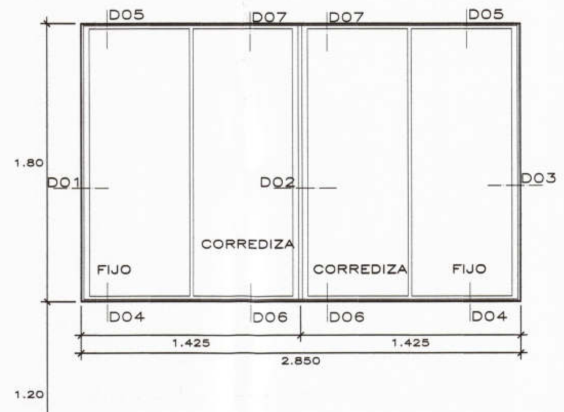
V-10 esc: 1/25 01 unidades VENTANA DE ALUMINIO SERIE 25 (MIYASATO O SIMILAR.) VIDRIO C. CRUDO DE 6 mm INCOLORO + LAMINA SEGURIDAD DE 4 MICRAS
