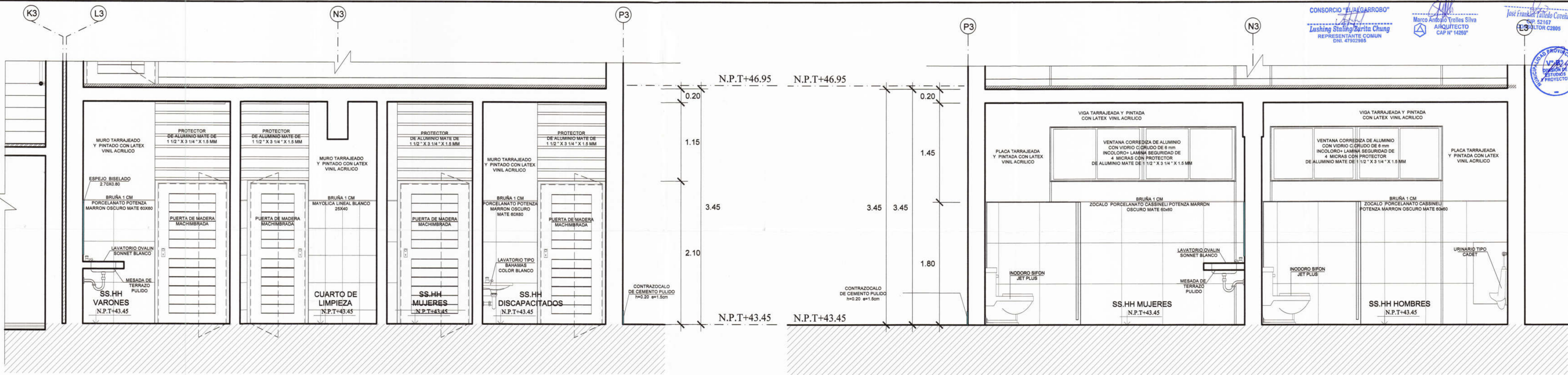
CORTE A-A 1/25
