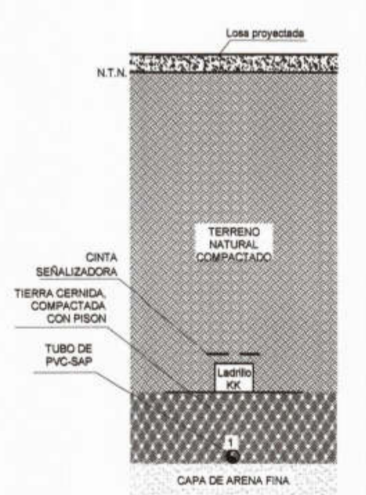
SECCION H-H
