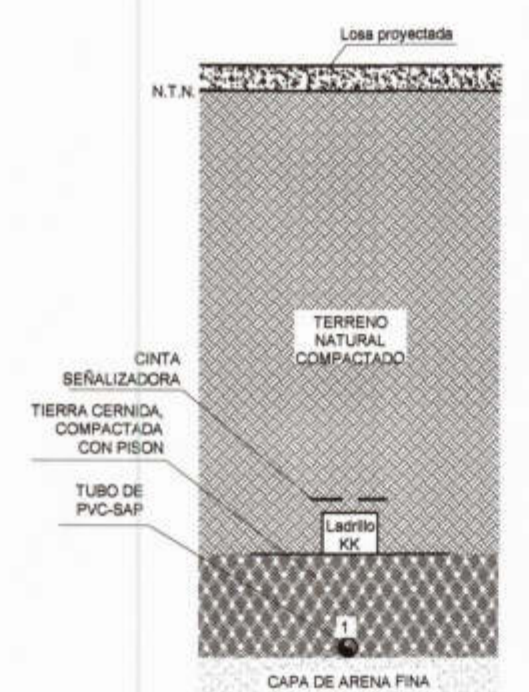
SECCION A-A
