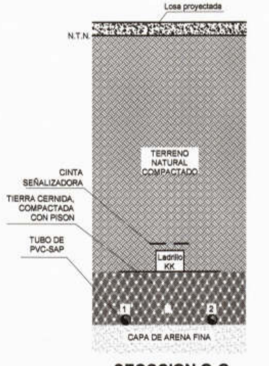
SECCION G-G
