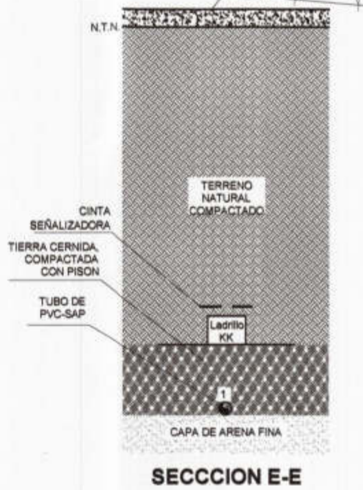
SECCION E-E
