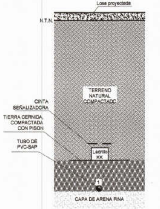
SECCION B-B
