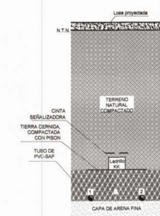
SECCION C-C
