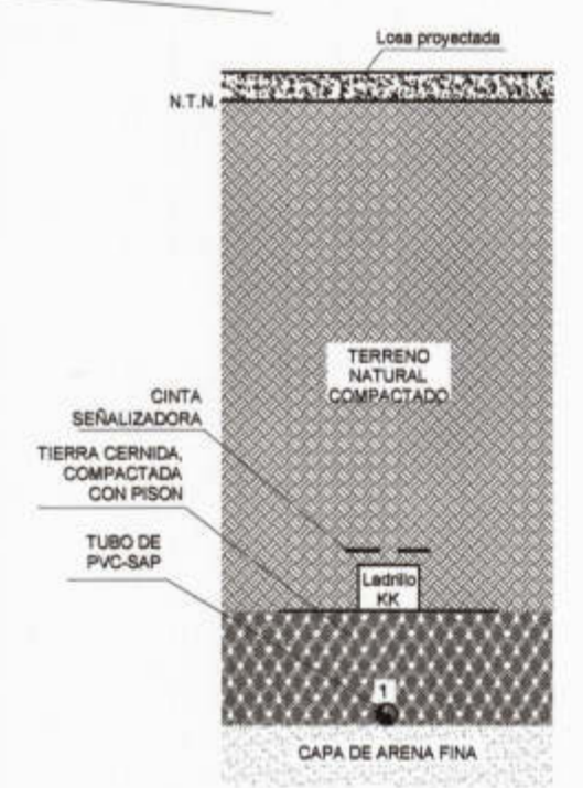
SECCION F-F
