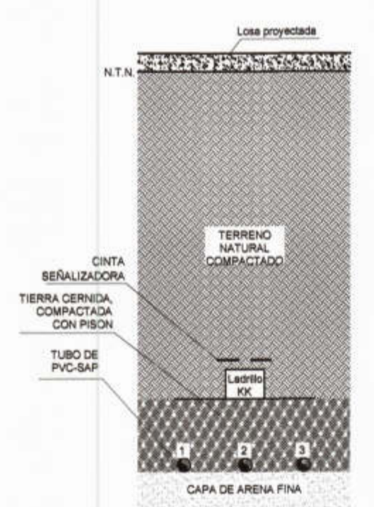
SECCION D-D
