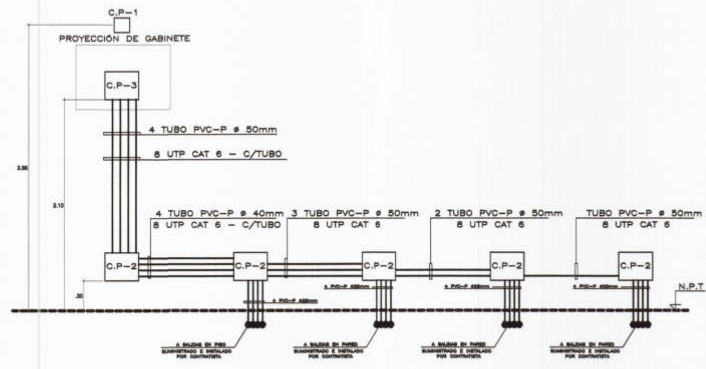
ESQUEMA DE CAJAS DE PASO/TUBOS PVC CABLEADO ESTRUCTURADO
