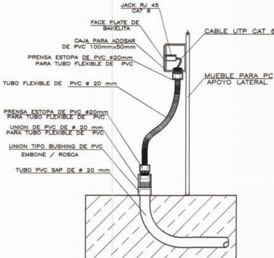
DETALLE DE SALIDAS DE DATA EN PISO
