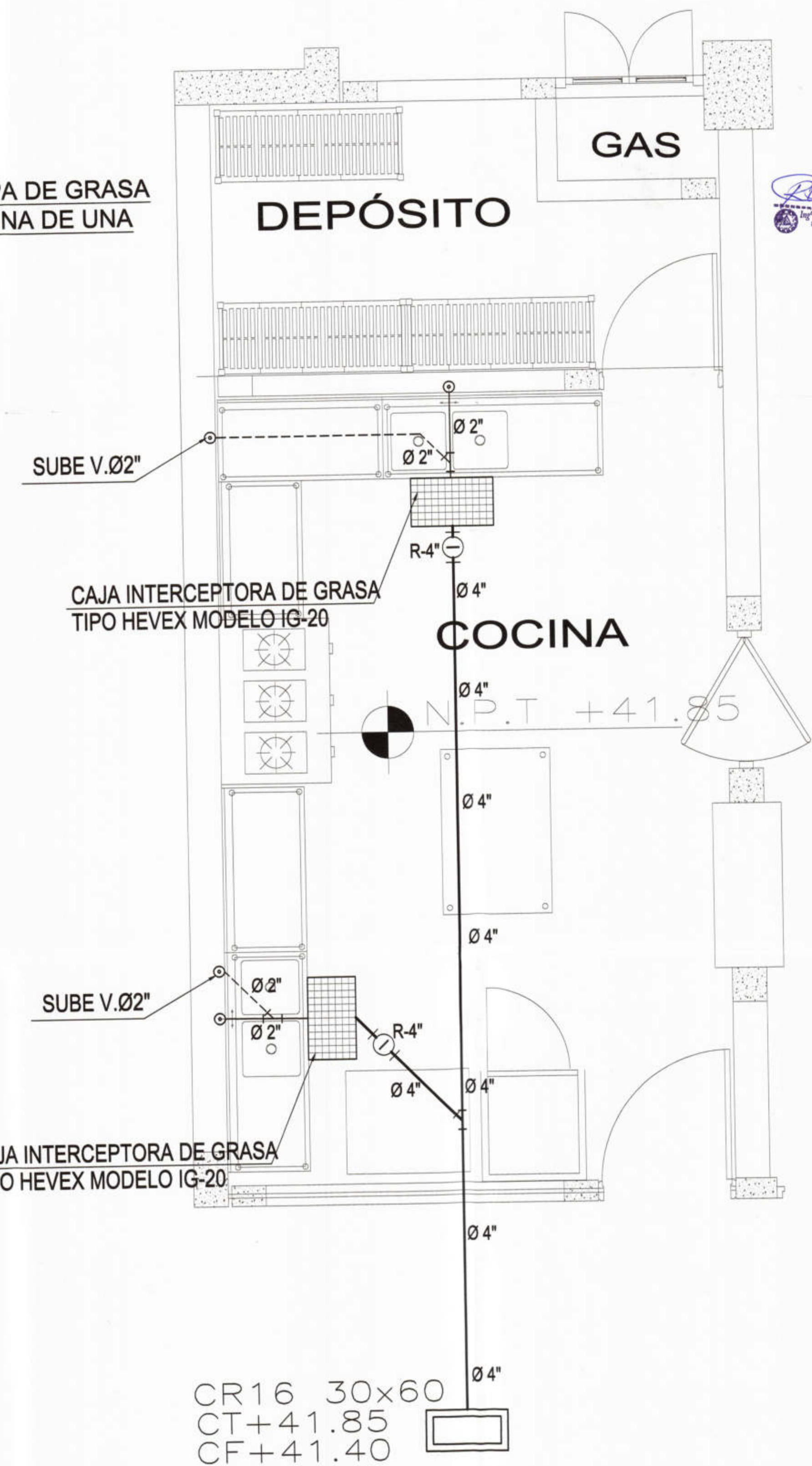
RED DESAGUE - COCINA PRIMARIA MODULO 01 1/25
