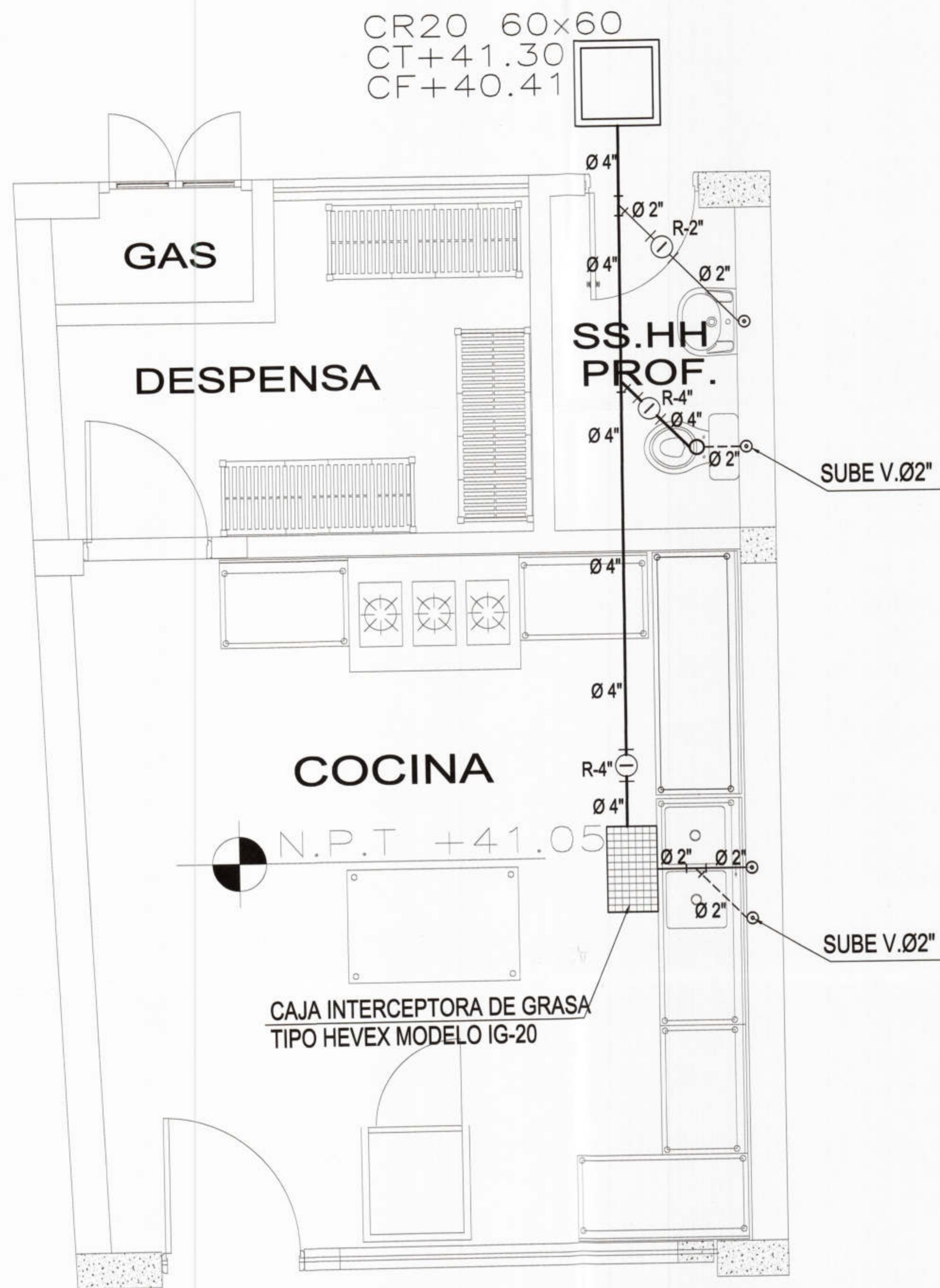
RED DESAGUE - COCINA NIVEL INICIAL MODULO 05 1/25
