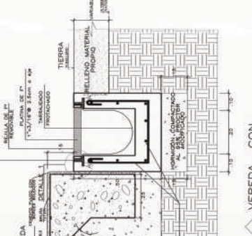
DETALLE 1 -CANALETA PLUVIAL CON REJILLA
