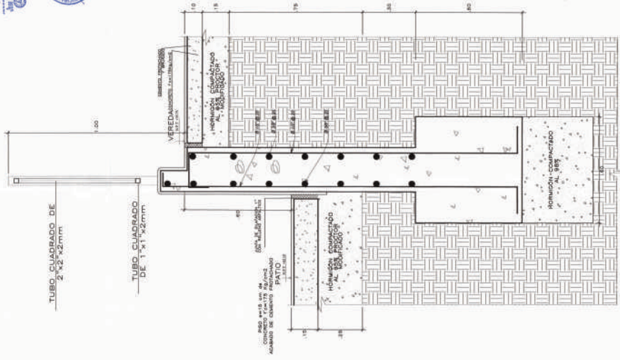
24 - DETALLE DE VEREDA - MURO CONTENCIÓN-PATIO
