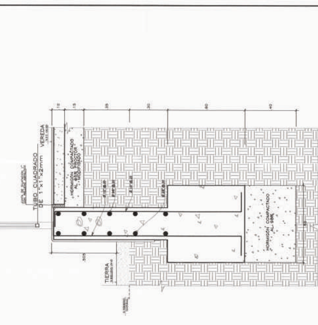
20- DETALLE DE VEREDA - MURO CONTENCIÓN-TIERRA
