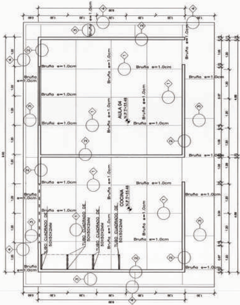
PRIMERA PLANTA-PISOS ESCALA: 1/100
