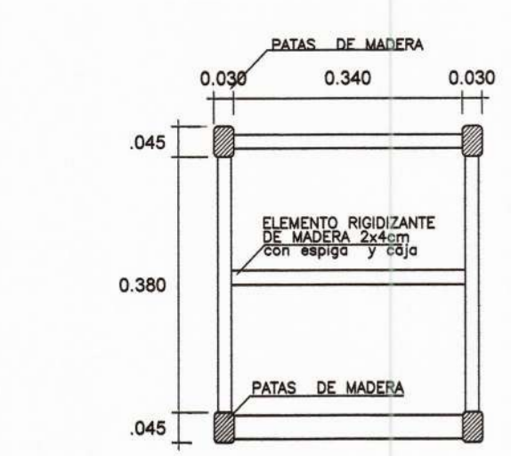
PLANTA DE ESTRUCTURA DE LA SILLA ESC. 1/10
