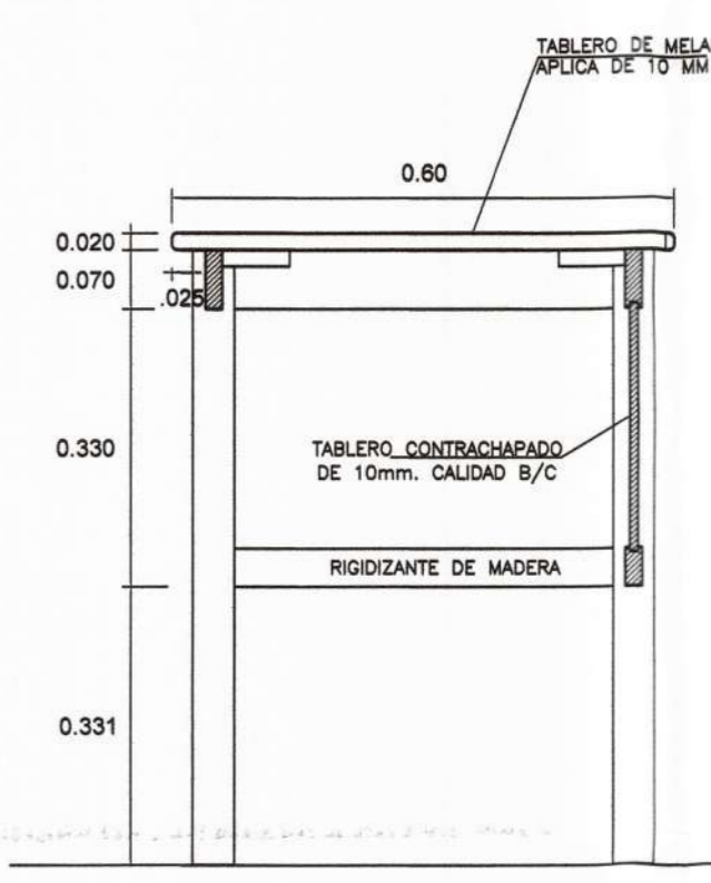
CORTE C-C ESC. 1/10
