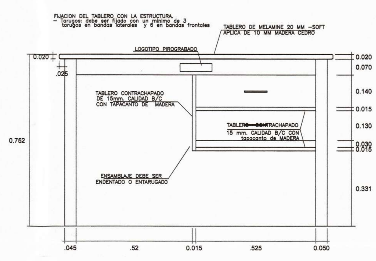
ELEVACION FRONTAL ESC. 1/10
