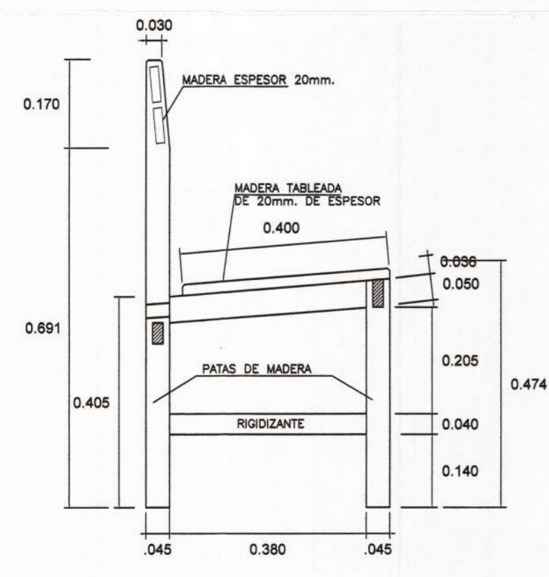
ELEVACION LATERAL ESC. 1/10
