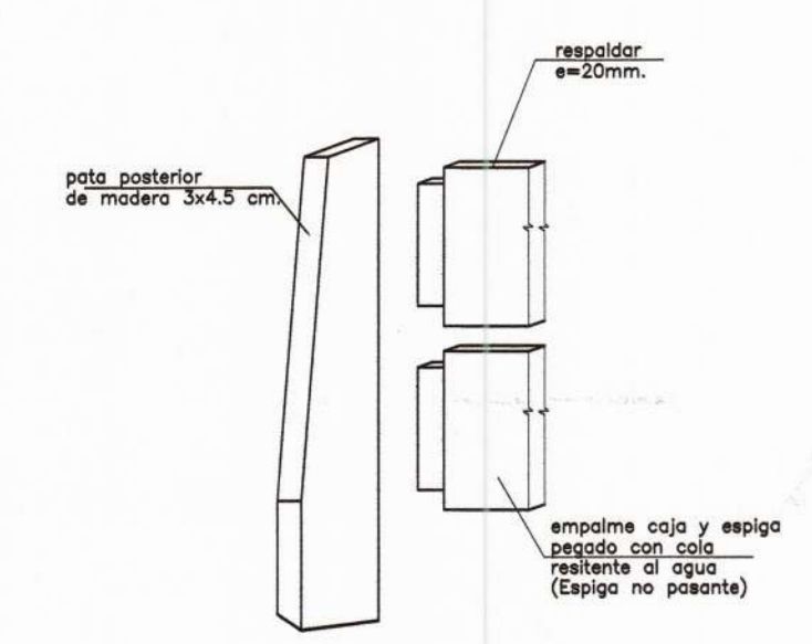
DETALLE A ESC. 1/2.5
