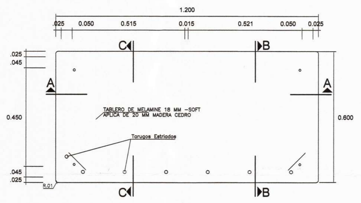
PLANTA ESC. 1/10
