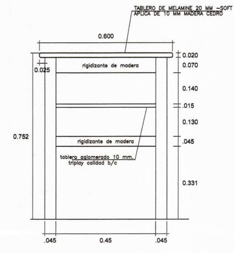
ELEVACION LATERAL ESC. 1/10
