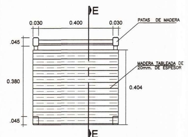
PLANTA ESC. 1/10
