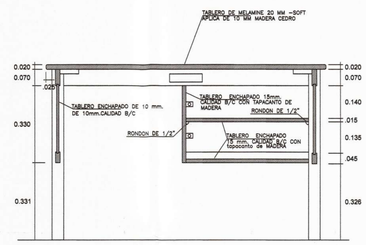
CORTE A-A ESC. 1/10
