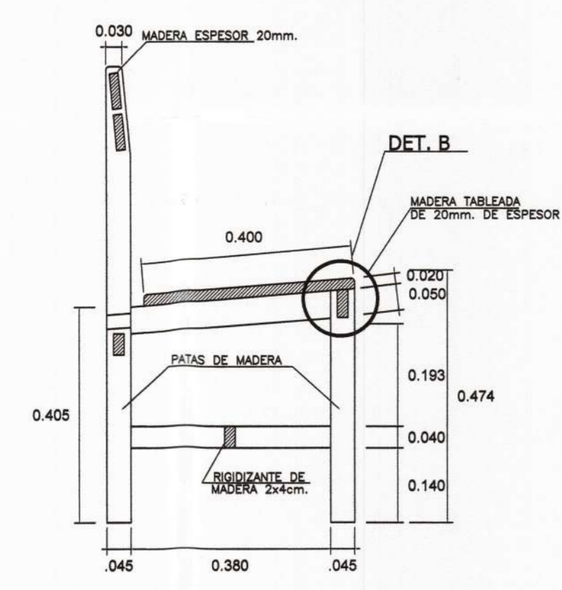
CORTE E-E ESC. 1/10
