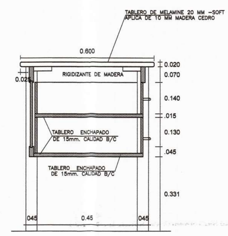
CORTE B-B ESC. 1/10
