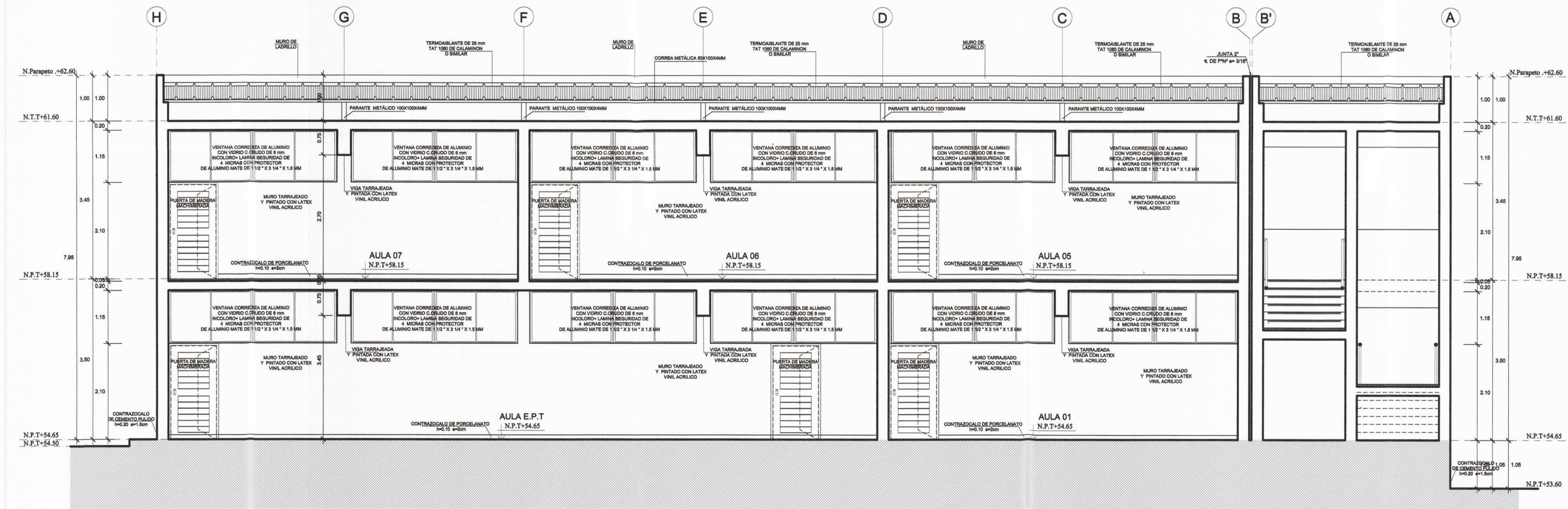
CORTE B-B 1/50
