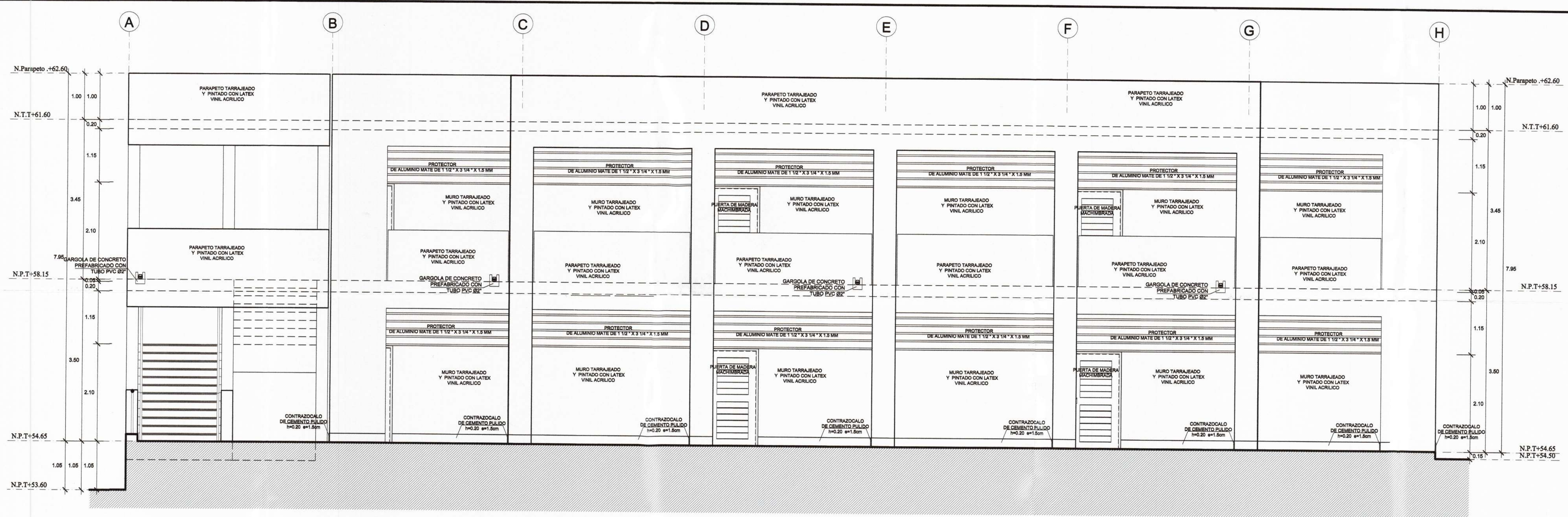
ELEVACIÓN 01 1/50
