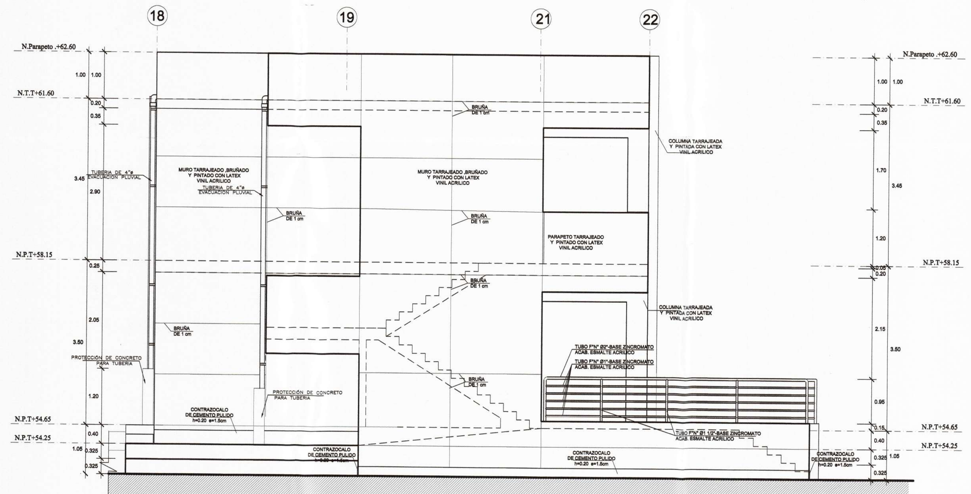
ELEVACIÓN 02 1/50
