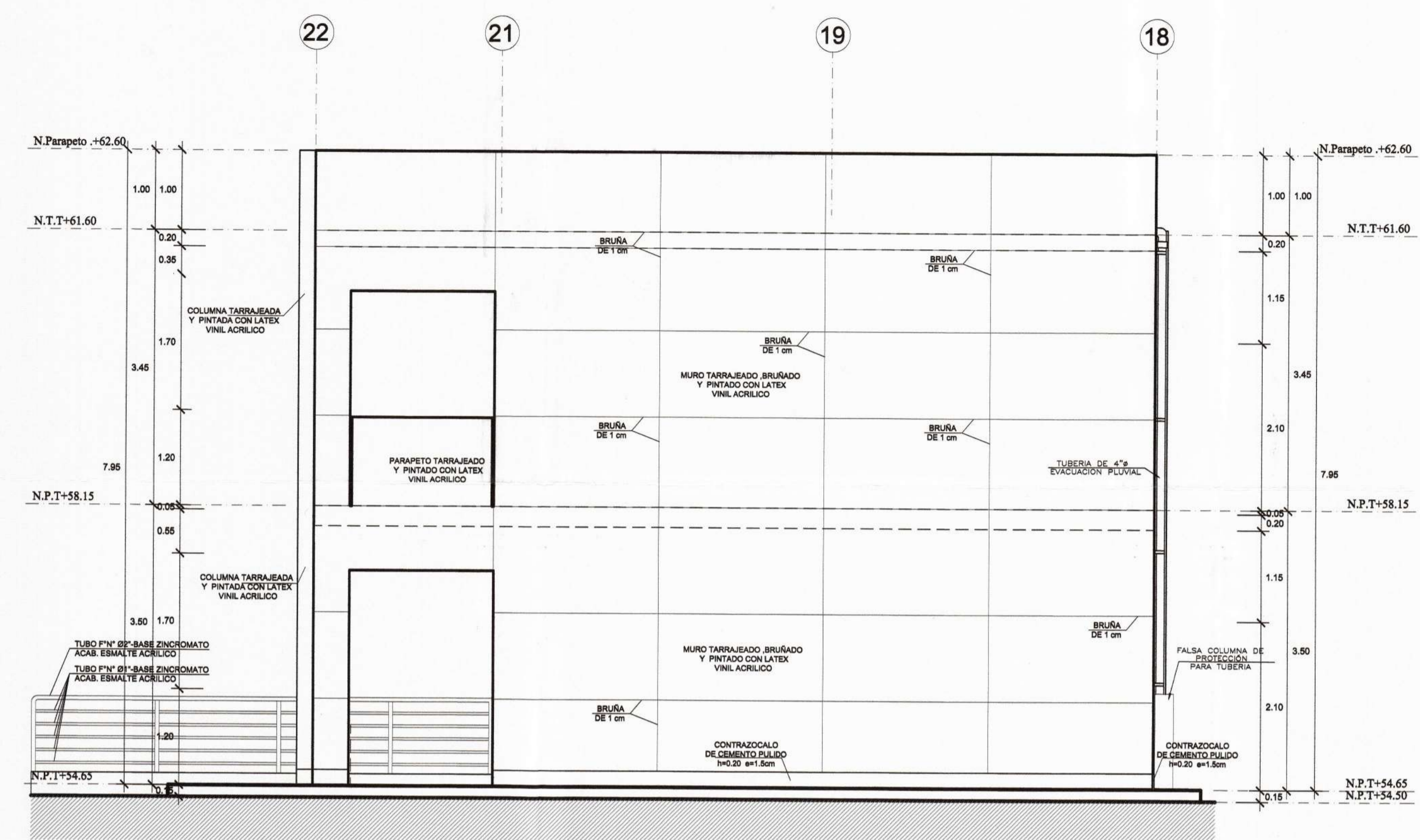
ELEVACIÓN 03 1/50
