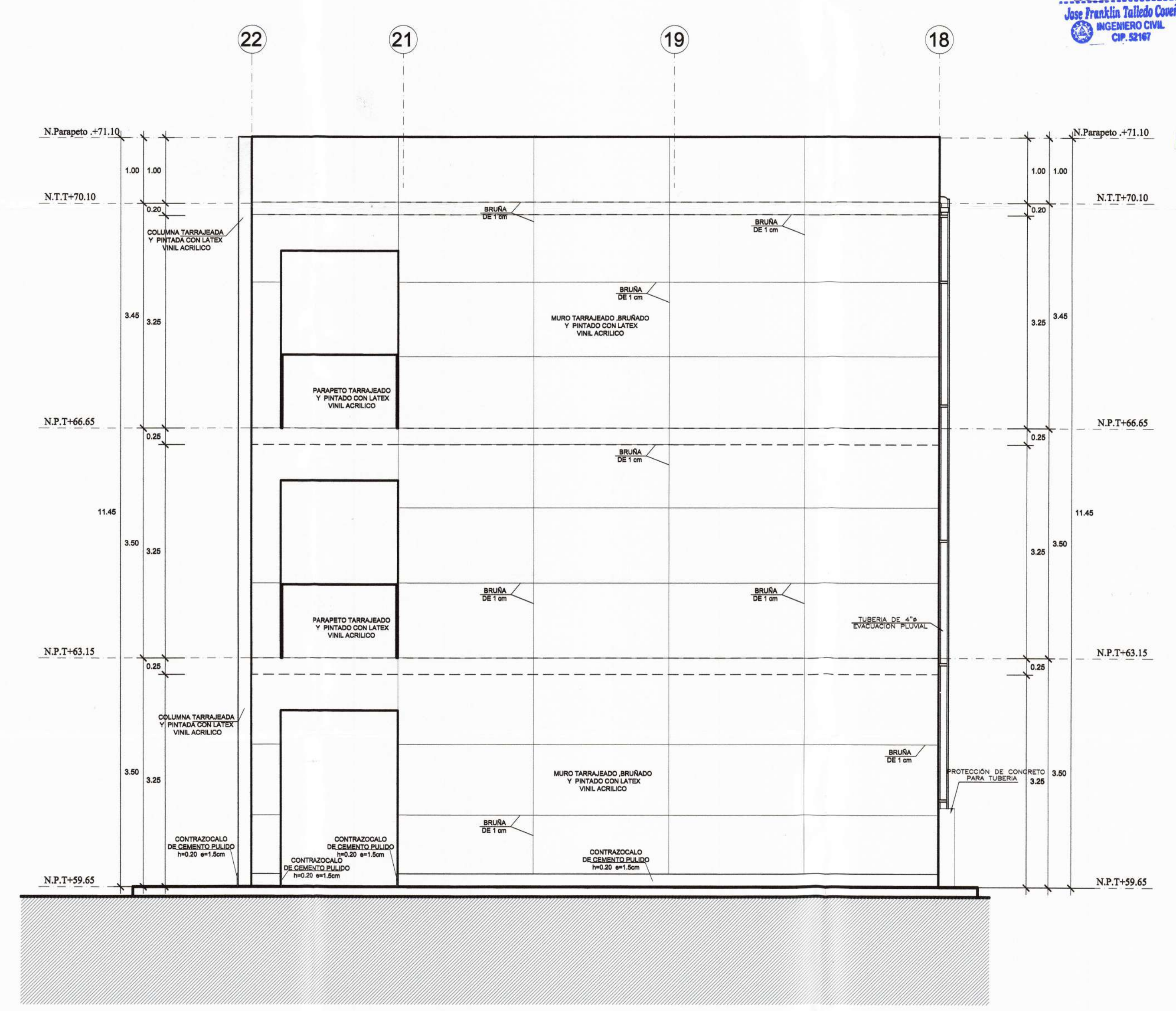
ELEVACIÓN 03 1/50
