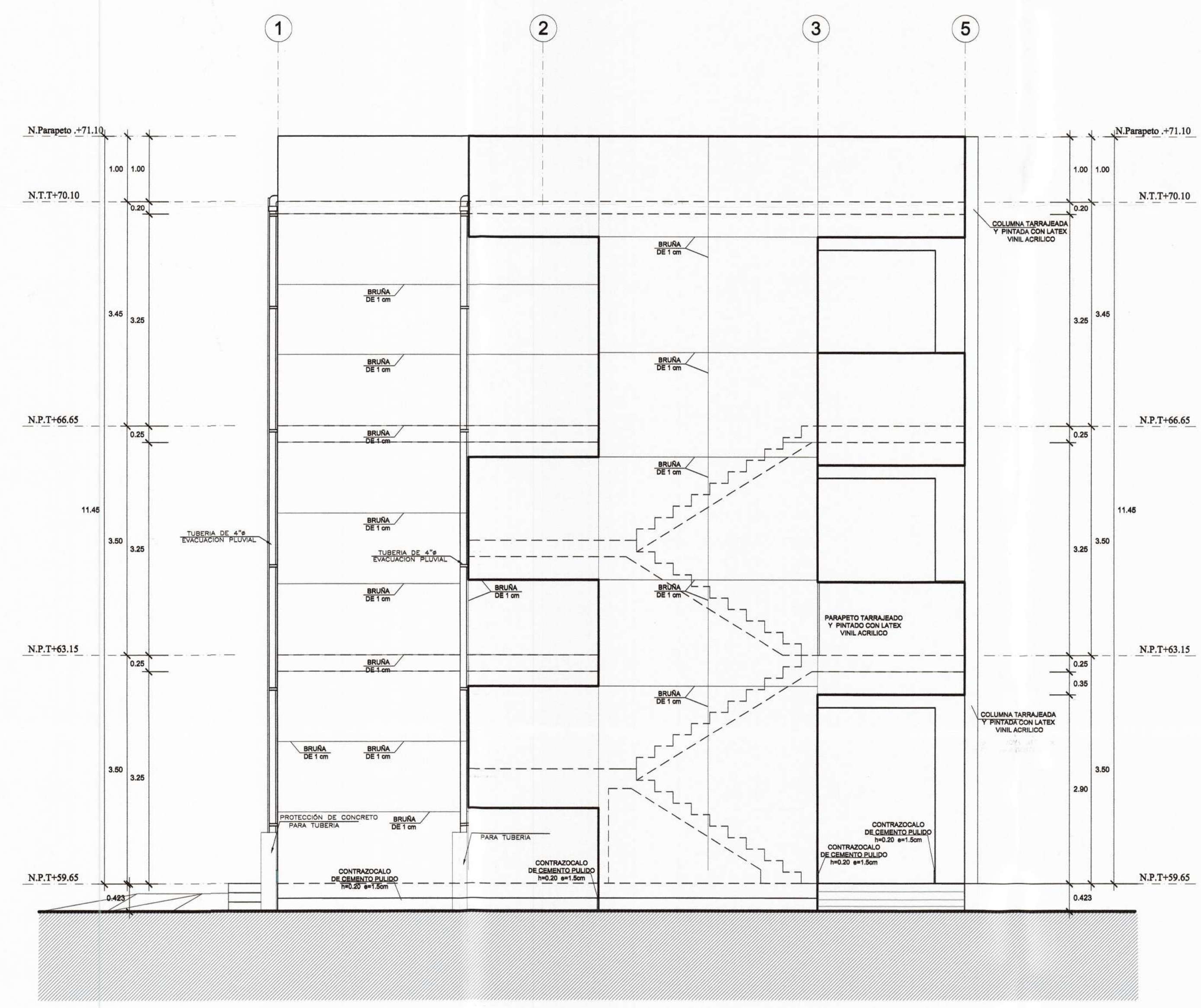
ELEVACIÓN 02 1/50
