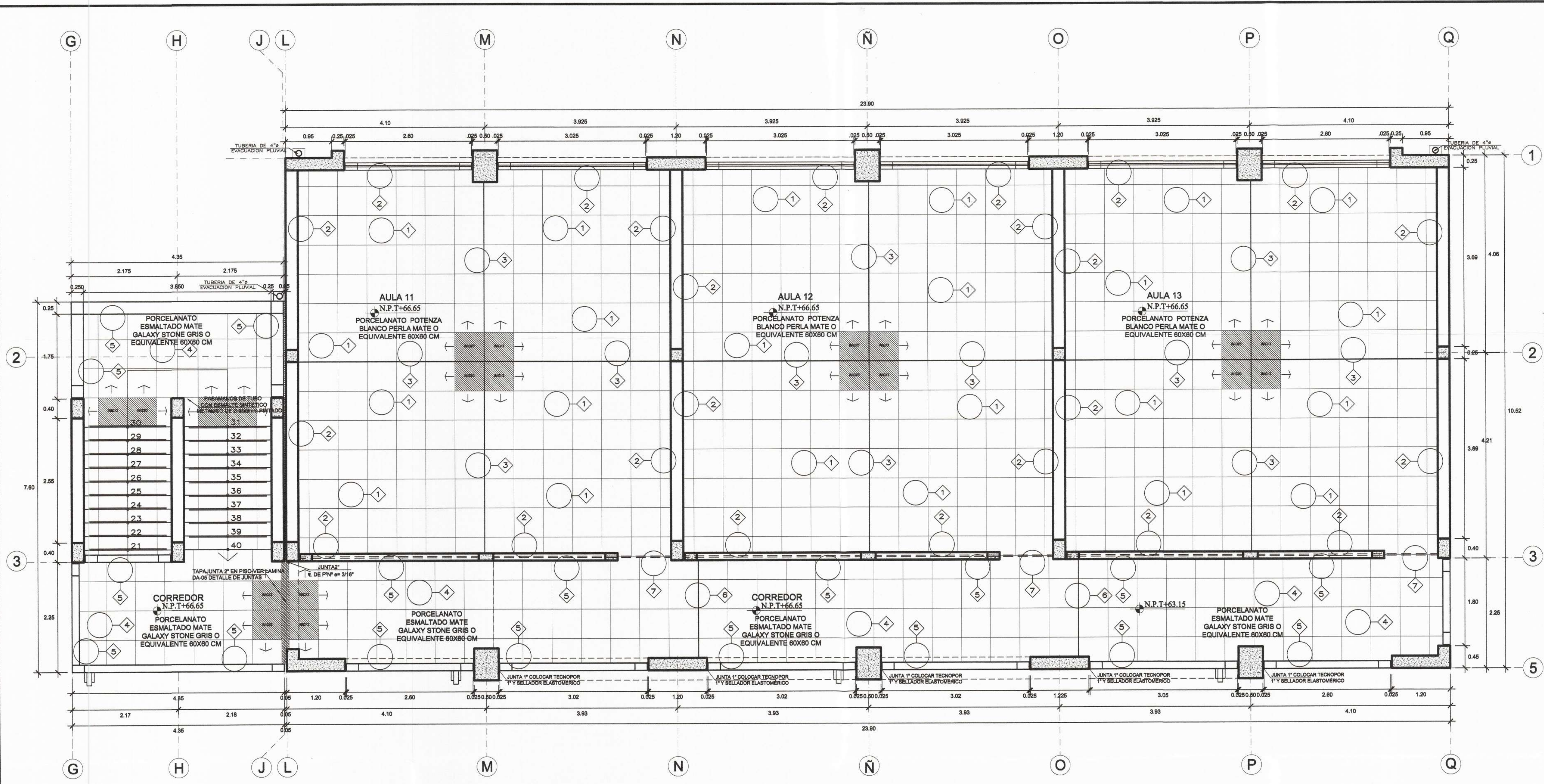
TERCERA PLANTA-PISOS 1/50
