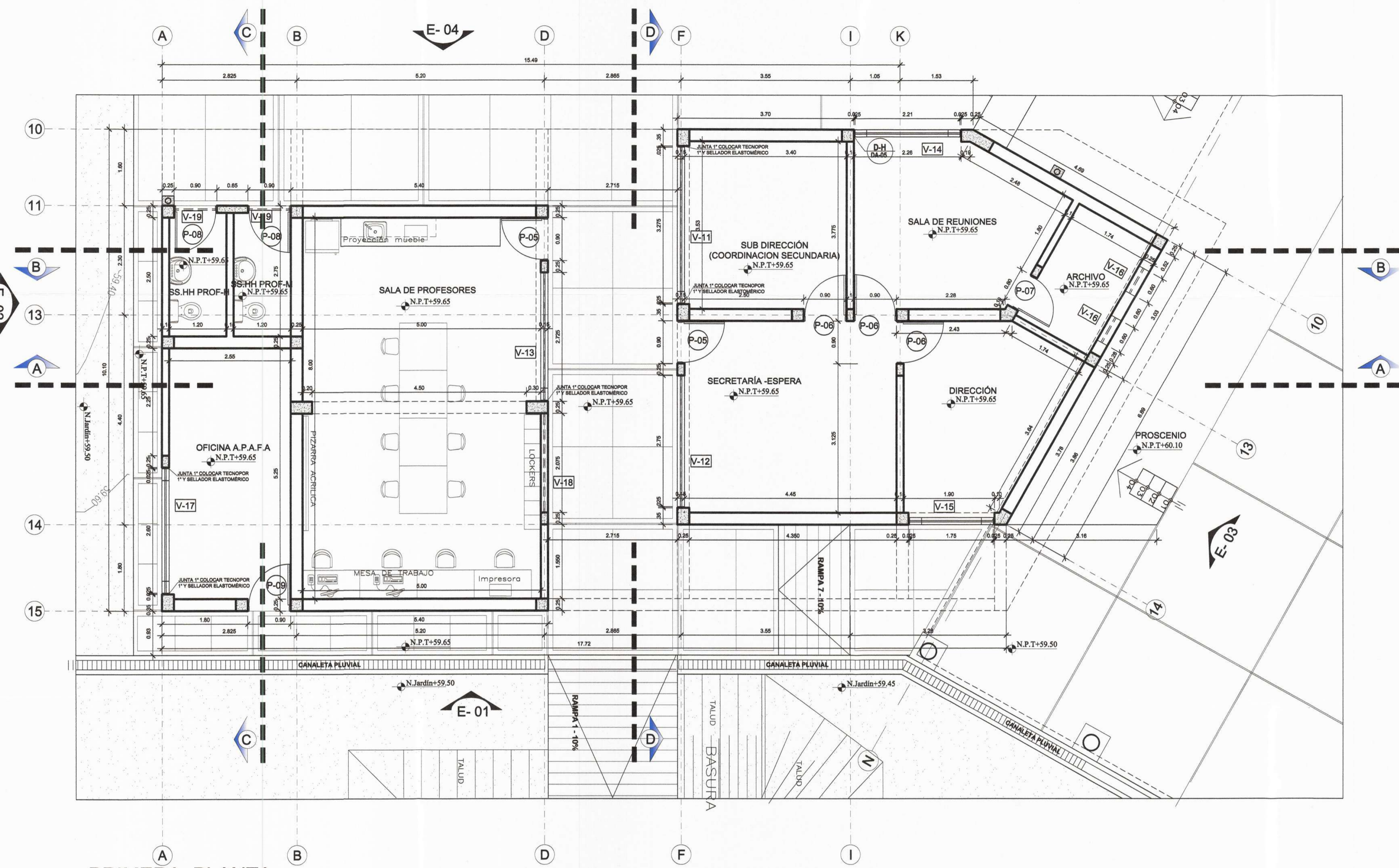
PRIMERA PLANTA 1/50
