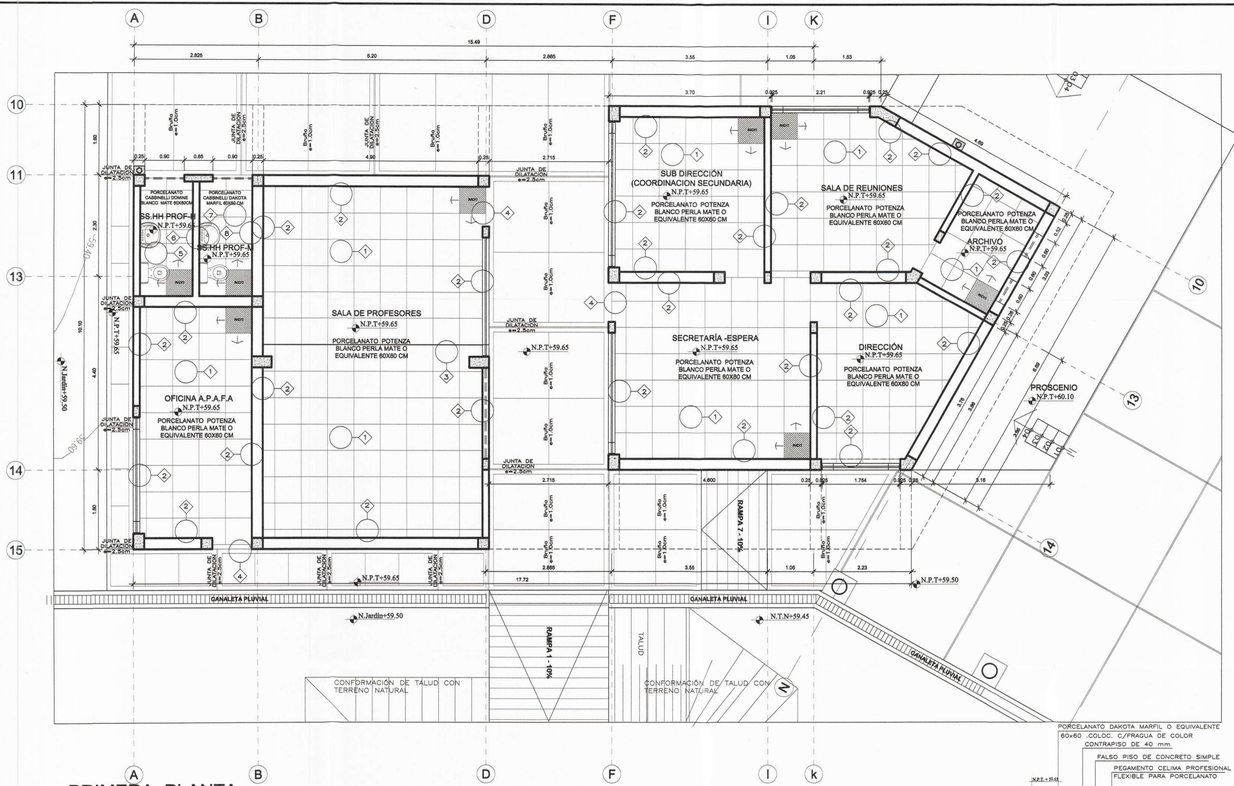
PRIMERA PLANTA 1/50
