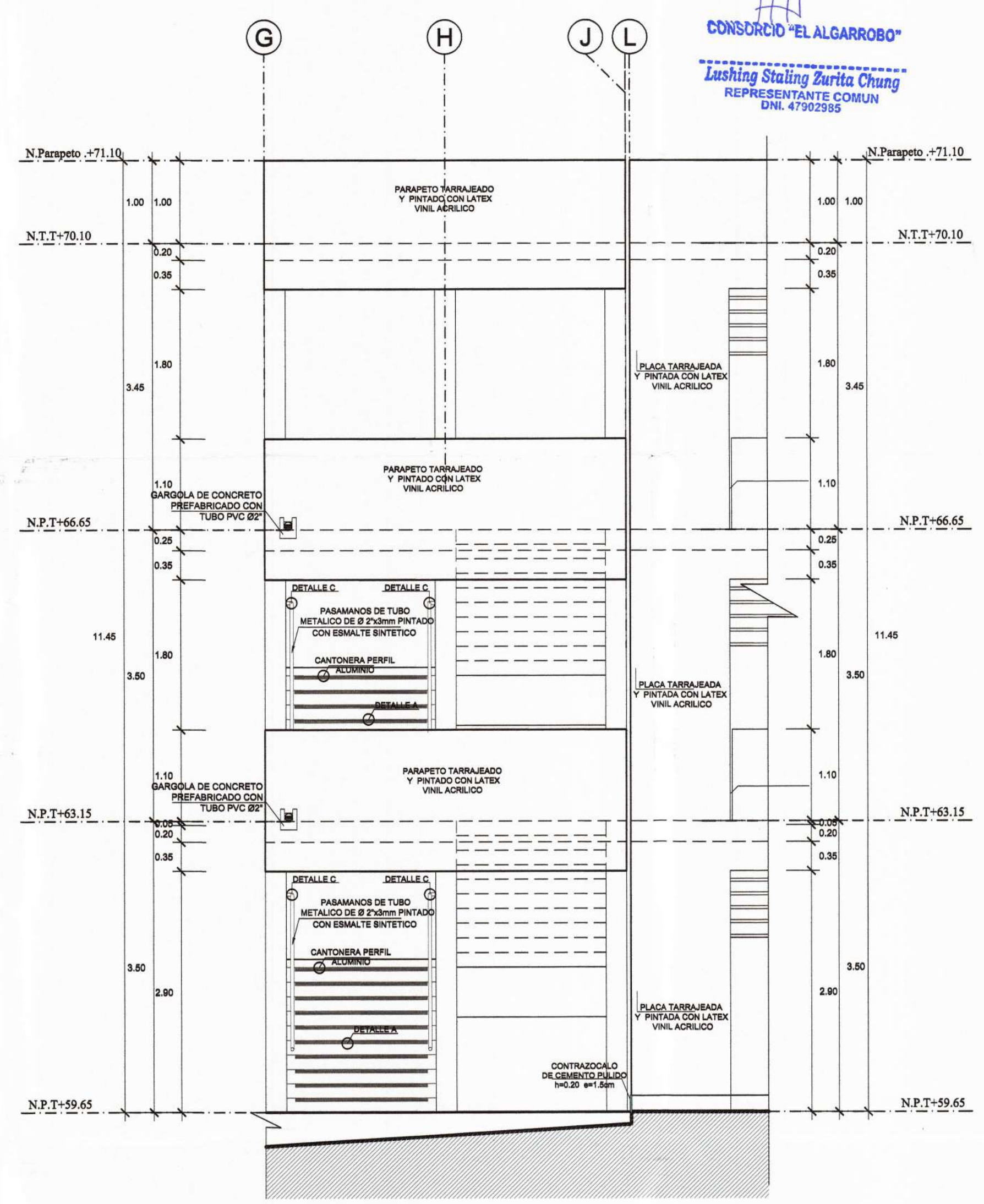
ELEVACIÓN 01 1/50
