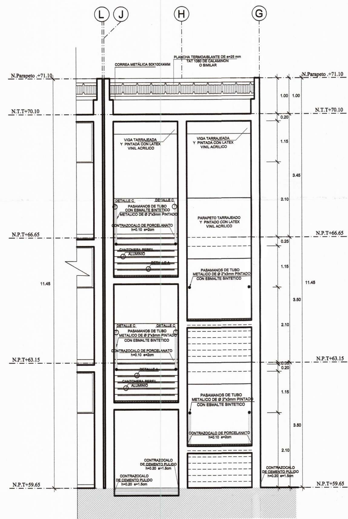
CORTE A-A 1/50
