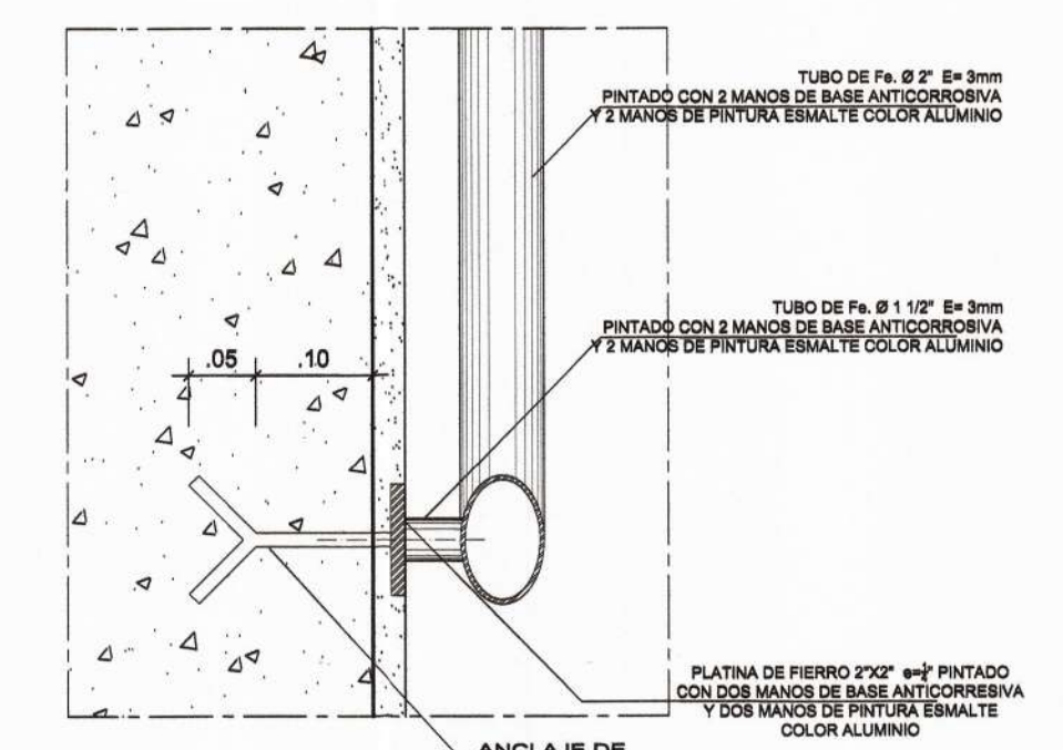
DETALLE C: PASAMANOS ESCALA: 1/10
