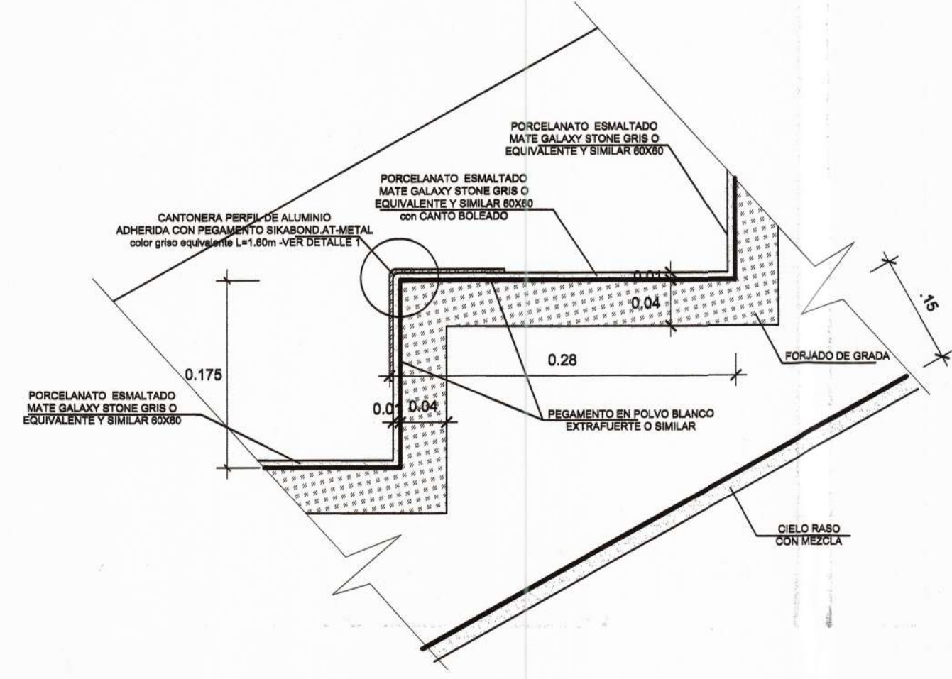
DETALLE A: PASO Y CONTRAPASO ESCALA: 1/10
