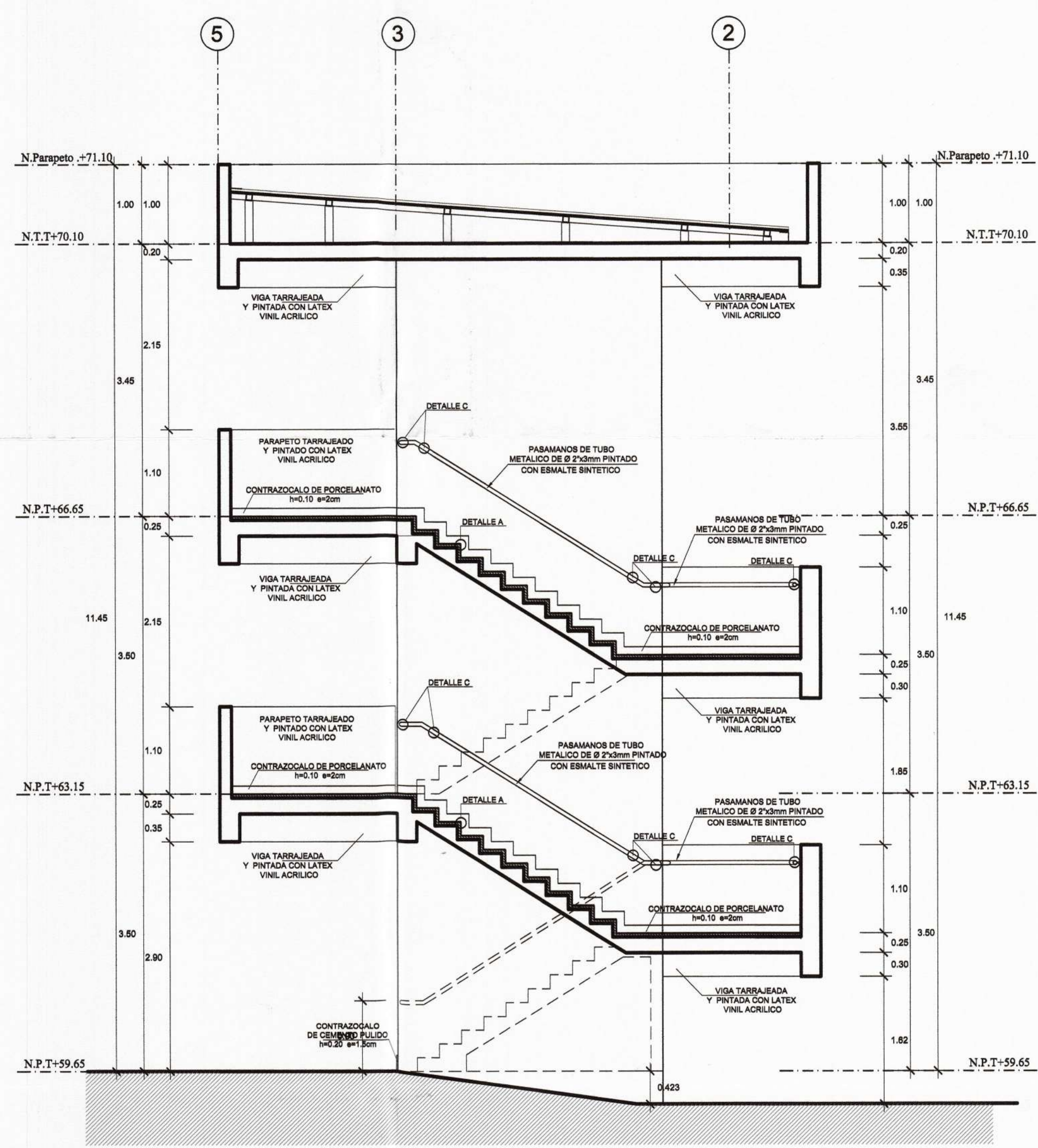
CORTE B-B 1/50
