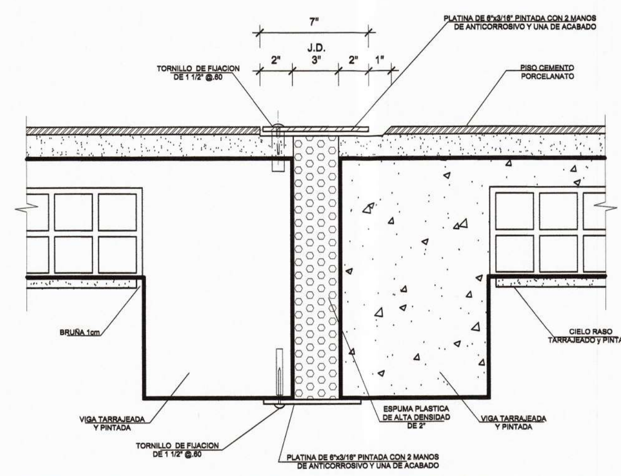
DETALLE B: JUNTA DE DILATACION DEL CORREDOR ESCALA: 1/10
