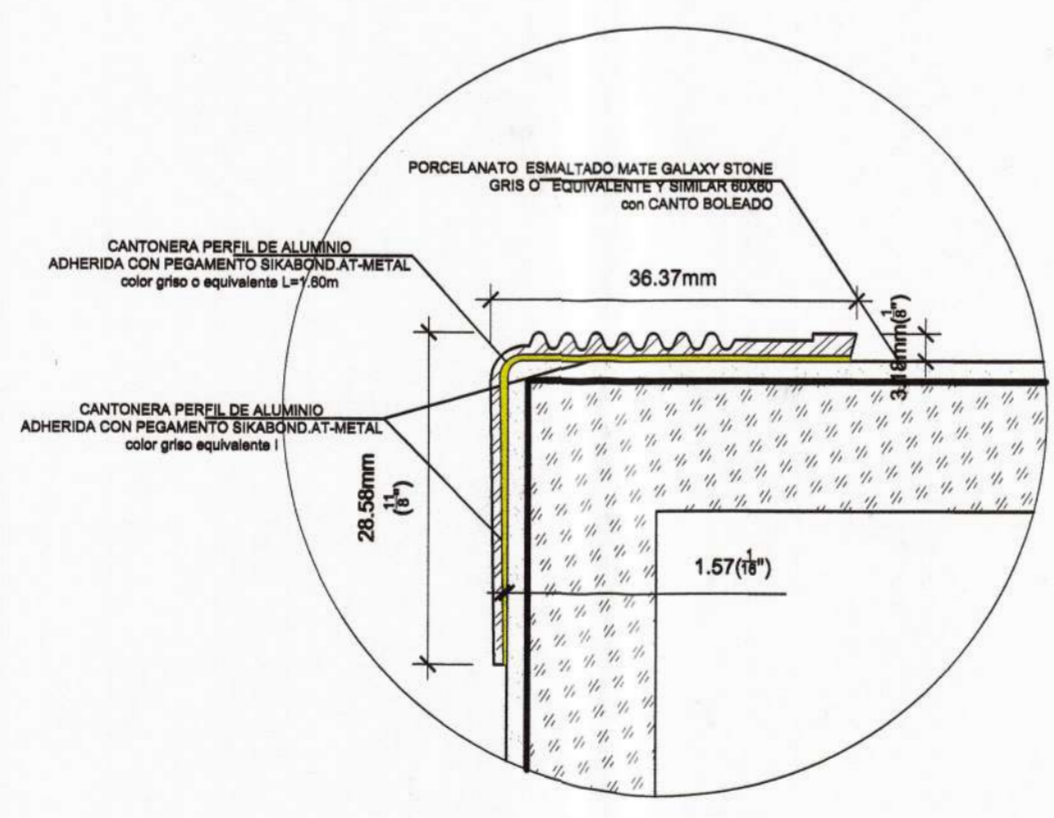
DETALLE 1: DETALLE DE CANTONERA ESCALA : 1/5
