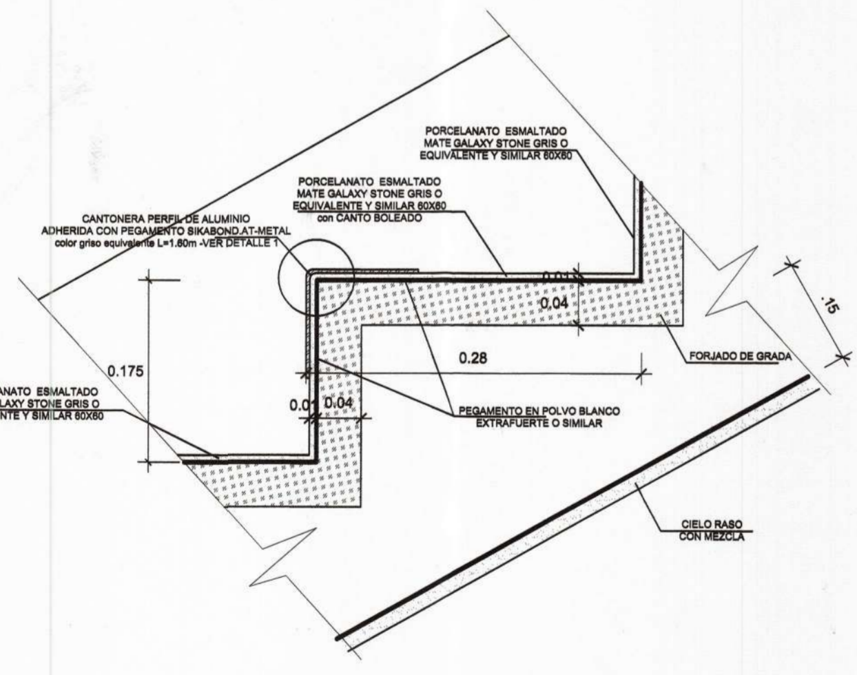
DETALLE A: PASO Y CONTRAPASO ESCALA : 1/10
