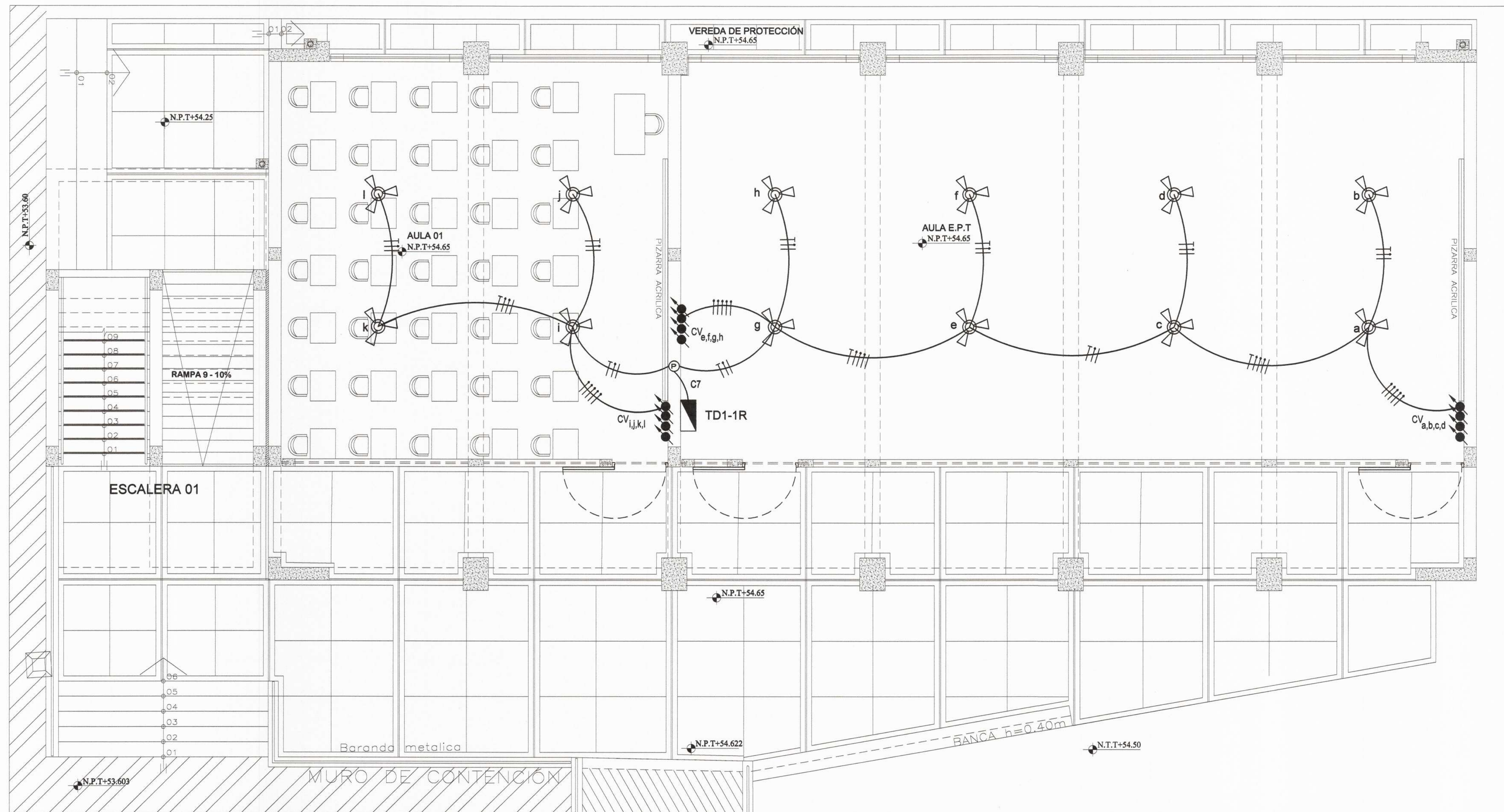
PRIMERA PLANTA-VENTILACIÓN 1/50
