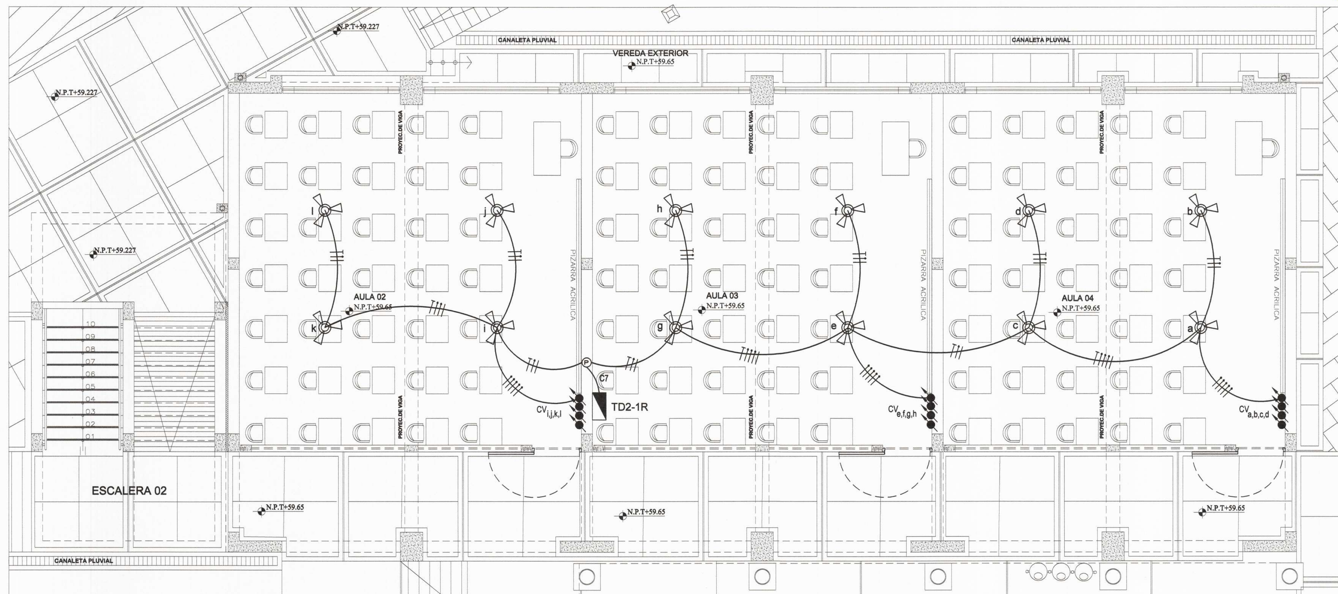
PRIMERA PLANTA-VENTILACIÓN 1/50
