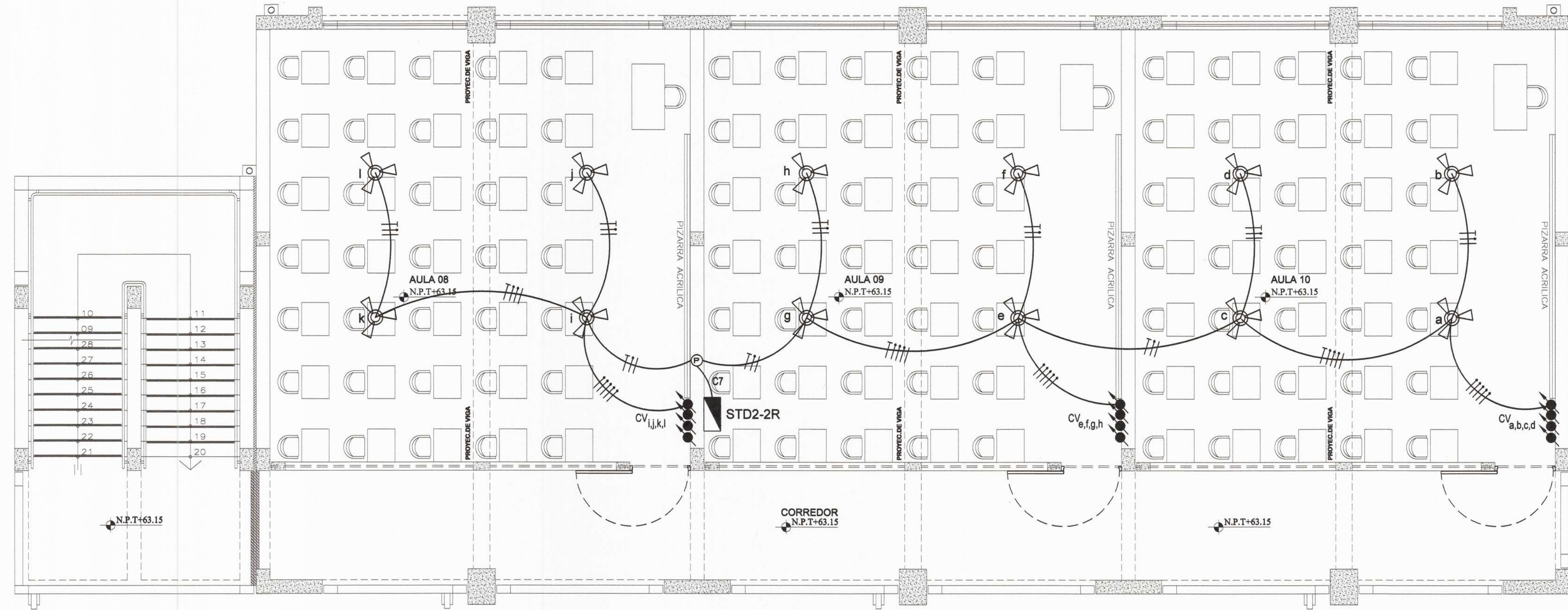
SEGUNDA PLANTA-VENTILACIÓN
