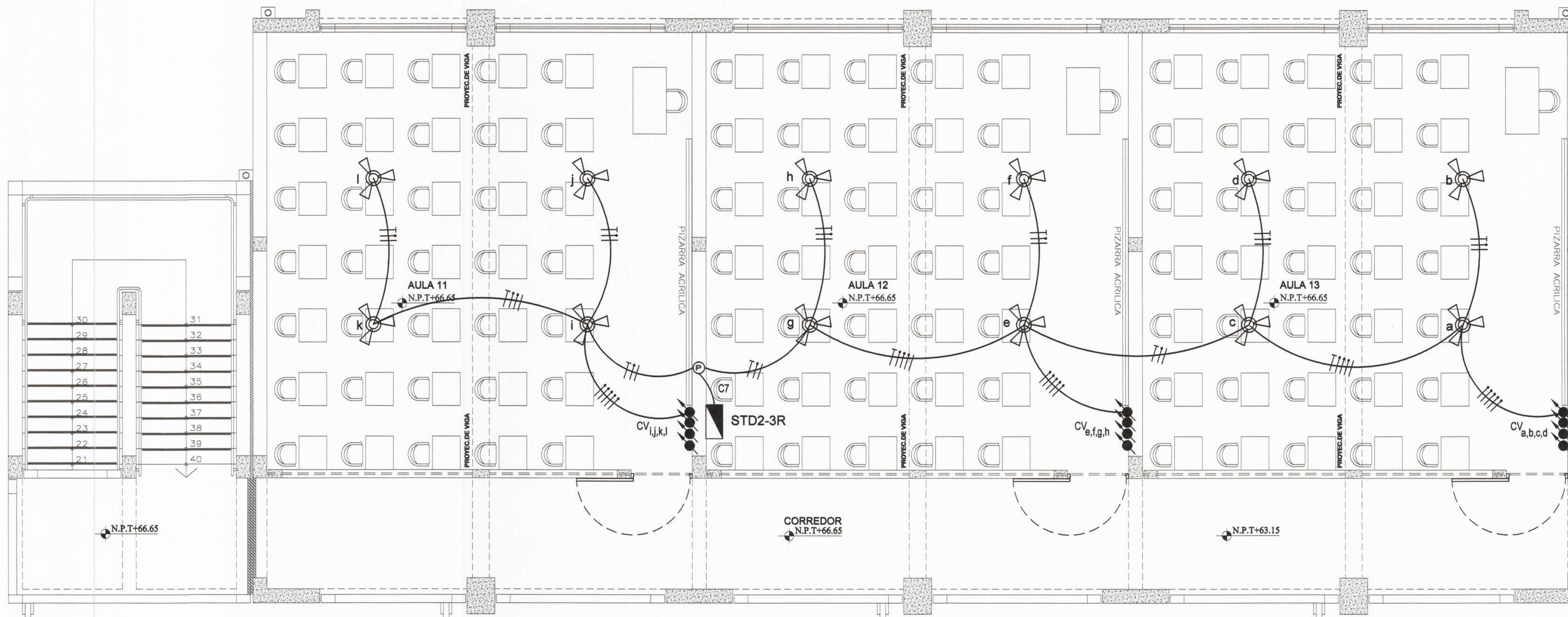
TERCERA PLANTA 1/50
