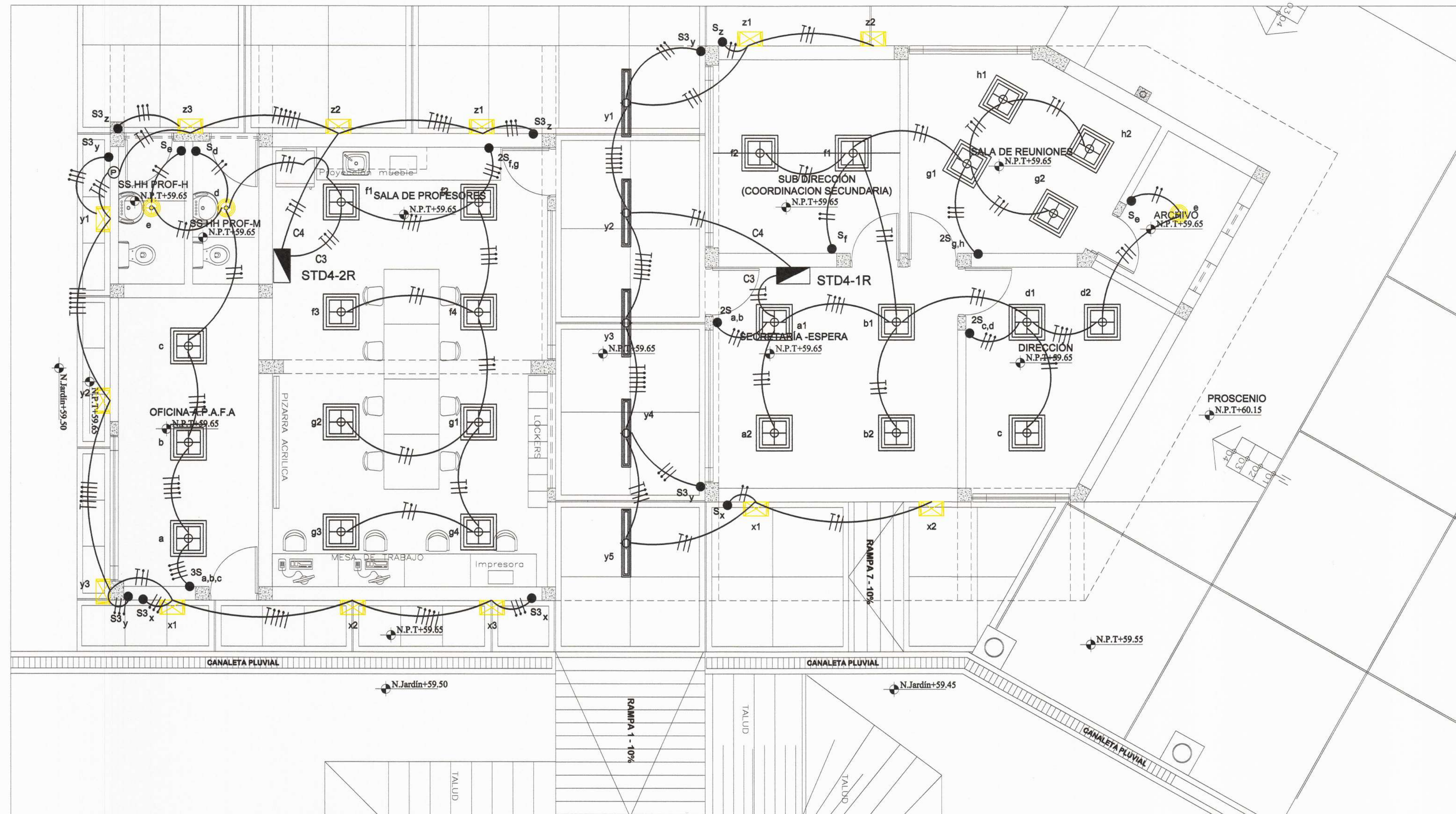
PRIMERA PLANTA-ILUMINACIÓN 1/50
