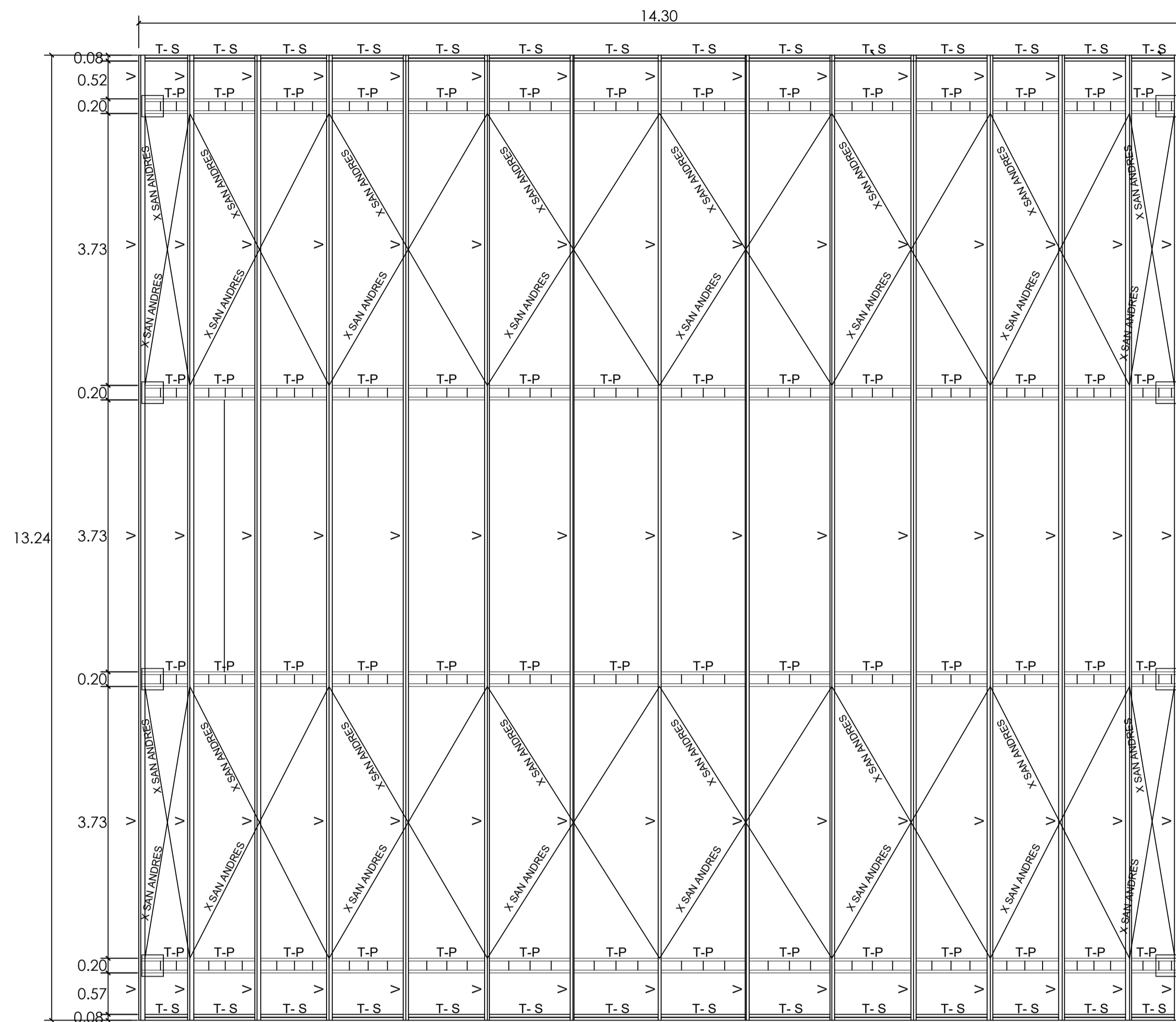
ESTRUCTURA DE TECHO E-1 Esc 1/50
