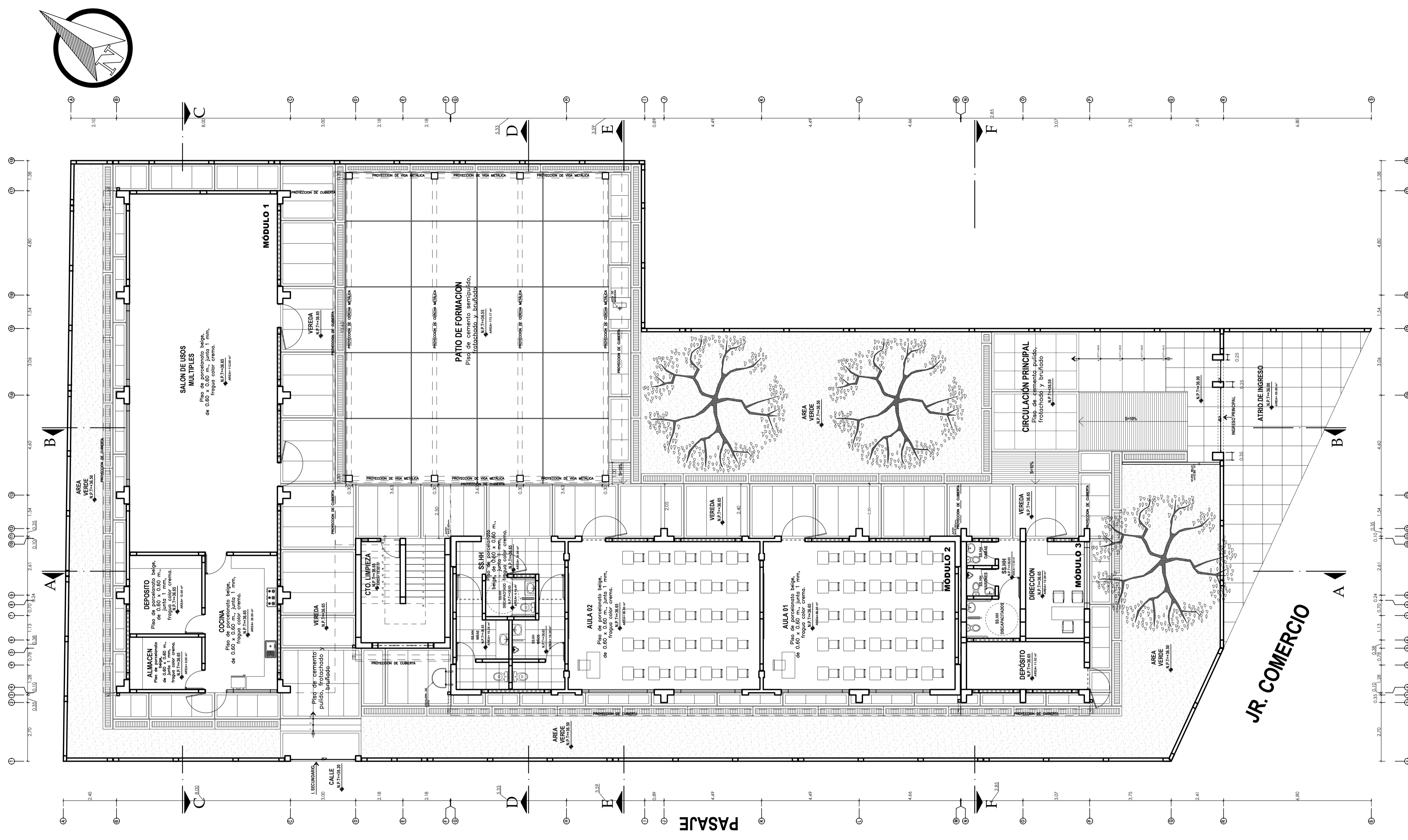
PLANTA GENERAL PRIMER NIVEL Esc 1:100
