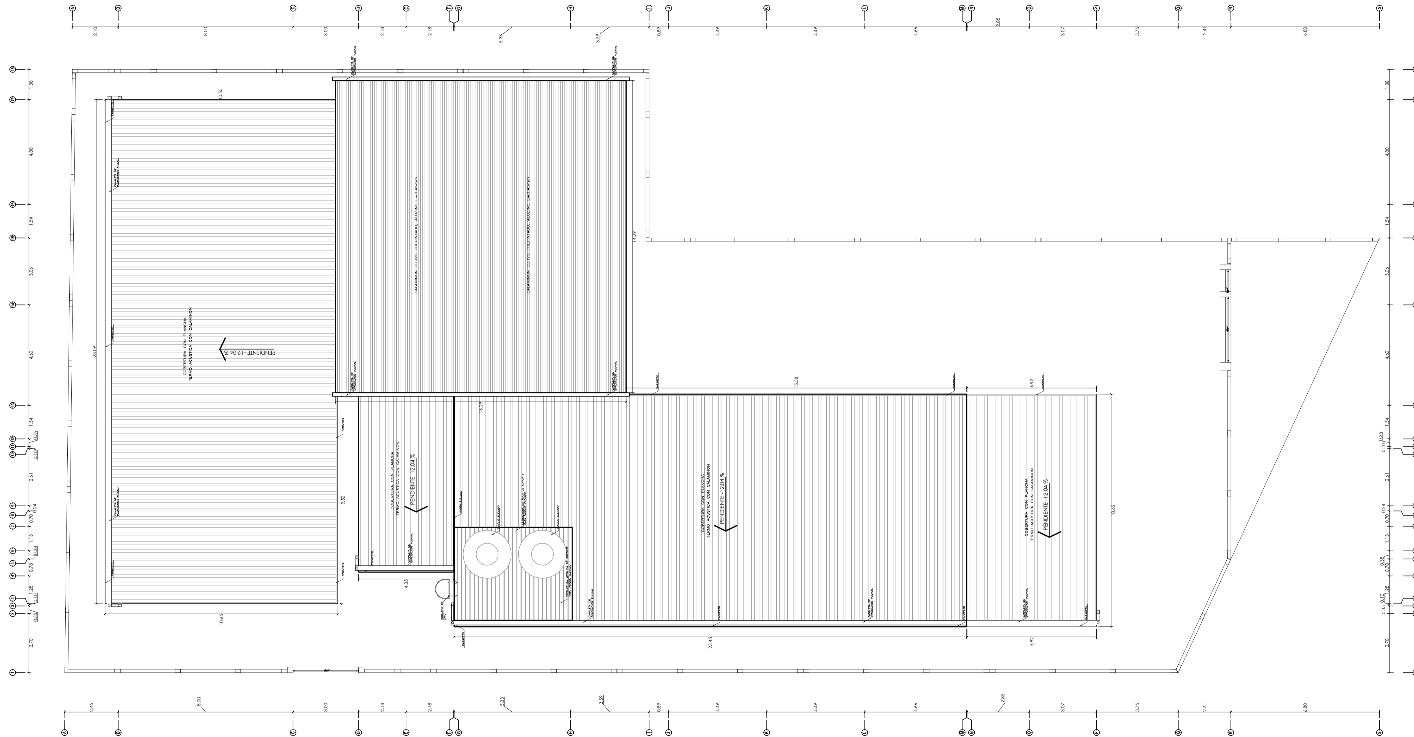
PLANTA DE TECHOS Esc 1:100
