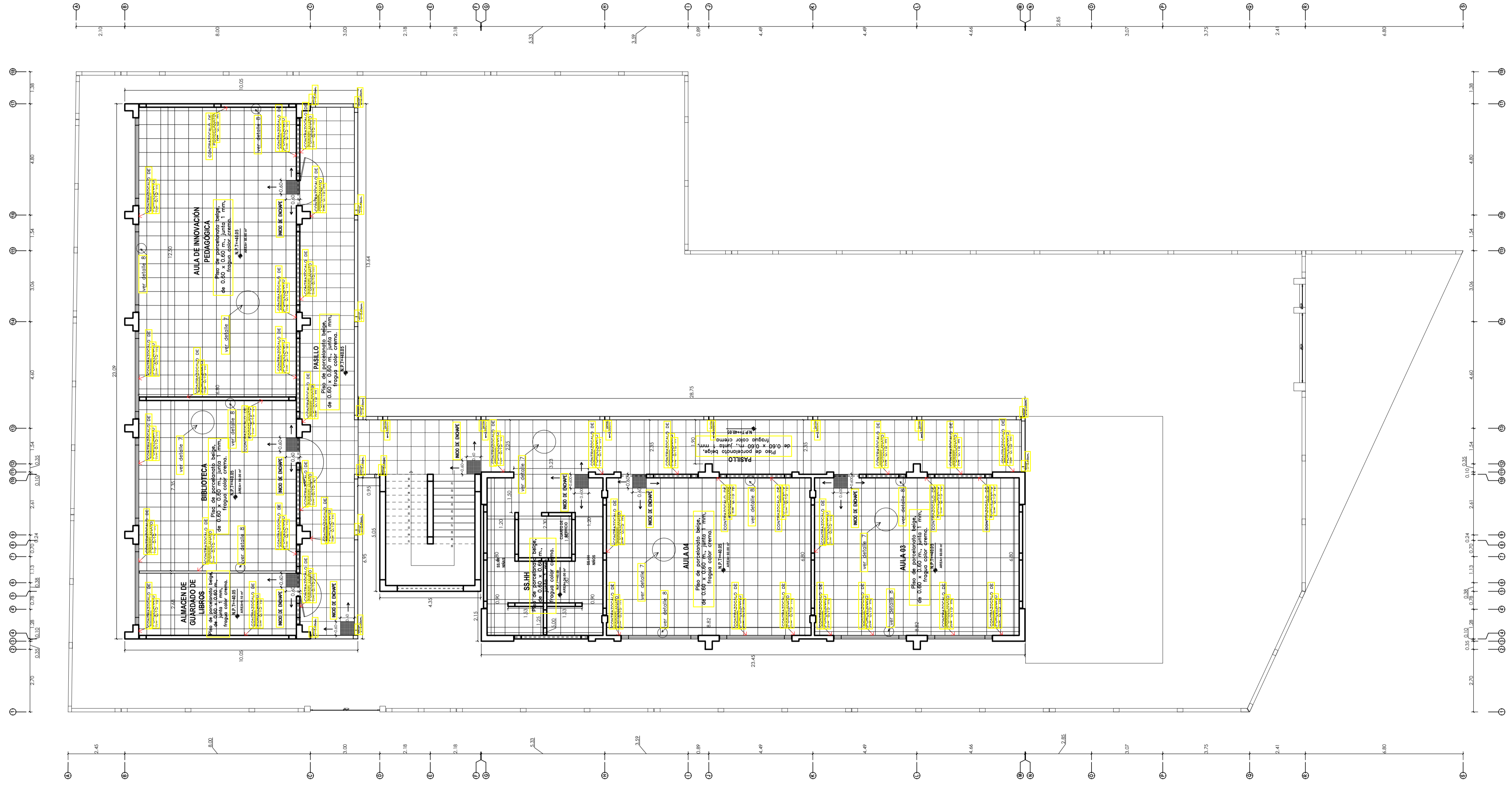
PLANTA DE PISOS SEGUNDO NIVEL Esc 1:100
