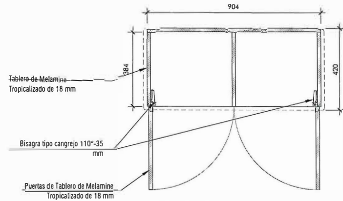
PLANTA 2
