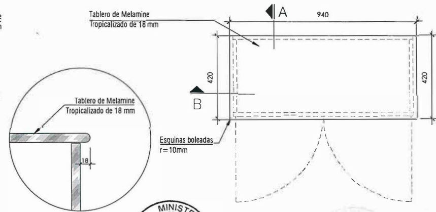
PLANTA 1
