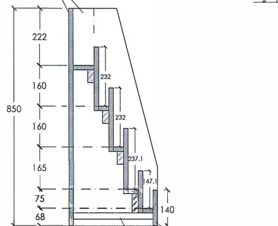
CORTE A-A
