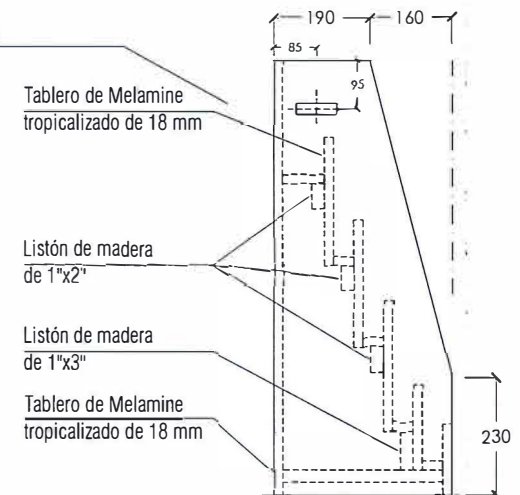
VISTA LATERAL
