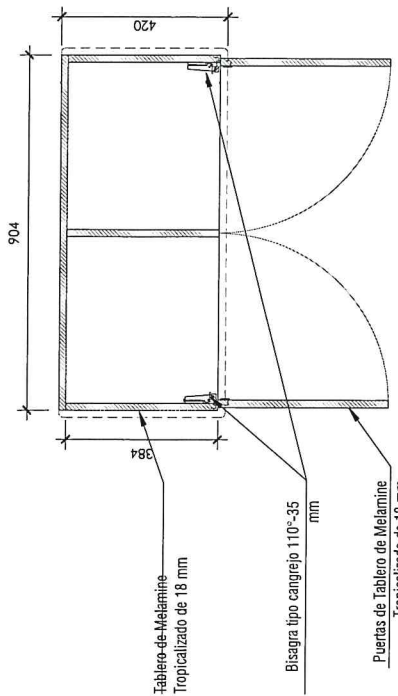
PLANTA 2
