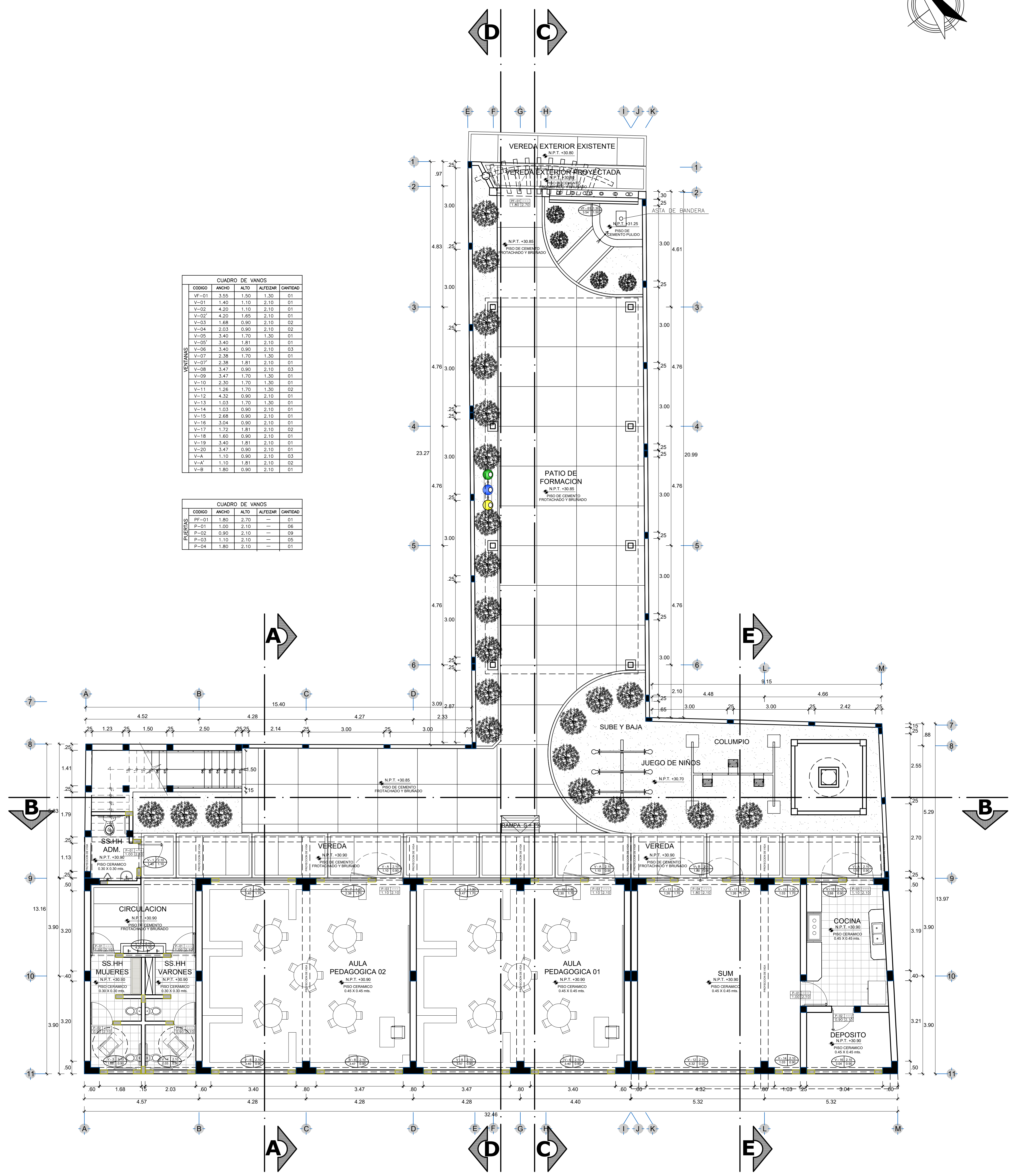
PLANTA GENERAL PRIMER NIVEL ESC: 1/75
