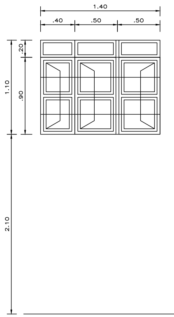
V-01 ESC: 1/25
