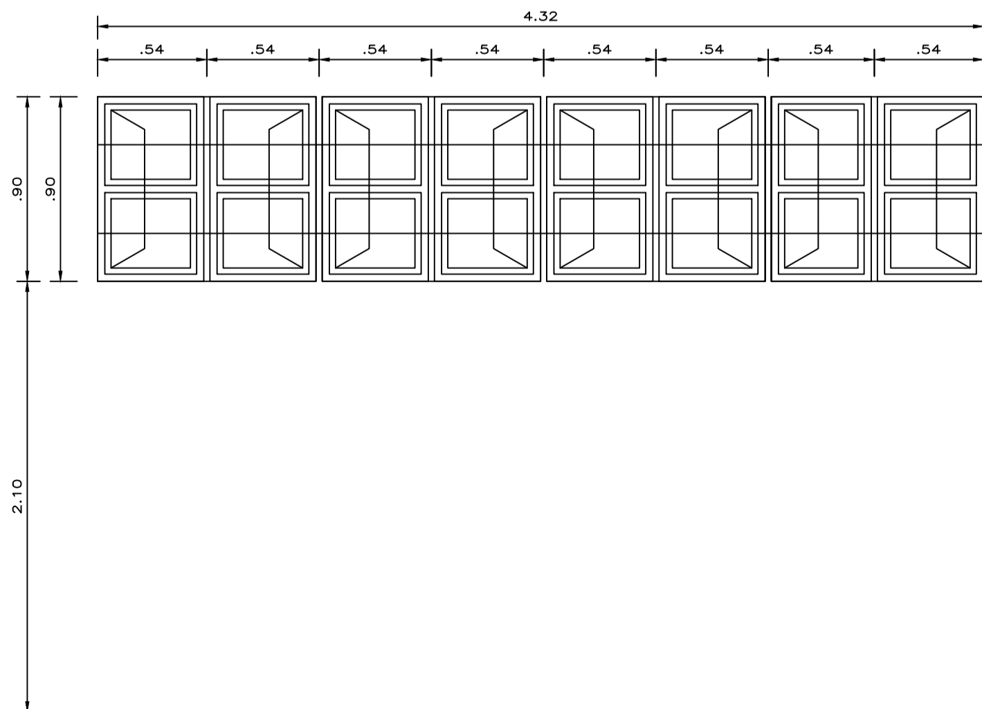
V-12 ESC: 1/25
