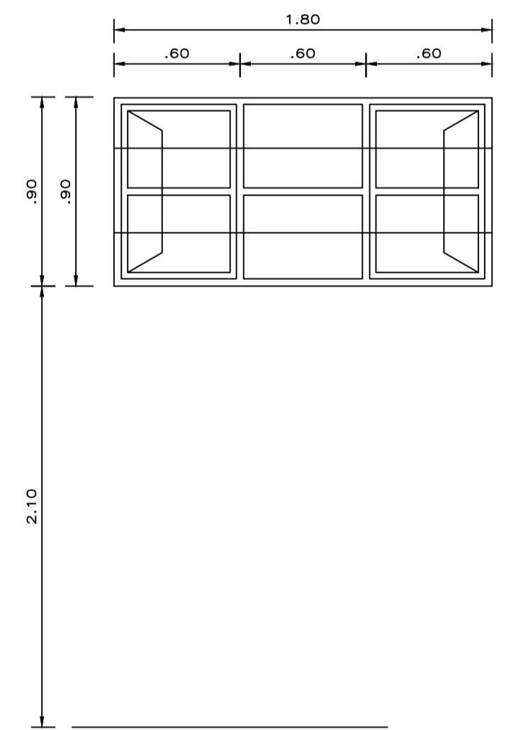
V-B ESC: 1/25
