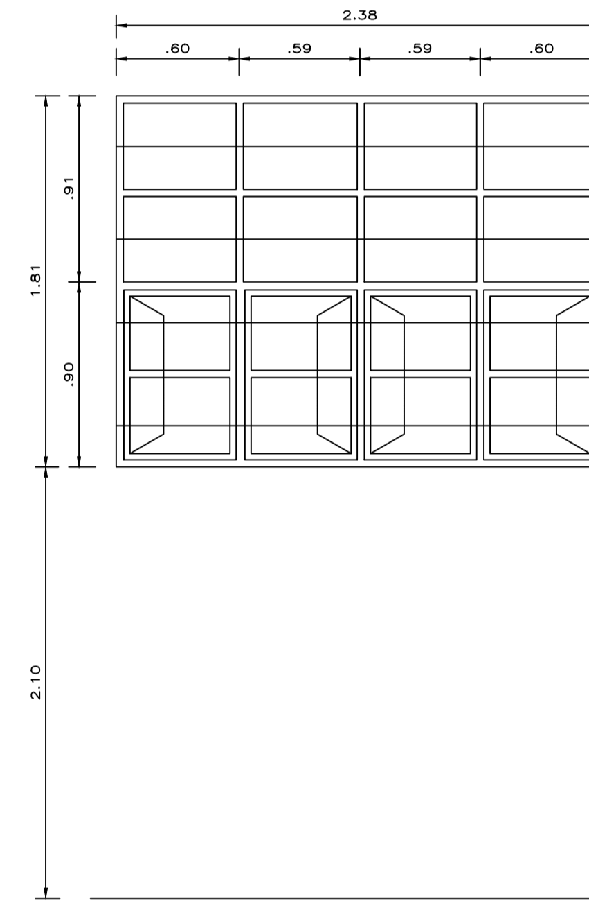
V-07' ESC: 1/25
