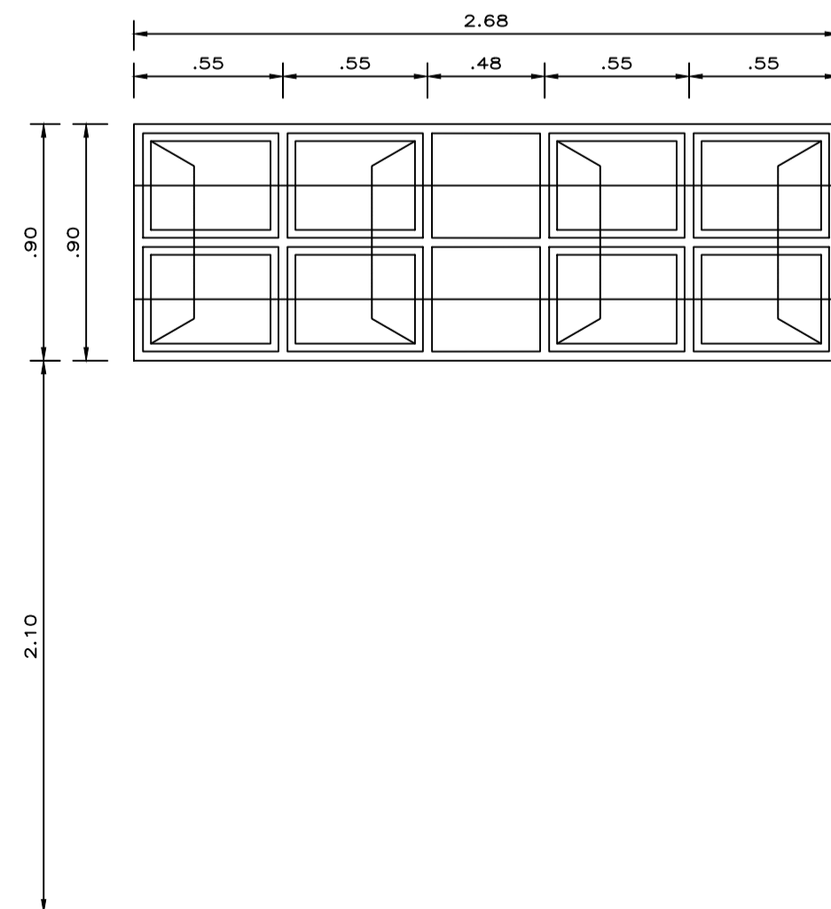
V-15 ESC: 1/25
