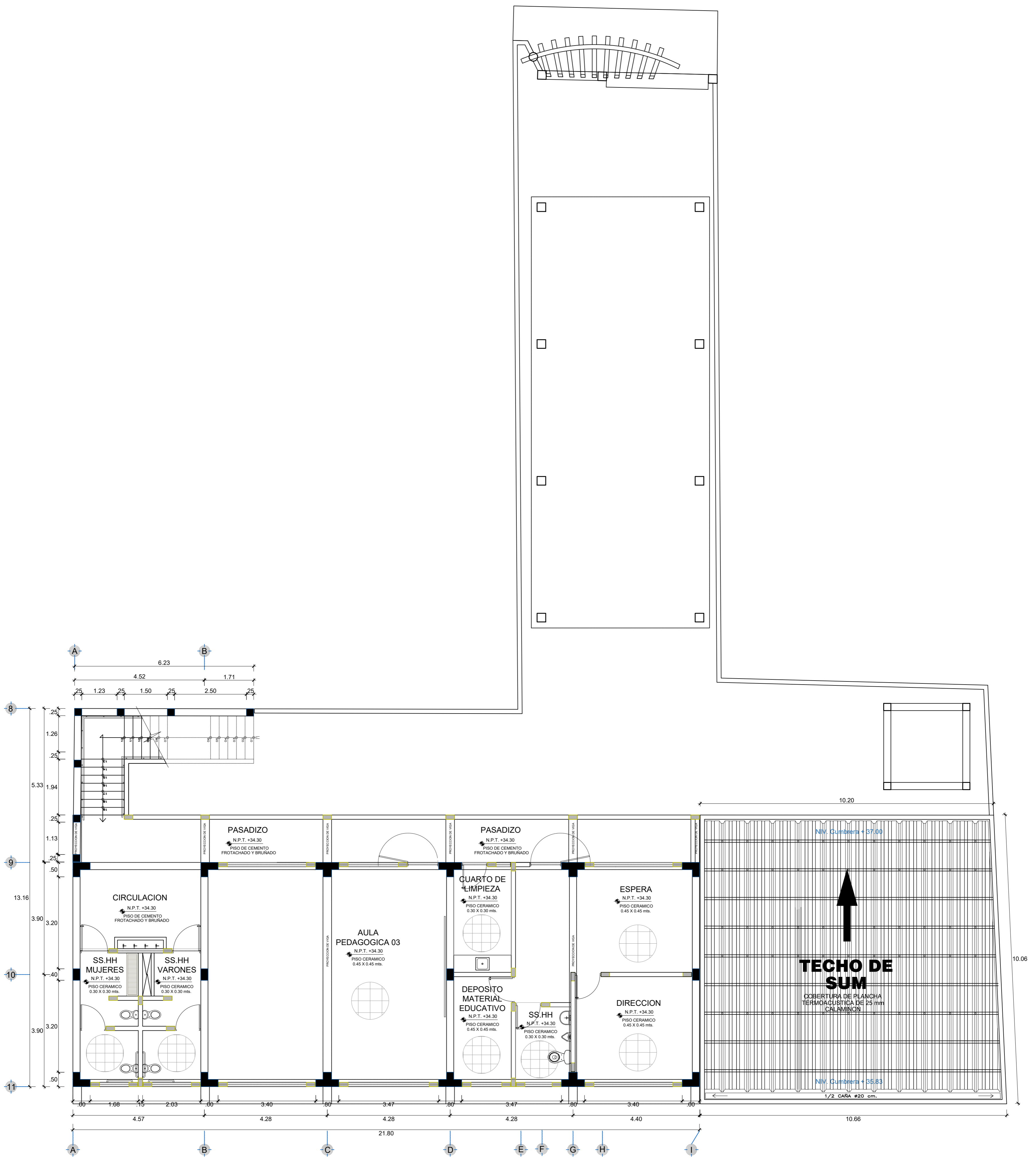
PLANTA SEGUNDO NIVEL - PISOS ESC: 1/75
