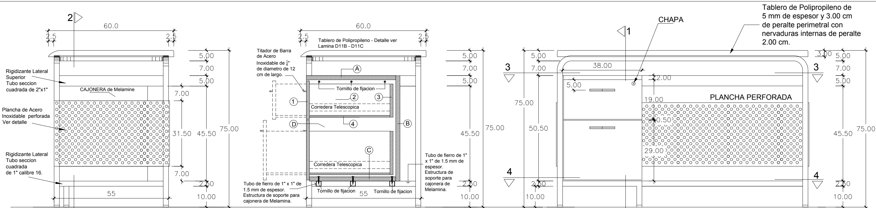
2 ELEVACION LATERAL 1 ELEVACION INTERNA
