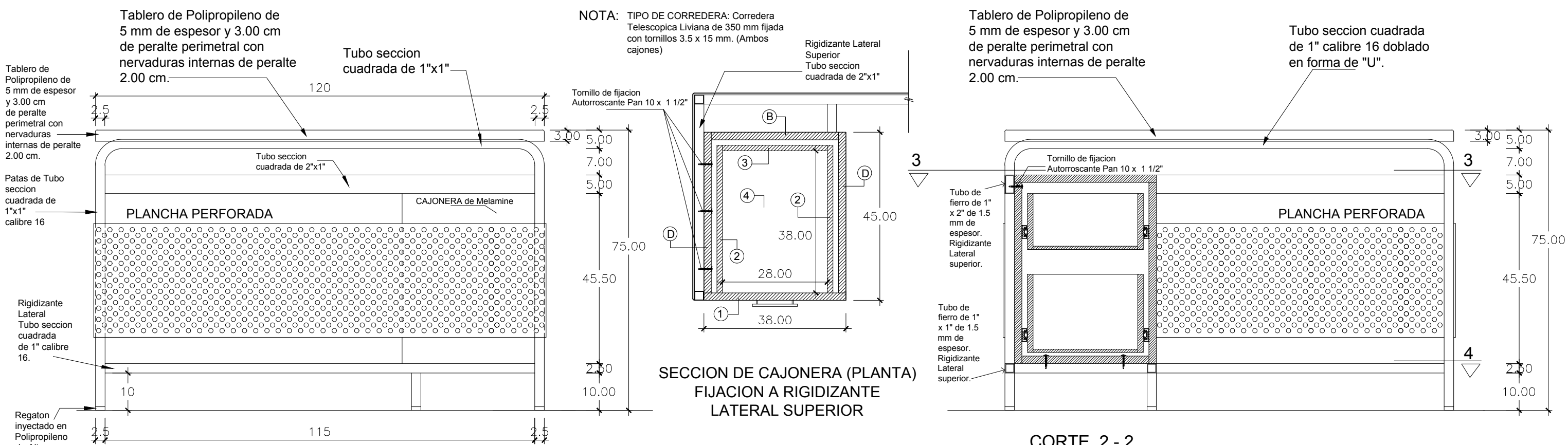
3 VISTA FRONTAL 2 SECCION DE CAJONERA (PLANTA) FIJACION A RIGIDIZANTE LATERAL SUPERIOR 4 CORTE 2-2
