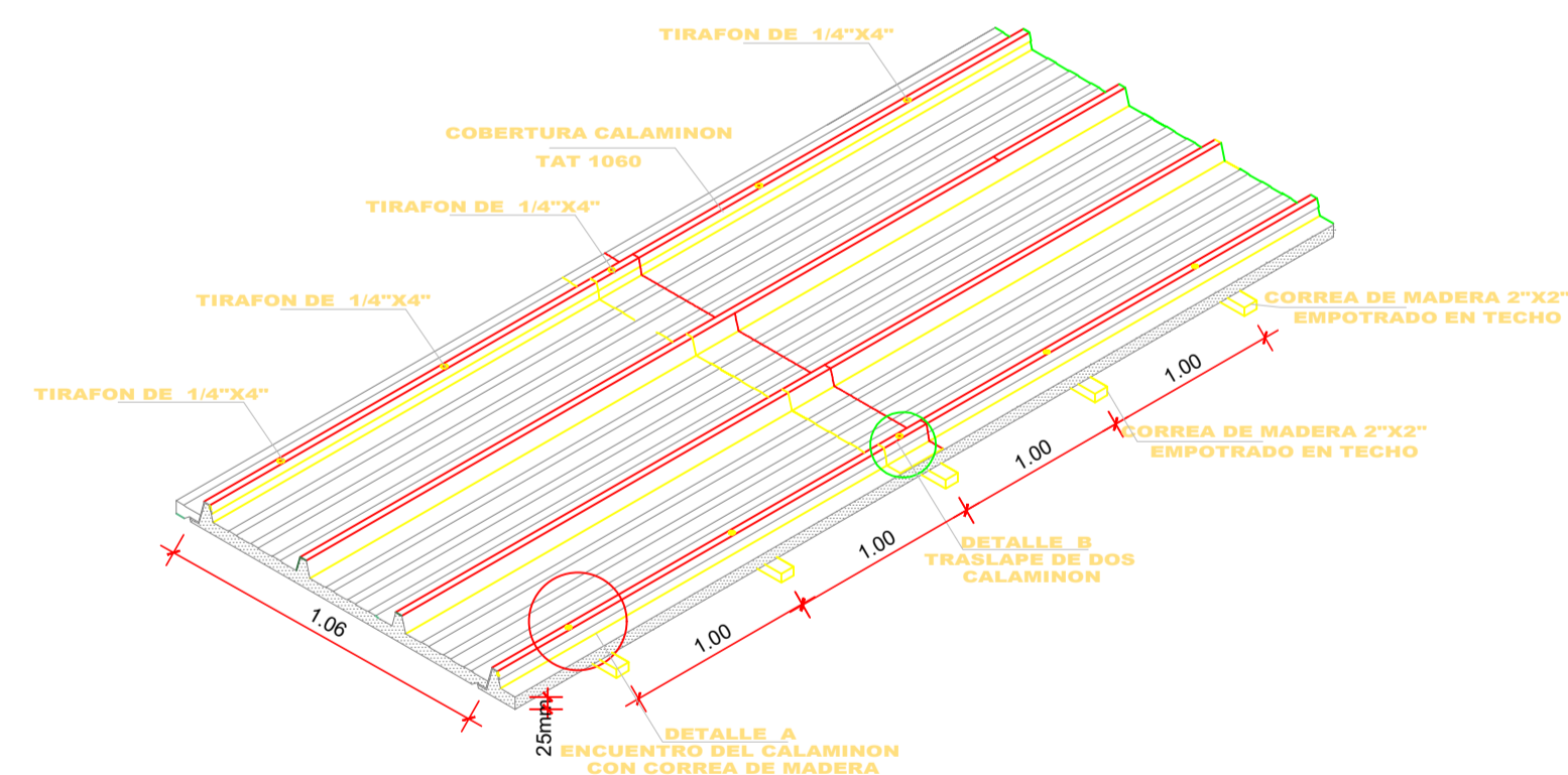
FIJ. EN PLANCHA CON CORREA
