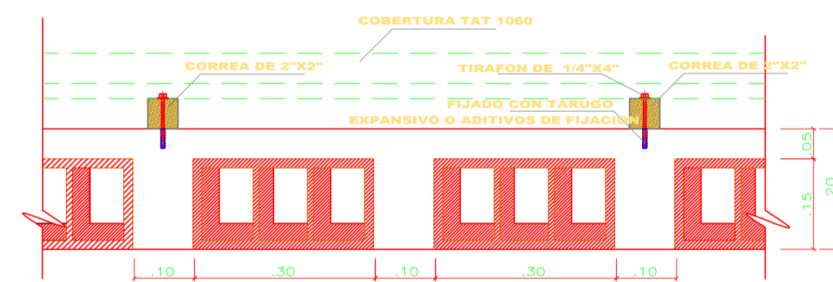
FIJADO DE CORREA A LOSA ALIGERADA
