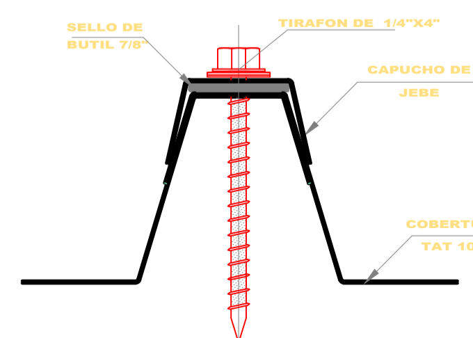
SELO BUTIL EN CAPUCHOS
