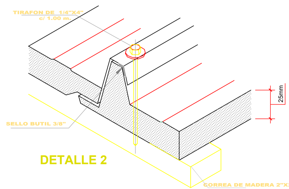
FIJ. EN PLANCHA CON CORREA
