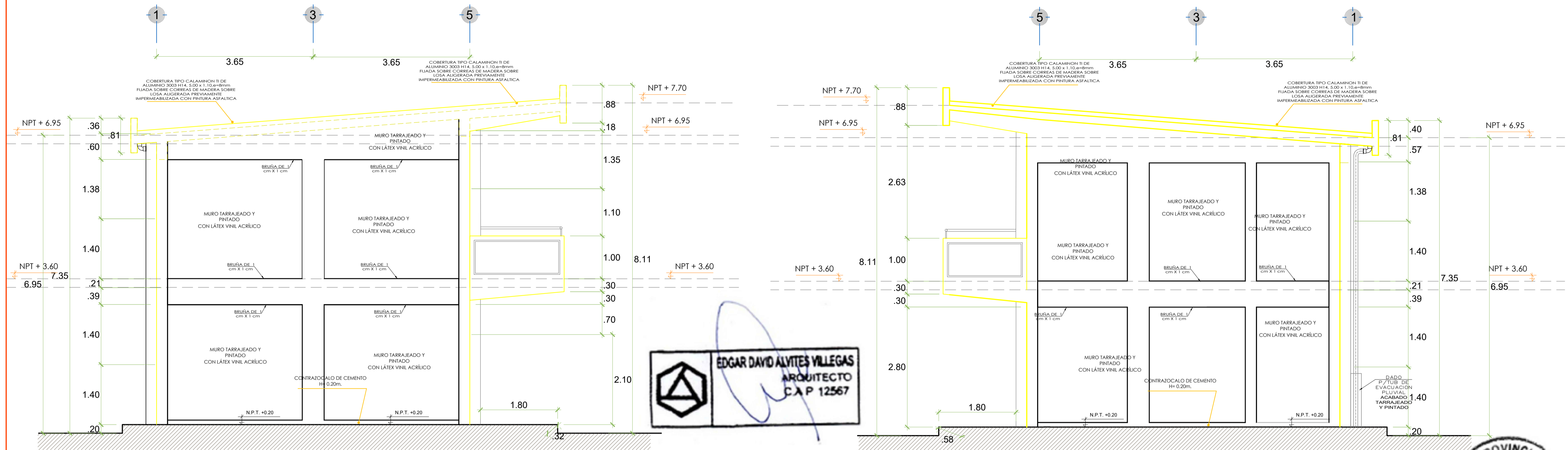
ELEVACION LATERAL IZQUIERDA ESC. 1/50
