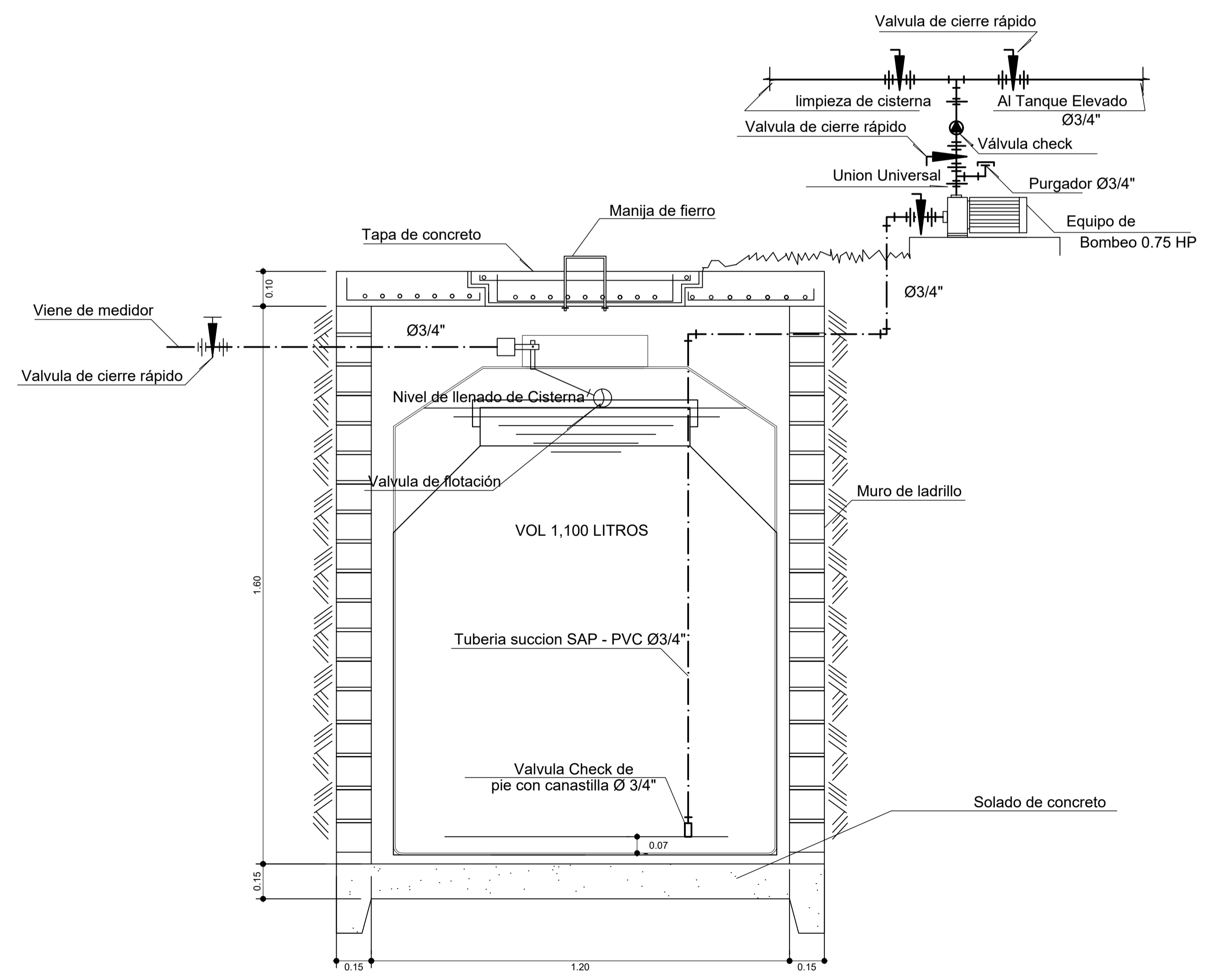
DETALLE DE CISTERNA ESC 1/20
