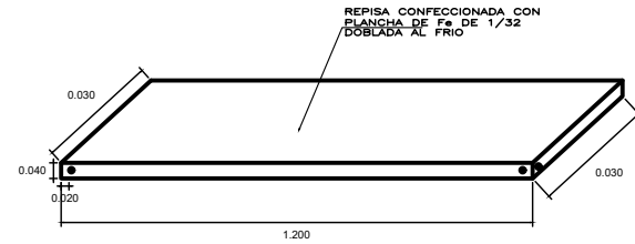
DETALLE DE BALDA ESC. 1/10
