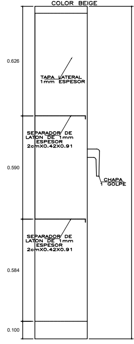
ELEVACION LATERAL ESC. 1/10
