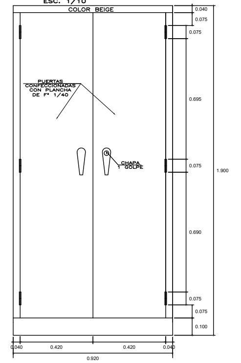
ELEVACION FRONTAL ESC. 1/10
