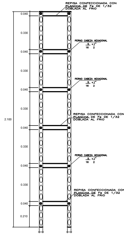
DETALLE DE BALDA ESC. 1/10
