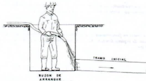
FIGURA Nº07: Limpieza de los tramos iniciales de los colectores.
