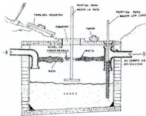
TANQUE SEPTICO
