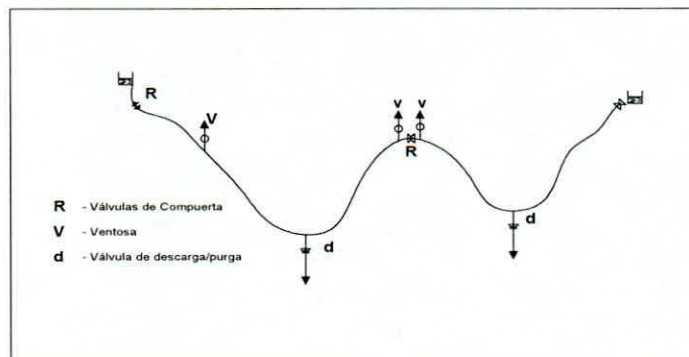
FIG. 1 - VALVULAS EN LINEAS
