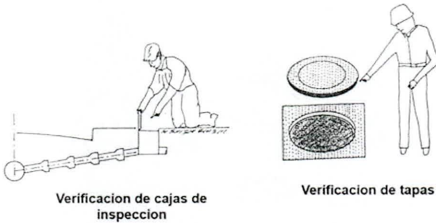
FIGURA N°03: Verificación de cajas de los registros domiciliarios y de las tapas.
