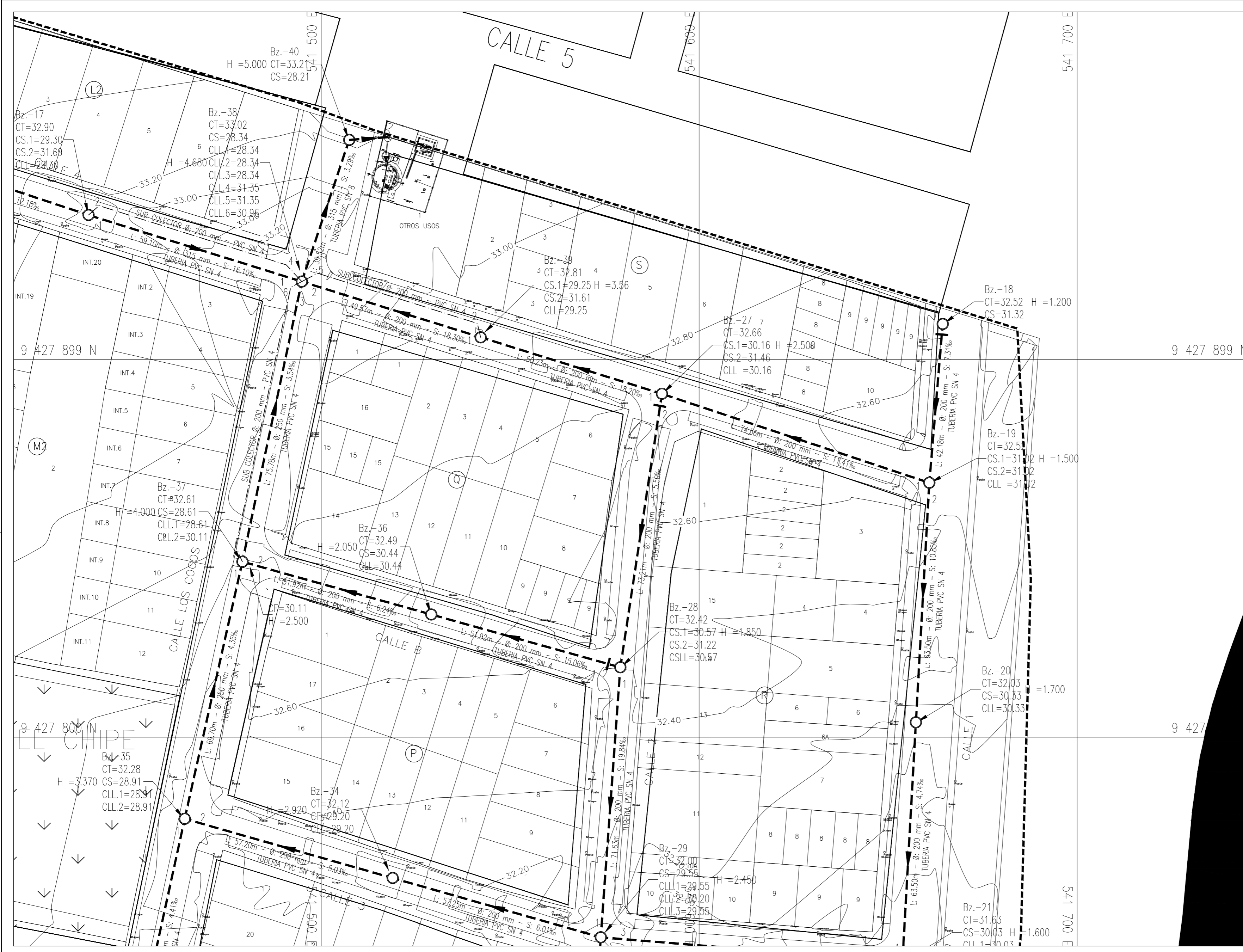
PLANO: ALCANTARILLADO PROYECTADO ESC.: 1/500
