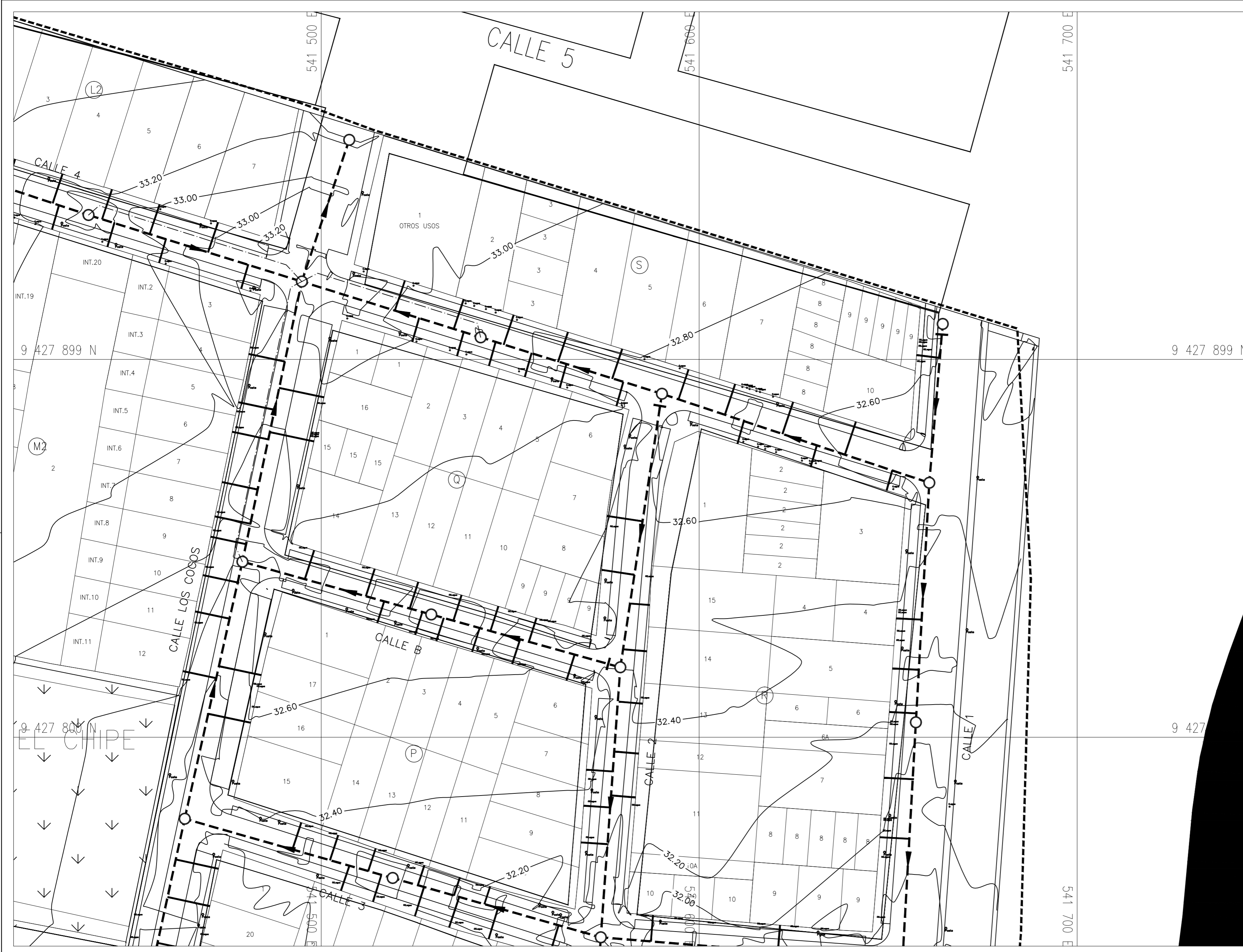
PLANO: CONEXIONES DOMICILIARIAS ALCANTARILLADO PROYECTADO ESC.: 1/500
