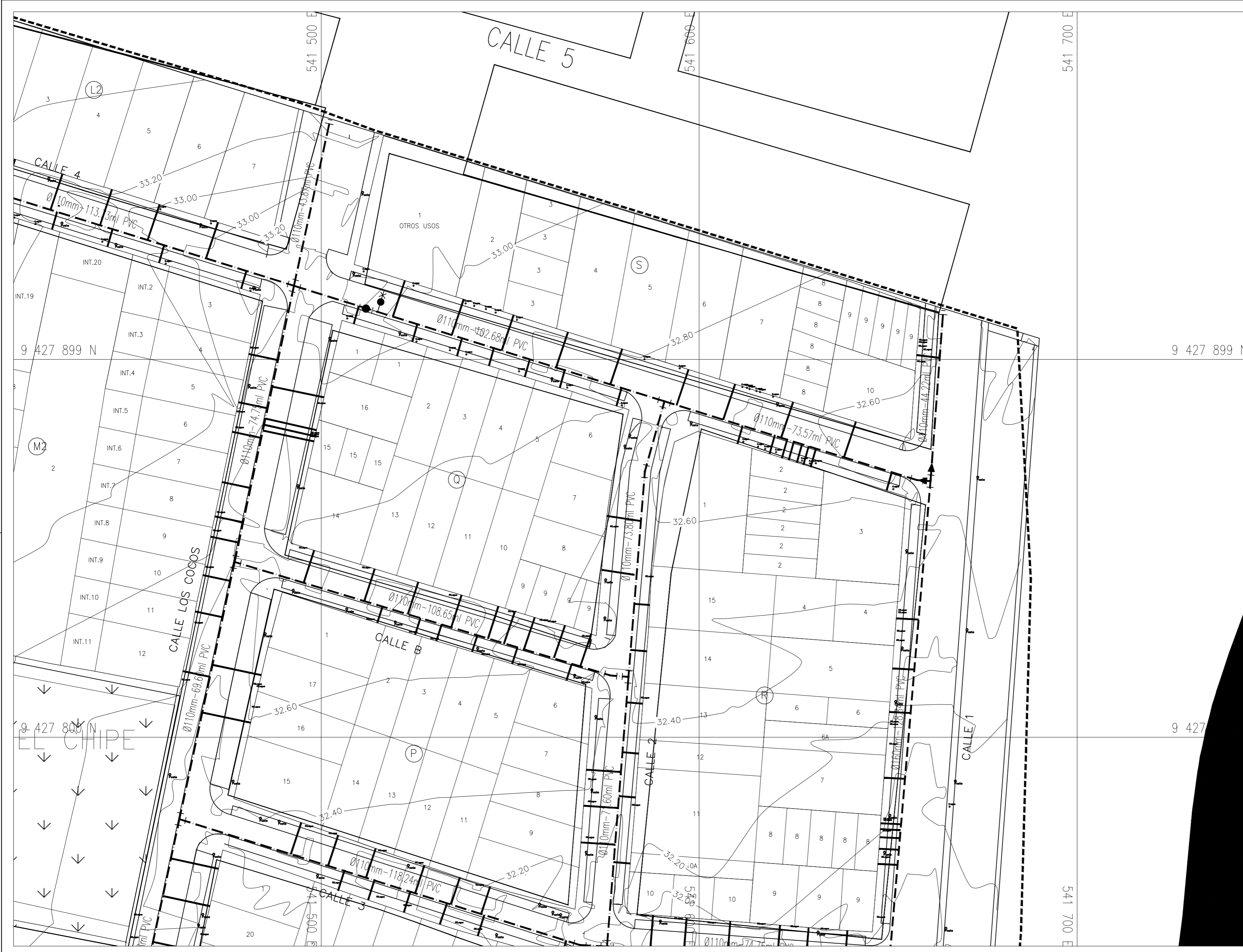
PLANO: CONEXIONES DOMICILIARIAS AGUA POTABLE PROYECTADO ESC.: 1/500
